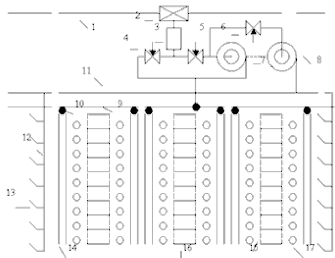
Рис. 1. Комбинированная система орошаемого земледелия фермерского хозяйства.
