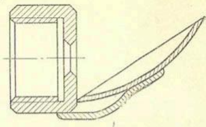
Рис. 27. Короткоструйная дождевальная насадка с ложкообразным дефлектором.
