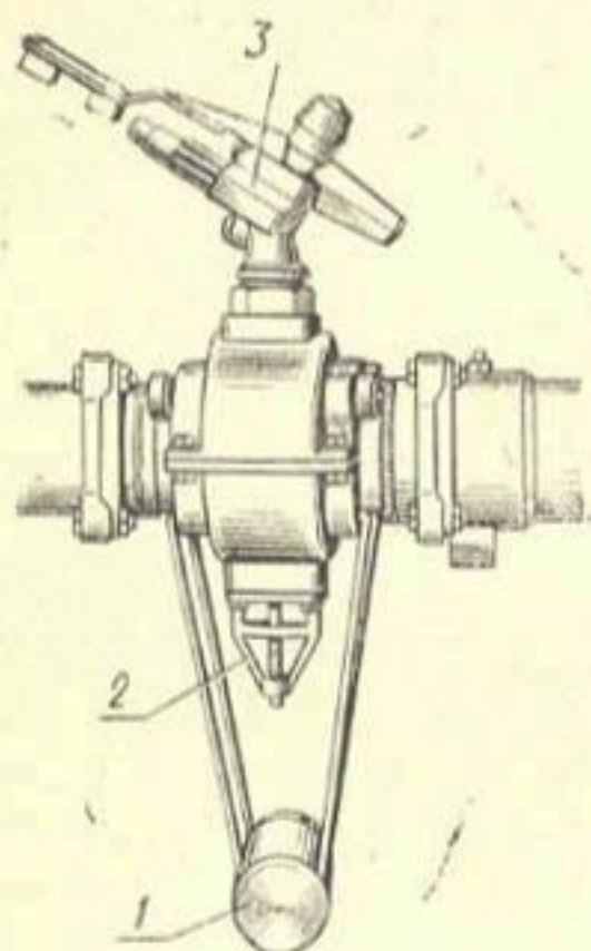
Рис. 104. Дождевальный аппарат:
