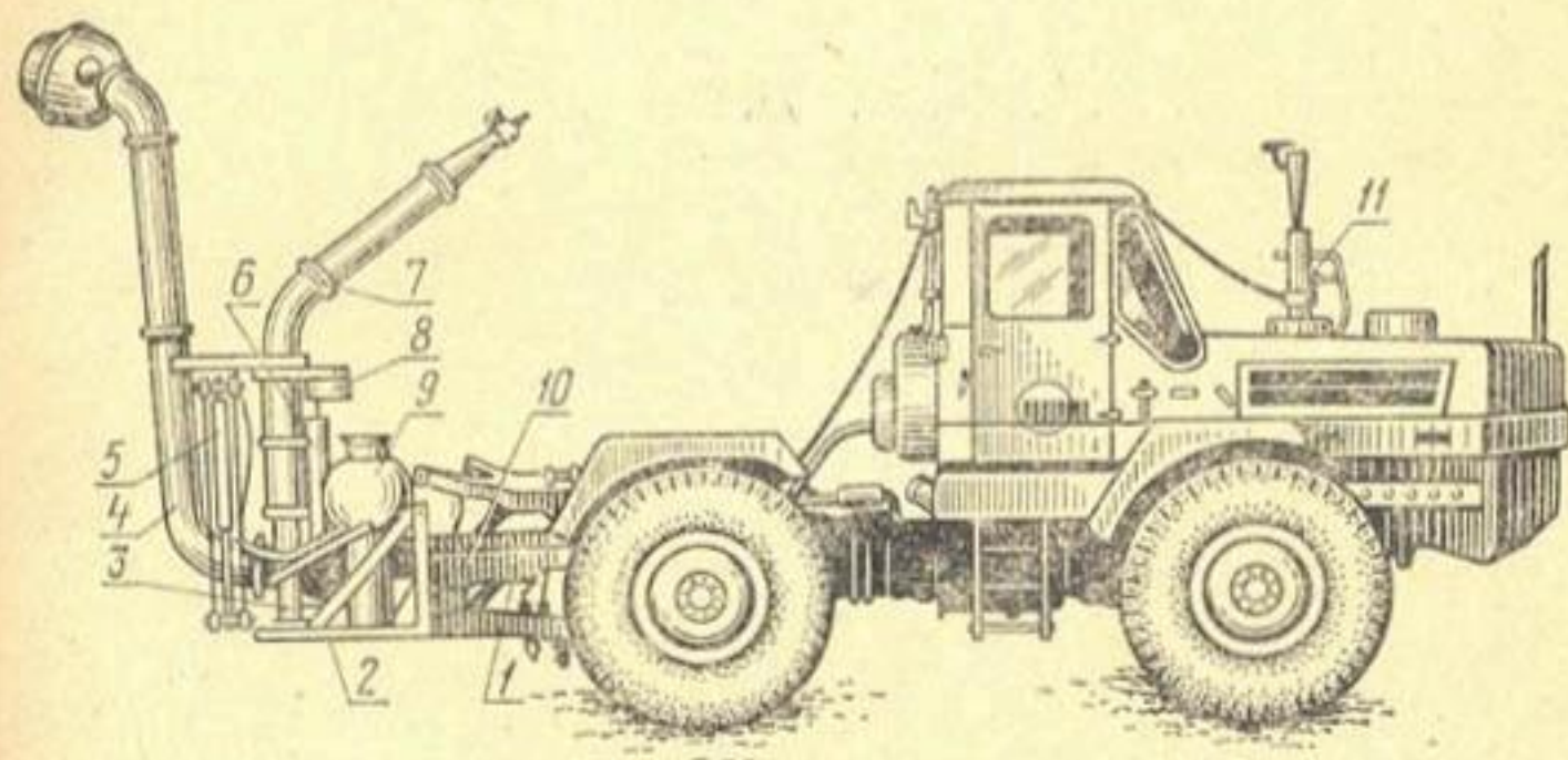
Рис. 71. Дальнейструйная дождевальная машина ДДН-100 навесная на трактор Т-150К:
