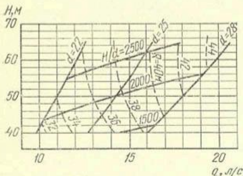
Рис. 41. Расходно-напорная характеристика дождевательного аппарата ДА-2 ( d в мм).
