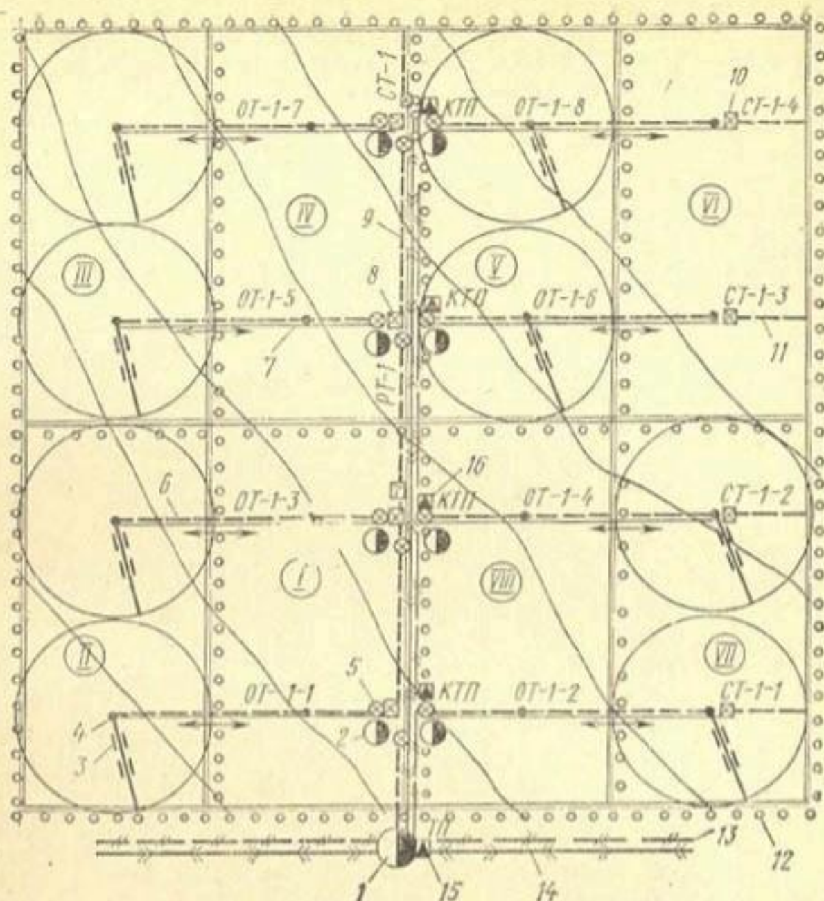
Рис. 92. Схема децентрализованной водоподачи на восьмипольном севооборотном участке при поливе дождевальными машинами «Фрегат»:
