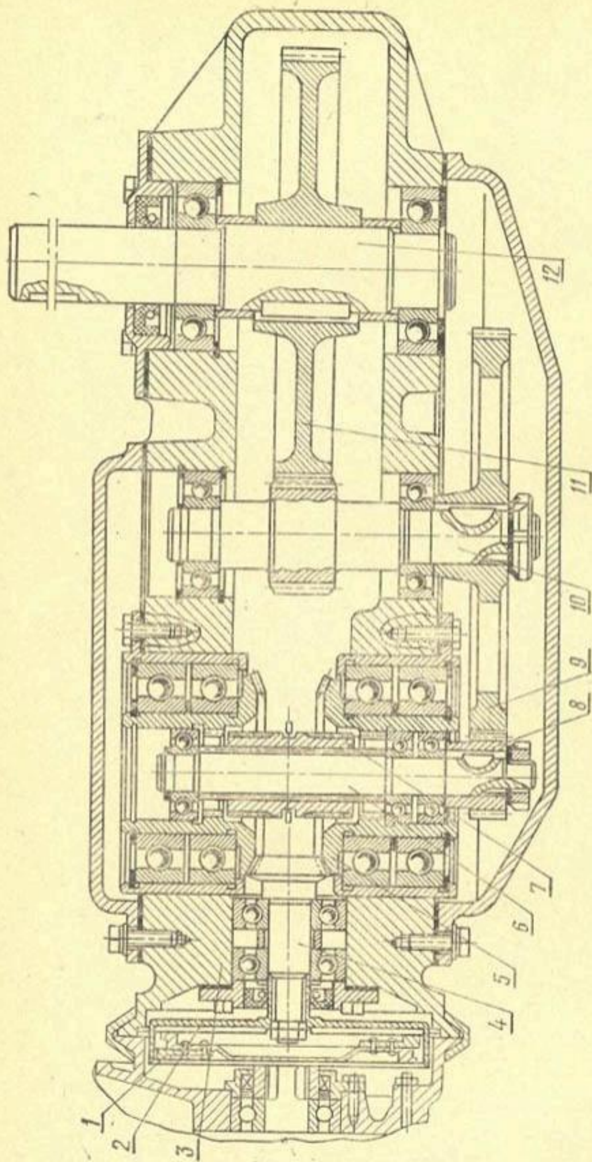
Рис. 78. Ревёрс-редуктор приводной тележки трубопровода «Волжанка»:
