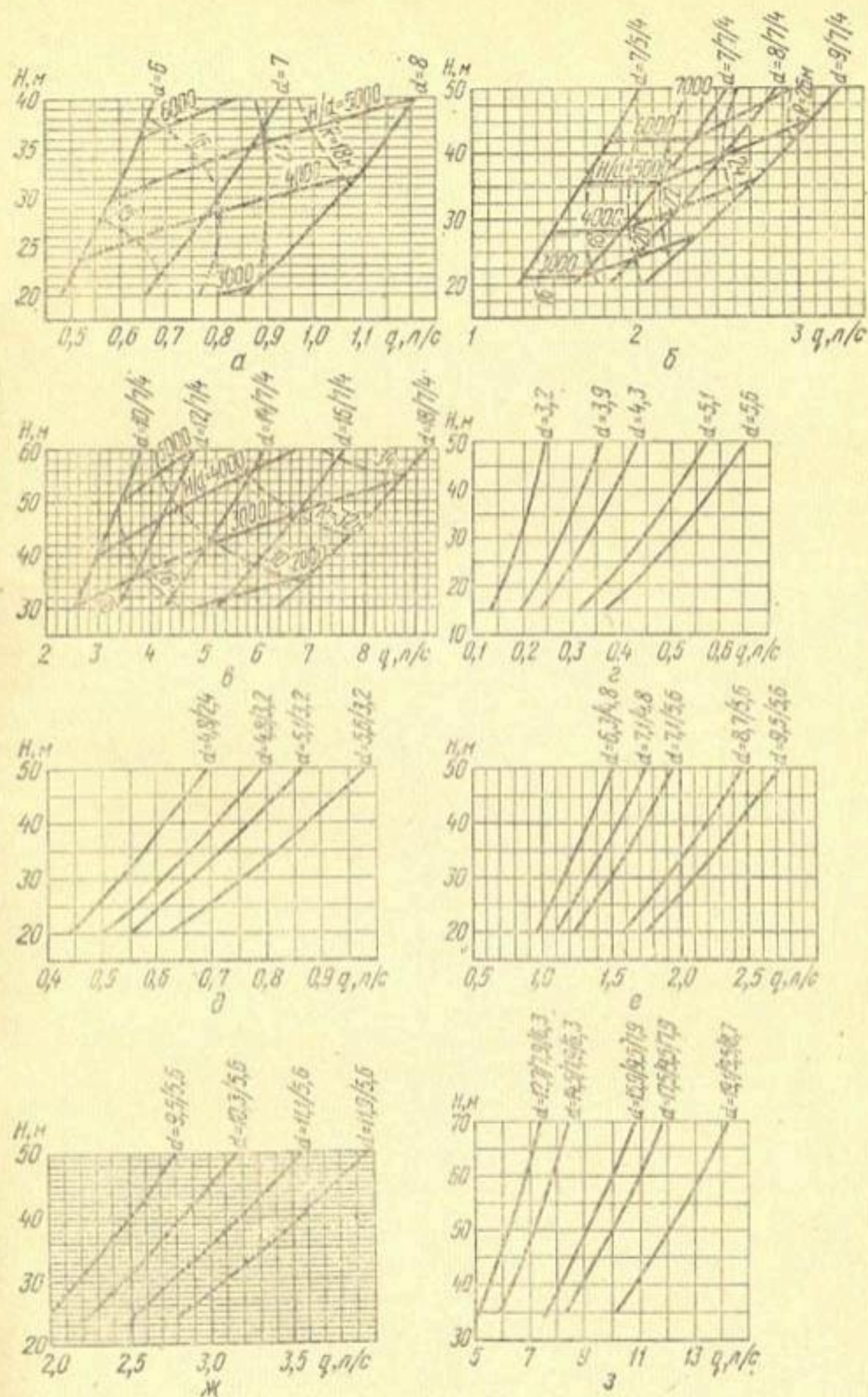
Рис. 38. Расходно-напорная характеристика дождевального аппарата: а — «Роса-1»; б — «Роса-2»; в — «Роса-3»; г — серии I ДМ «Фрегат»; д — се- рии II ДМ «Фрегат»; е — серии III ДМ «Фрегат»; ж — серии IV ДМ «Фре- гат»; з — концевое дождевальное аппарата ДМ «Фрегат» ( d в мм).
