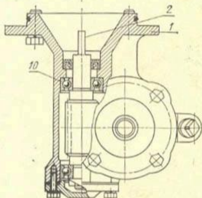
Рис. 68. Червячный редуктор дождевателя ДДН-70:
