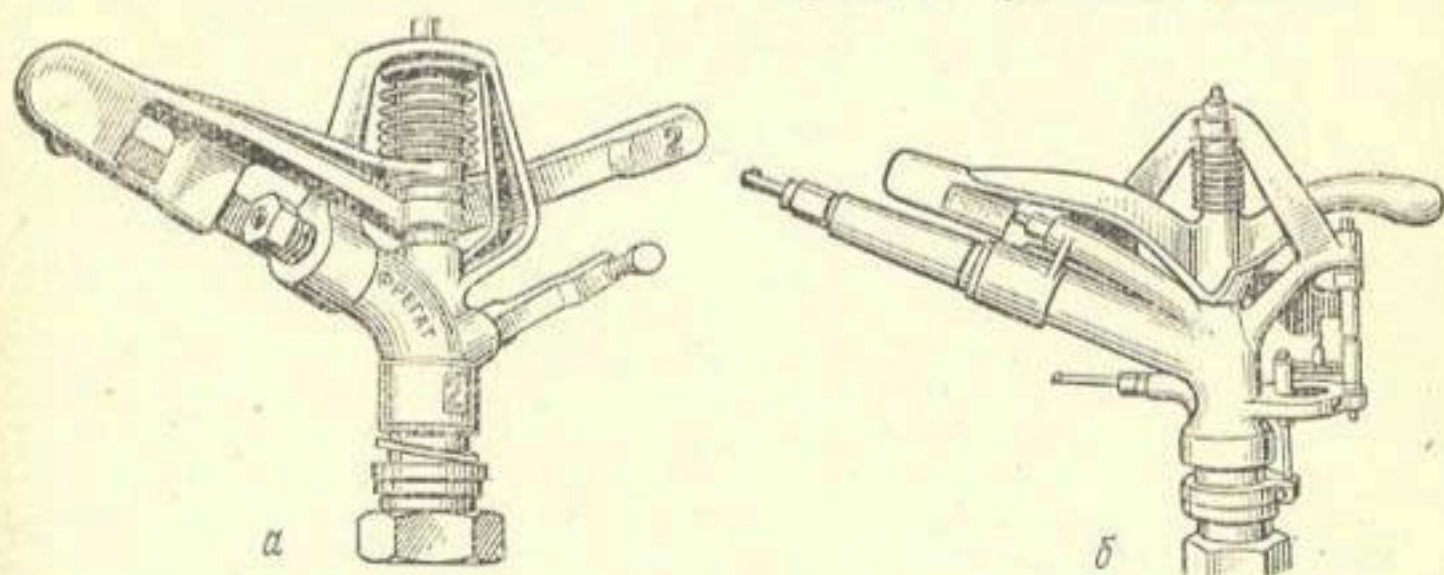
Рис. 35. Среднеструйный дождевальный аппарат серии II (а) и концевой дождевальный аппарат (б) ДМ «Фрегат».
