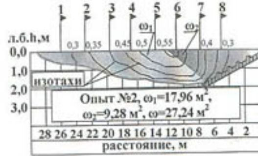
Рисунок 4 - Распределение продольных скоростей потока в изотахах (правая ветка канала Чиркейли).
