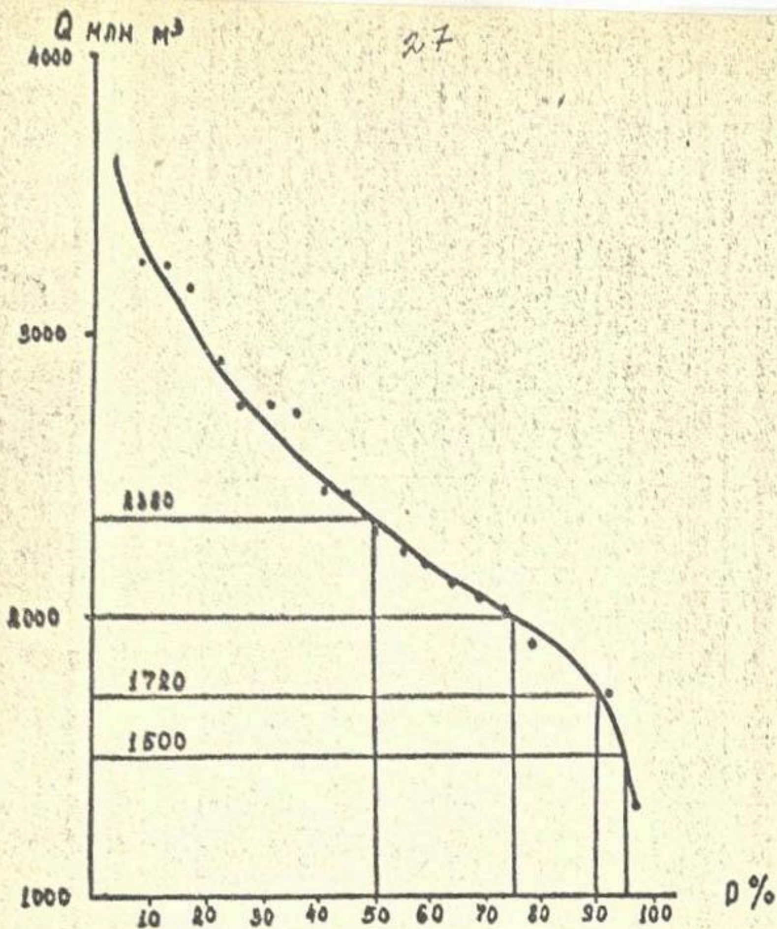
Рис. 1 Эмпирическая кривая обеспеченности годового стока КДС (млн.м 3 ) по Хорезмской области. за 1966 - 1986 г.
