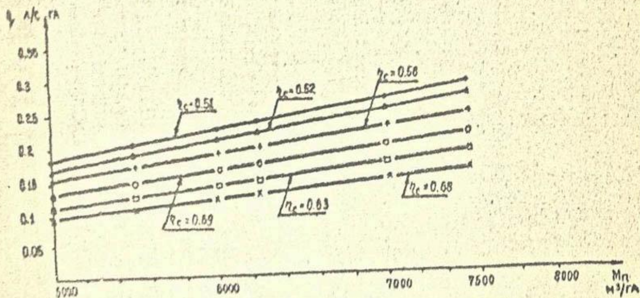
Рис. 7. Зависимость вегетационного дренажного модуля от обводнённости почвы при различных К.П.Д системы Нигиарынского района.
