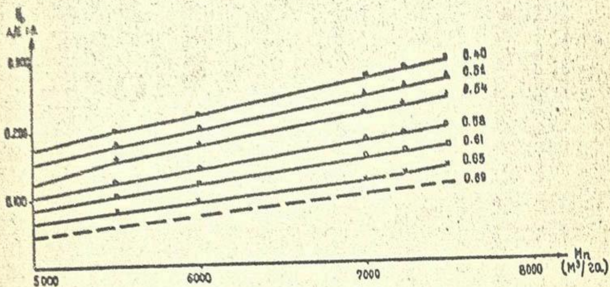
Рис. 2 Зависимость вегетационного дренажного модуля от оросительной нормы при различных К.П.Д системы по Богатскому району.
