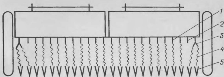
Рис. 13. Схема установки делителей потока на сеялке:
