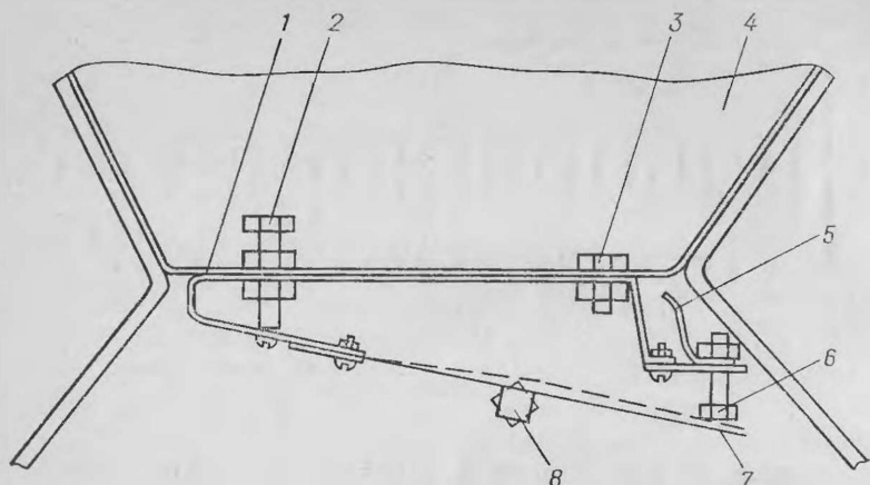
Рис. 14. Схема установки сигнализатора на сеялке:
