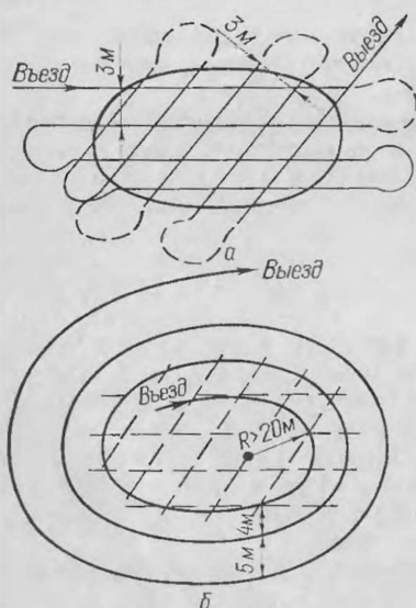
Рис. 12. Схема движения агре- гата при глубоком рыхлении местных понижений («блю- дец»):
