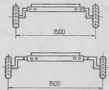
Рис. 21. Установка колеи опрыскивателя ОПШ-15-01.
