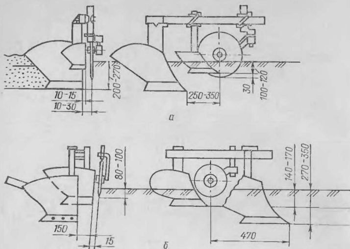
Рис. 5. Установка дискового ножа и предплужника на плуге: а — общего назначения; б — для ярсной вспашки.
