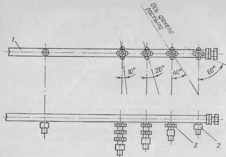
Рис. 24. Схема расположения распылителей на дополнительной секции в опрыскивателе ОПШ-15-01:
