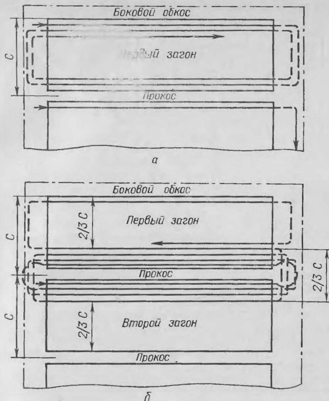
Рис. 31. Схема движения агрегата загонным способом: а — с правыми поворотами; б — с расширением прокоса.
