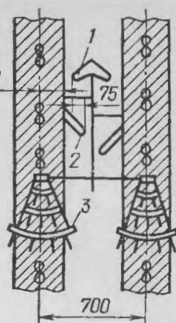
Рис. 34. Расстановка рабочих органов культиватора на междурядной обработке:
