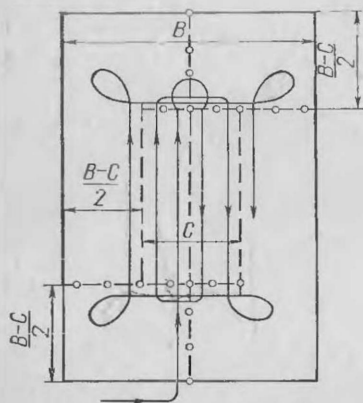
Рис. 6. Разметка поля и схема движения пахотного агрегата беззагонно-круговым способом от центра поля к периферии.
