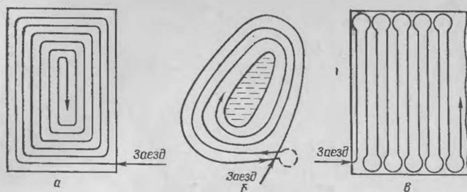
Рис. 29. Способы движения уборочных агрегатов:
