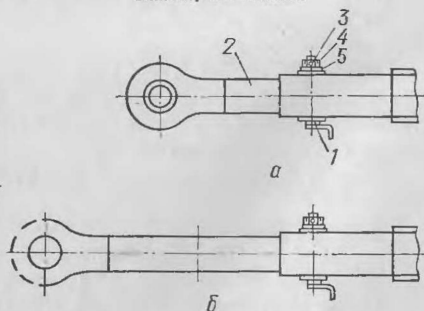
Рис. 19. Регулировка прицепной серьги опрыскивателя ОП-2000-2-01:
