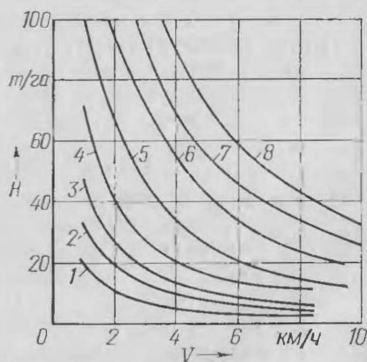
Рис. 32. Зависимость дозы внесения жидких органических удобрений (Н) от скорости движения агрегата (V) при ширине захвата 7 м и диаметре отверстий жиклеров:
