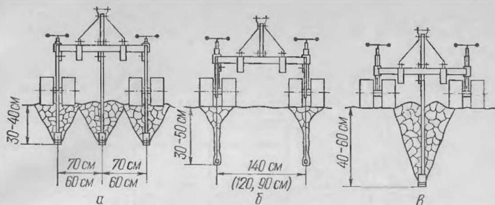
Рис. 10. Схема расположения рабочих органов при щелевании:
