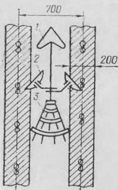
Рис. 35. Расстановка рабочих органов культиватора при междурядных обработках с присыпанием сорняков слоем почвы:
