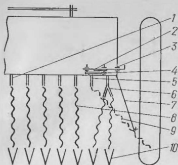
Рис. 17. Схема установки на сеялку приспособления для контроля нормы высева:
