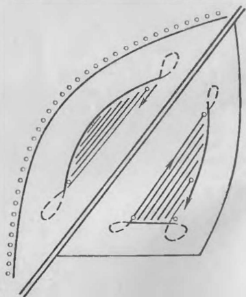
Рис. 7. Схема движения пахотного агрегата на полях с разной конфигурацией.
