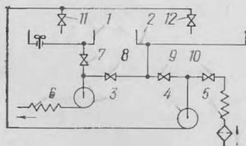
Рис. 27. Технологическая схема Ма Пемикс-1002:
