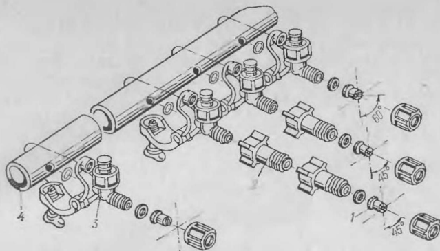
Рис. 25. Схема установки крайних распылителей на коллекторе опрыскивателя ОП-2000-2-01:
