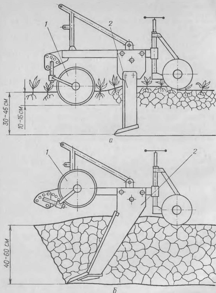
Рис. 9. Технологическая схема работы щелевателя:
