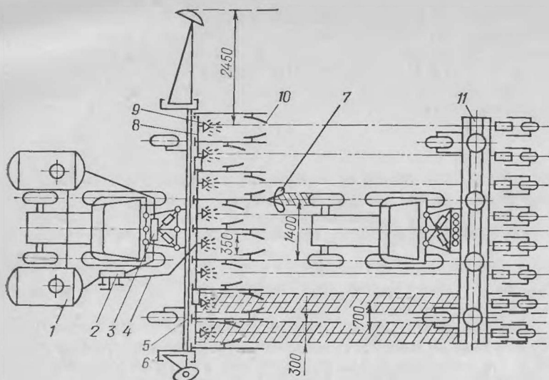
Рис. 33. Схема дооборудования и работы агрегатов на посеве кукурузы с полосным внесением гербицидов:
