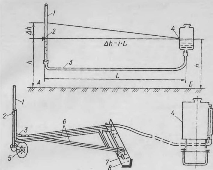
Рис. 11. Схема работы и конструктивные элементы устройства «Горизонталь» для вождения почвообрабатывающих агрегатов по горизонталям склонов:
