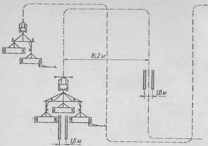
Рис. 16. Схема движения посевных агрегатов при разметке технологических колеи через 16,2 м.
