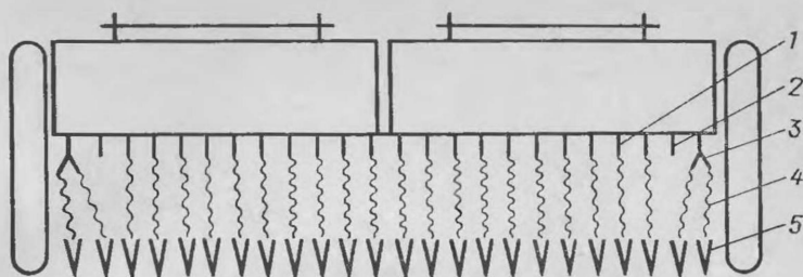
Рис. 13. Схема установки делителей потока на сеялке:
