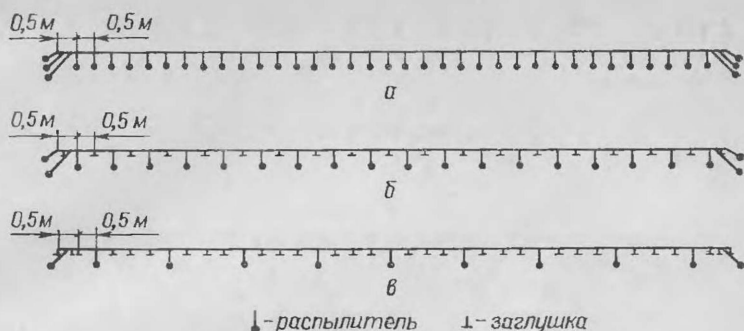
Рис. 22. Схема расстановки распылителей на коллекторе опрыскивателя ОП-2000-2-01:
