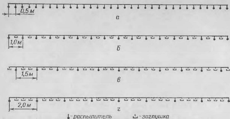
Рис. 23. Схема расстановки дефлекторных распылителей на коллекторе штанги опрыскивателя ПОМ-630:
