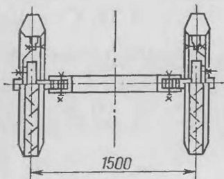
Рис. 18. Установка колес опрыскивателя ОП-2000-2-01.
