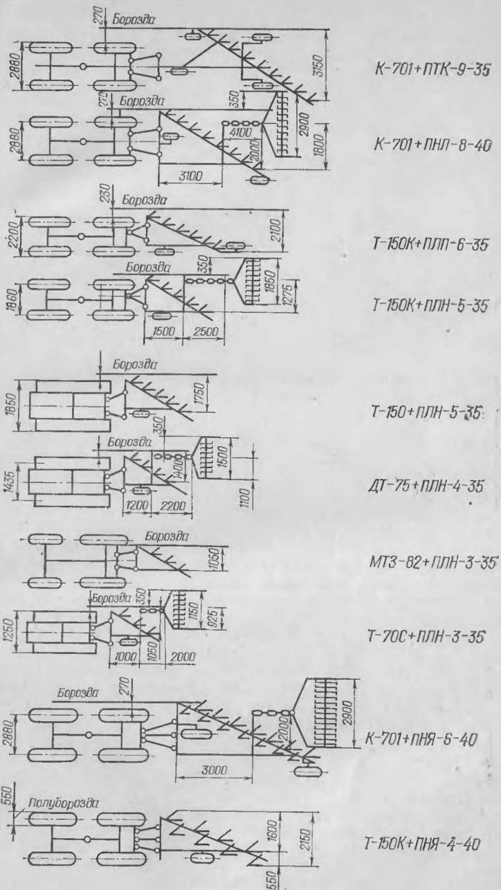
Рис. 4. Состав пахотных агрегатов.
