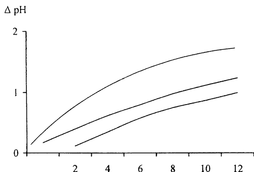
Рис. 1 Влияние доз извести ( \text{CaCO}_3 , т/га) на сдвиг рН дерново-подзолистых почв
