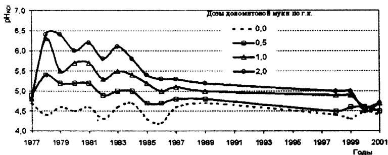
Рис. 8 Динамика pH_{KCL} почвы при внесении N_{90}P_{90}K_{120} на фоне различных доз доломитовой муки
