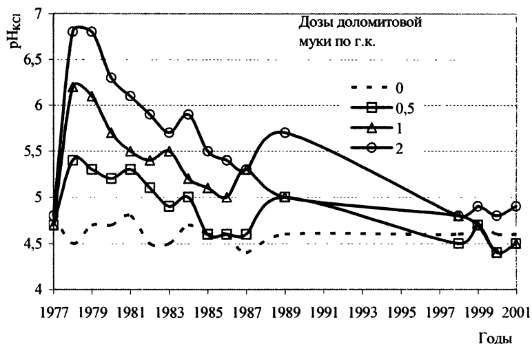
Рис. 19 Динамика pH_{KCl} почвы при внесении 80 т/га навоза + N_{90}P_{90}K_{120} на фоне различных доз мелиоранта
