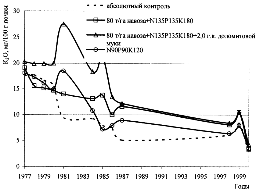
Рис.23 Динамика содержания обменного калия в почве
