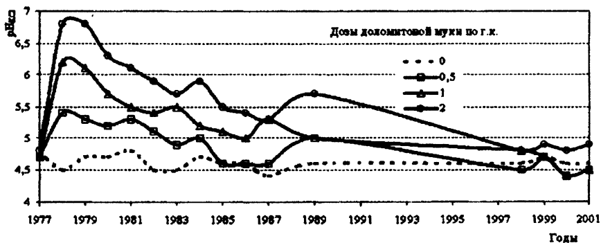
Рис. 7 Динамика pH_{KCL} почвы при внесении 80т/га навоза + N_{90}P_{90}K_{120} на фоне различных доз мелиоранта
