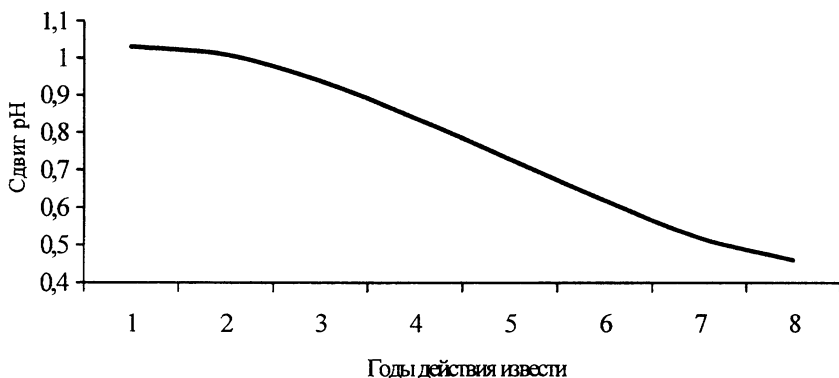
Рис. 2 Изменение сдвига величины pH известкованных почв во времени
