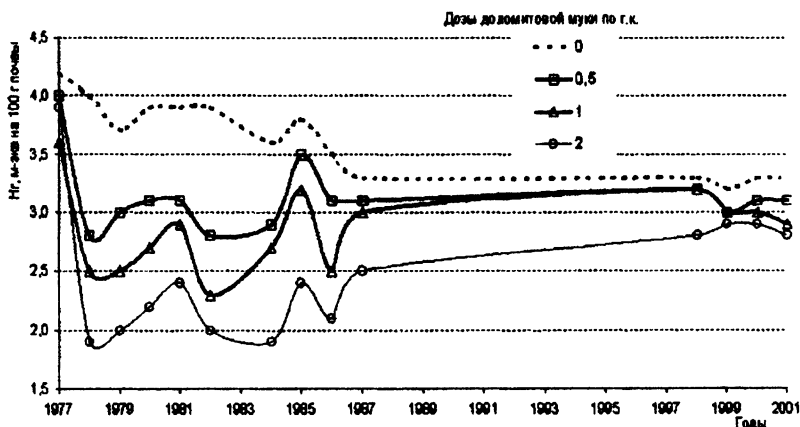
Рис. 9 Динамика гидролитической кислотности почвы при внесении 80 т/га навоза + N_{135}P_{135}K_{180} на фоне различных доз мелиоранта
