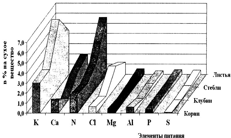
Рис. 29 Распределение элементов питания по органам растений картофеля
