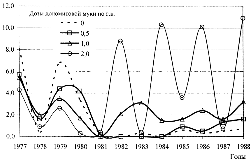
Рис. 28 Распространение парши обыкновенной (сильная степень) при внесении N_{135}P_{135}K_{180} на различных фонах известкования
