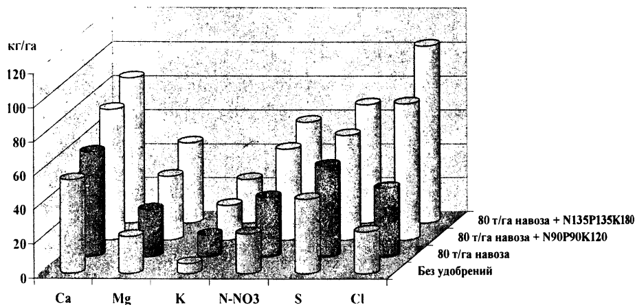
Рис. 31 Потери элементов питания с инфильтрационными водами из пахотного слоя дерново-подзолистой супесчаной почвы (1977-1984 гг.), кг/га
