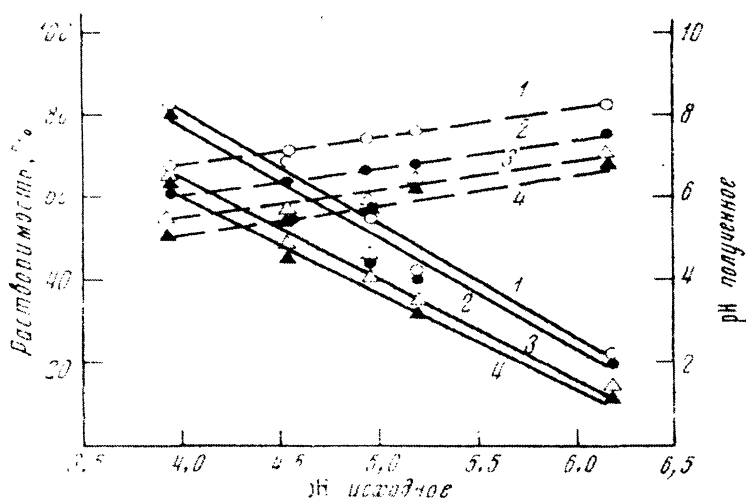
Рис. 17 Растворимость CaO и MgO минералов в буферных растворах и влияние их на изменение pH этих растворов
