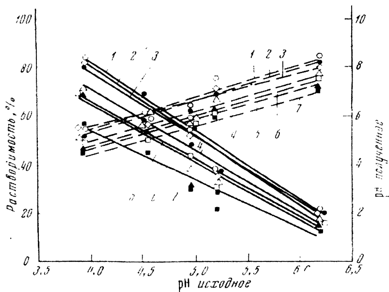
Рис. 16 Растворимость CaO и MgO шлаков в буферных растворах и влияние их на изменение pH этих растворов
