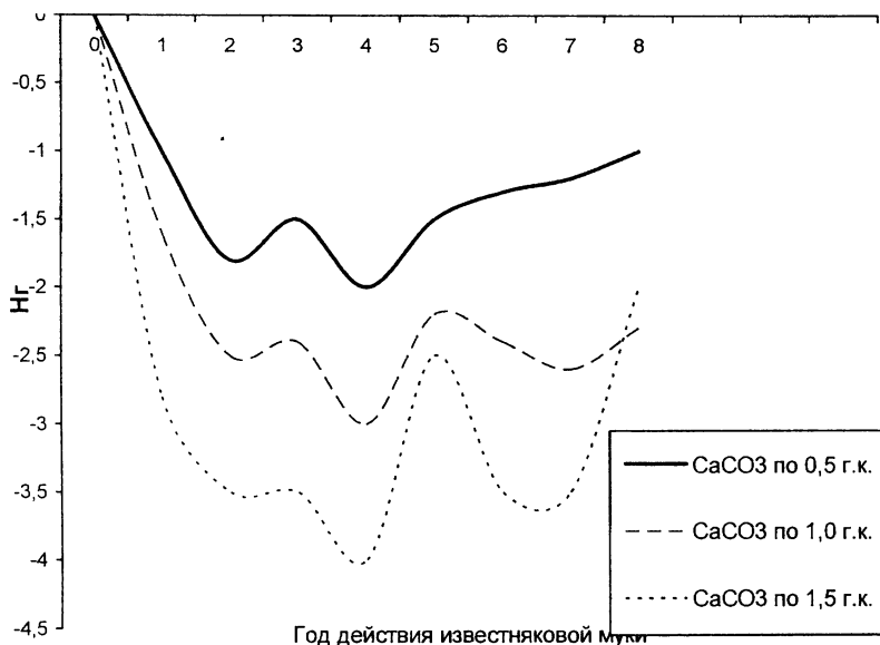
Рис. 12 Изменение Нг во времени в произвесткованном выщелоченном тяжелосуглинистом черноземе
