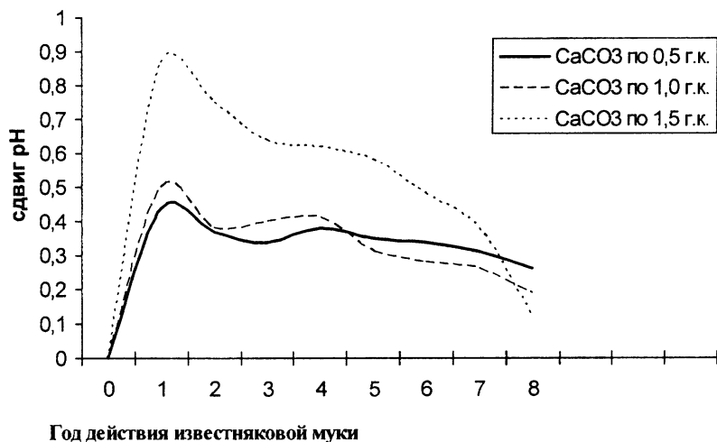
Рис. 11 Изменение pH во времени в произвесткованном выщелоченном тяжелосуглинистом черноземе
