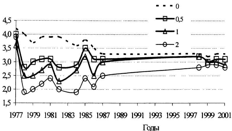
Рис. 21 Динамика гидролитической кислотности почвы при внесении 80 т/га навоза + N_{135}P_{135}K_{180} на известкованных фонах
