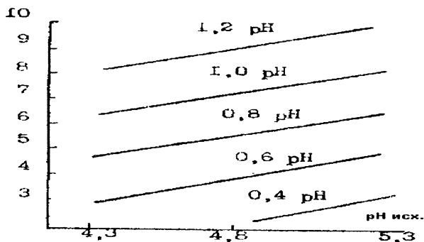
Рис. 13 Серые лесные почвы
