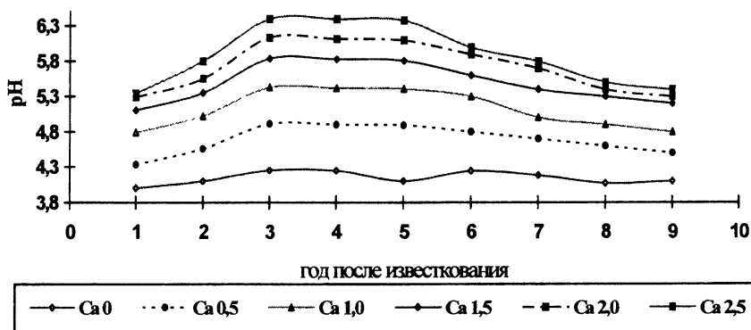
Рис. 5 Изменение реакции почвенной среды после известкования
