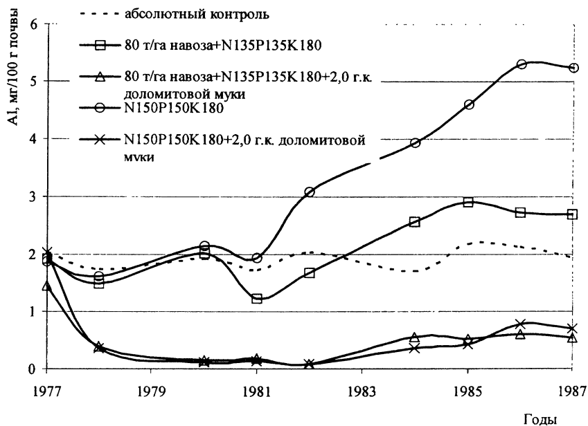
Рис.22 Динамика содержания подвижного алюминия в почве
