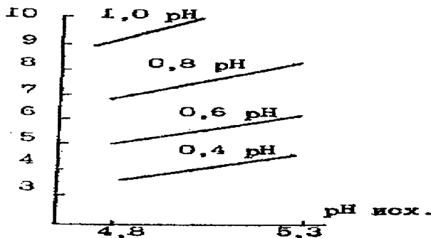
Рис. 15. Чернозёмы выщелоченные и оподзоленные
