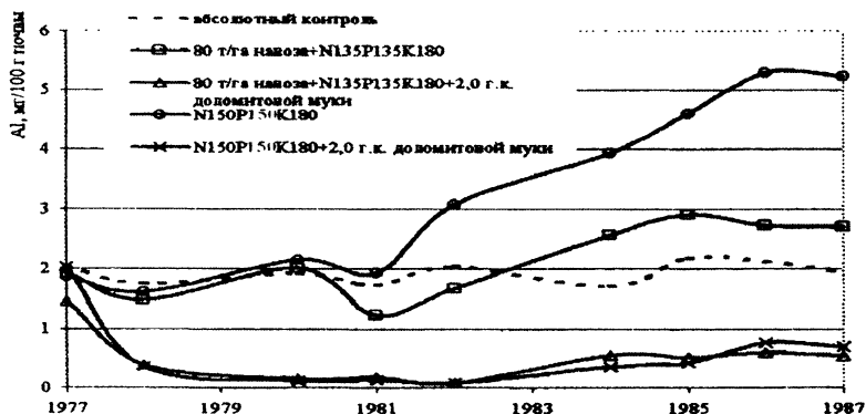
Рис. 10 Динамика содержания подвижного алюминия в почве
