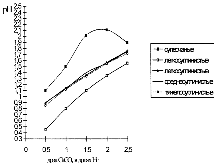
Рис. 6 Влияние дозы извести на сдвиг pH почв разного гранулометрического состава
