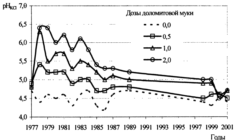
Рис. 20 Динамика pH_{KCl} почвы при внесении N_{90}P_{90}K_{120} на фоне различных доз доломитовой муки
