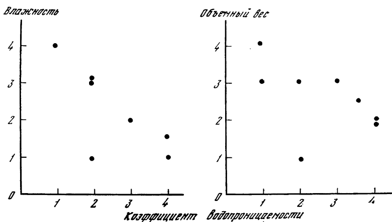
Рис. 1. Зависимость коэффициента водопроницаемости от влажности и объемного веса дерново-подзолистой почвы
