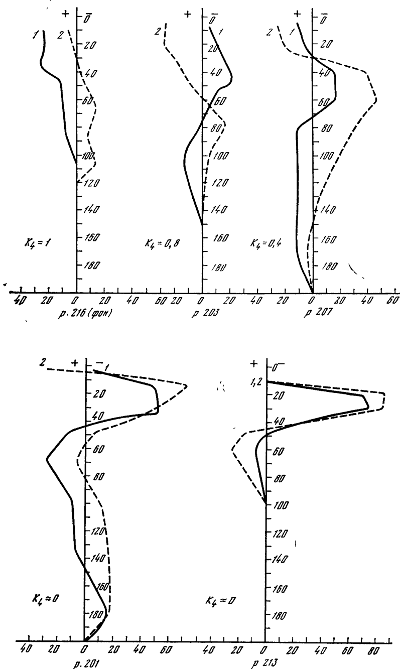
Рис. 4. Кривые выноса — накопления ила и суммы обменных \text{Ca}+\text{Mg} по отношению к породе
