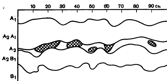
Рис. 2. Фрагменты второго гумусового горизонта на фоне подзолистого гор. A_2 , вскрытые траншеями на лесном участке
