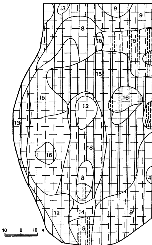
Рис. 1. Почвенный покров холма моренного рельефа Жемайтской возвышенности
