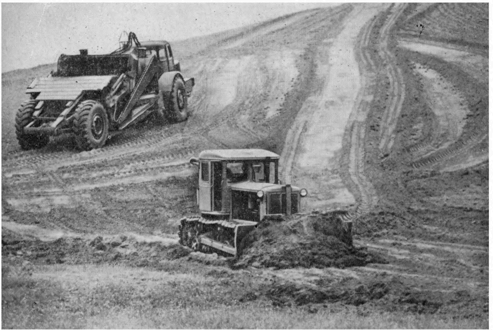
Рис. 1. Выполаживание склона автоскрепером и засыпка заболоченной впадины бульдозером (фото Я. Талберга)
