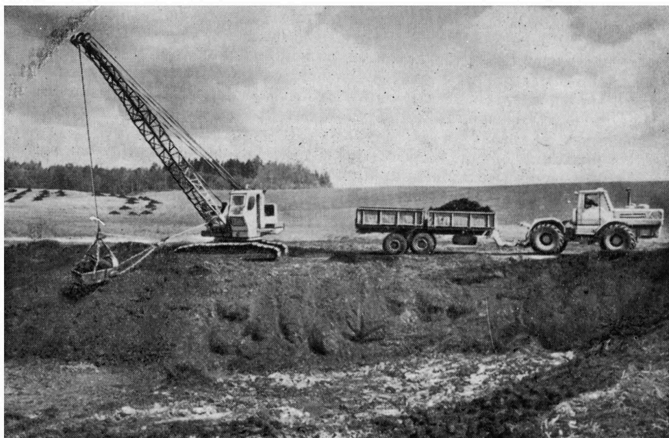
Рис. 4. Добыча торфа для рекультивации в предварительно осушенном котловане стокорегулирующего пруда-копая (фото Я. Талберга)
