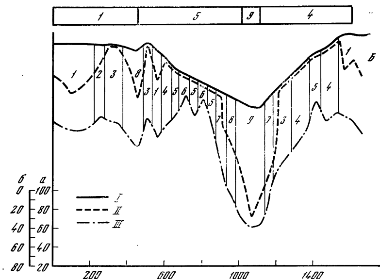
Рис. 1. Почвенно-геоморфологический профиль
