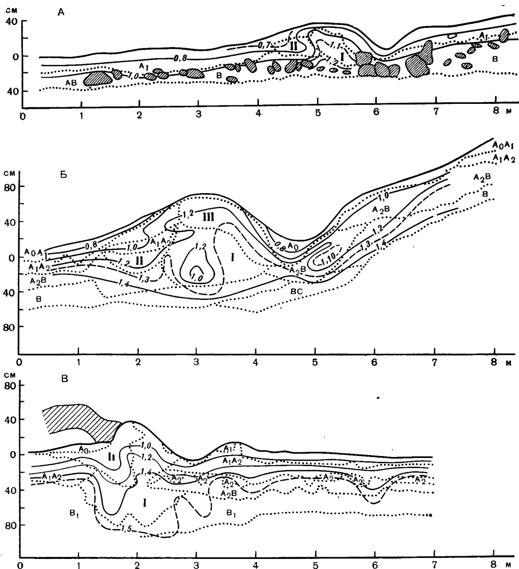
Рис. 2. Распределение ОВ в вывалах
