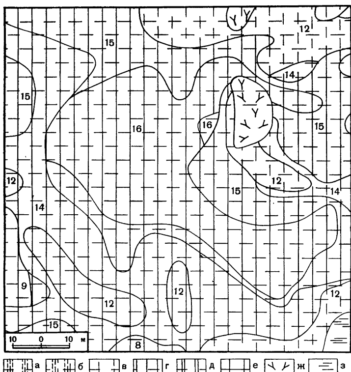
Рис. 1. Почвенный покров холма моренного рельефа Жемайтской возвышенности
