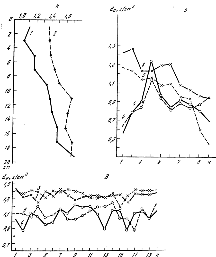
Рис. 1. Изменение ОВ дерново-подзолистой почвы при рекреационном воздействии А — мощность уплотненного слоя: 1 — контроль, 2 — тропа; Б — ОВ по радиусу парцеллы в березняке; В — ОВ в пределах парцеллы в ельнике: глубина 0—4 см; 3 — тропа, 4 — контроль; глубина 0—2 см: 5 — тропа, 6 — контроль
