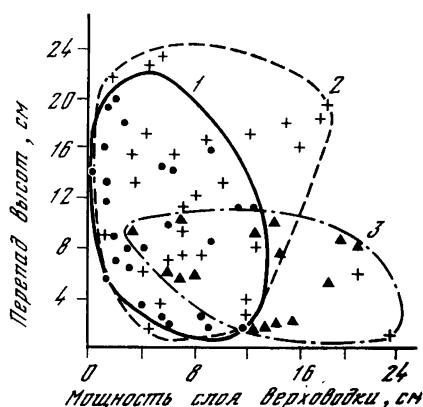
Рис. 6. Связь почв основных ЭПА участка с условиями микрорельефа и внутреннего стока верховодки
