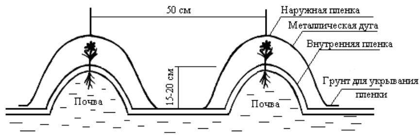
Рис. 7. Схема строения пленчатого укрытия (термостата) для выращивания томатов
