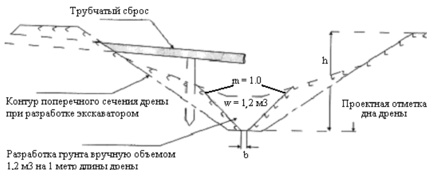
Рис. 2. Поперечное сечение дрена. М – 1:50 (разработка грунта вручную)
