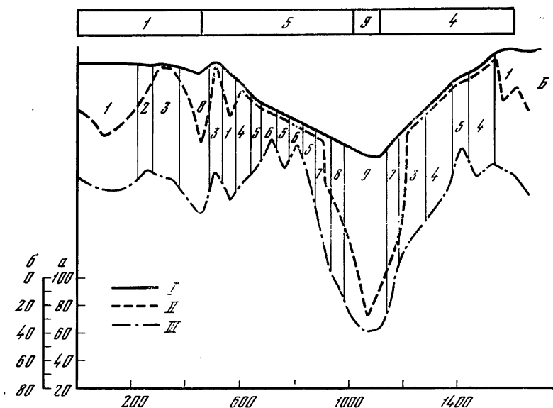
Рис. 1. Почвенно-геоморфологический профиль
