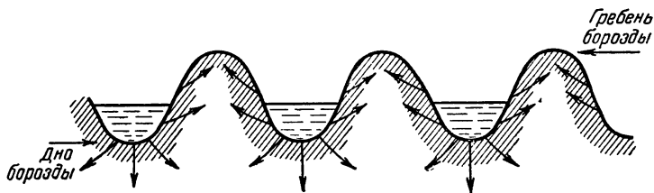
Рис. 25. Схема движения и накопления солей на гребнях борозд при поливе (по В. А. Ковда, 1946).
