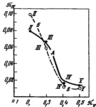
Рис. 25. Поэтапный характер связи между критериями почвенного подобия P_{гv} (показатель интенсивности изменения солепроявления в почве) и P_v (КЗИ)
