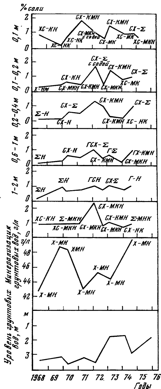
Рис. 8. Результаты много- летних (1968—1977 гг.) наблюдений на массиве Кегейли за динамикой за- солнения почв и зоны аэра- ции (гидрохимкуст 16, см рис. 3), а также за глубин- ной, минерализацией и химическим составом грунтовых вод
