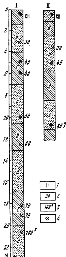
Рис. 20. Термолюминесценция разновозрастных почв и суглинков лёссов Чарвакской котловины I — геологическая канава, II — шурф 39. 1 — свечение образцов отсутствовало; 2 — свечение мелкозема; 3 — свечение конкреций; 4 — место взятия образцов
