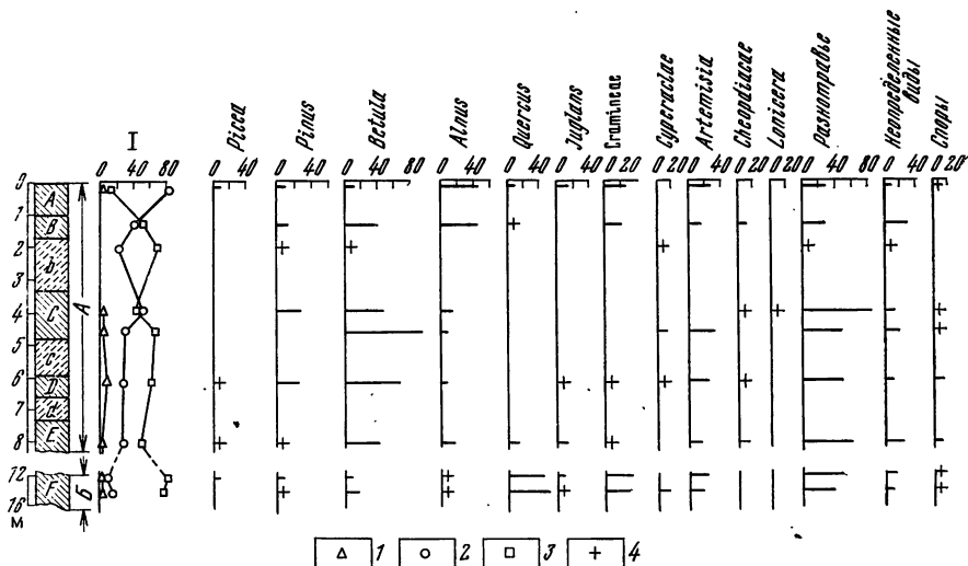
Рис. 16. Диаграмма спорово-пыльцевого анализа шурфа 44 (А) и стенки срыва оползня (Б) в верховье р. Чимган
