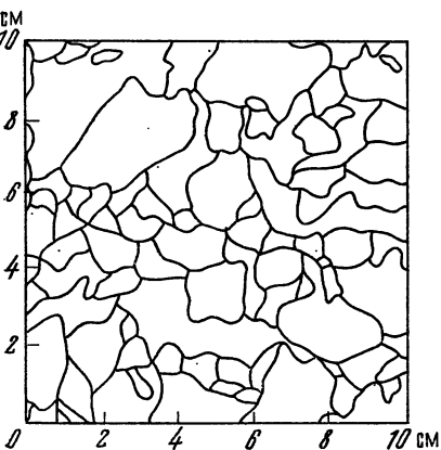
Рис. 10. Вертикальный срез почвы B отполированной стенки шурфа 39
