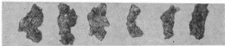
Рис. 19. Формы и размеры конкреций журавчиков из лёссовых суглинков b Чарвакской котловины
