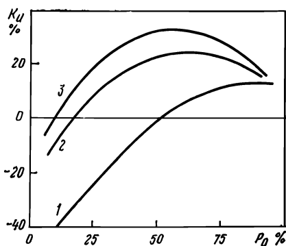
Рис. 5. Зависимости коэффициентов подпитывания злаковых трав от обеспеченности осадками на дерново-подзолистой (1), торфянисто-глебовой (2) и низинно-болотной (3) почвах.
