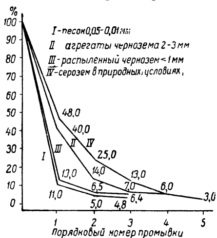
Рис. 35. Кривые выщелачивания \text{CaCl}_2 водой.
