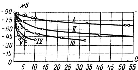
Рис. 3. Изменение электрокинетического потенциала в милливольты золя трехсернистого мышьяка в присутствии комплексных солей кобальта различной валентности (С — концентрация соли).
