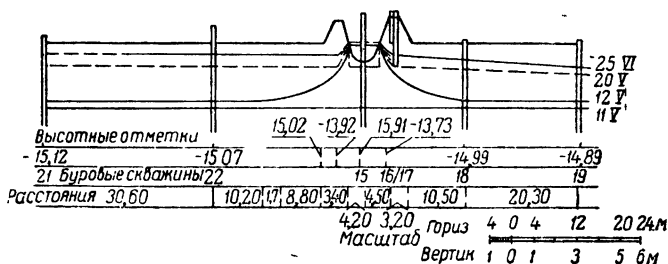
Рис. 117. Разрез поперечника буровых скважин через Ново-Харьковскую оросительную ветвь на Джафарханской опытной станции (Ф. П. Саваренский).
