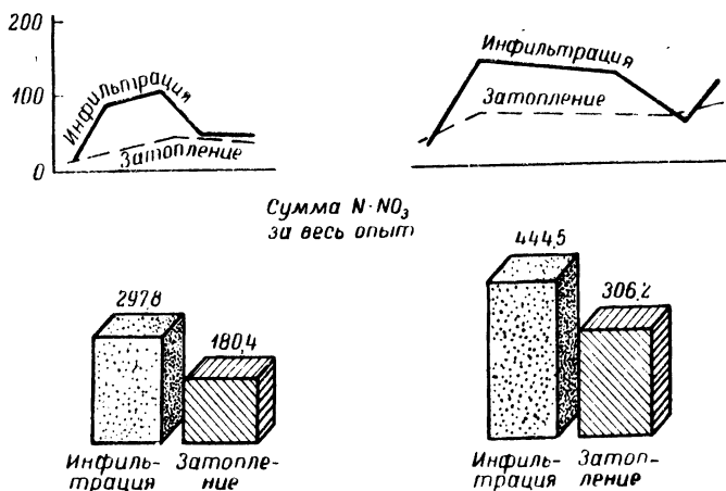
Рис. 88. Диаграмма процесса нитрификации при затоплении и инfiltrации. Динамика нитратного азота в миллиграммах на 1 кг почвы (Гельцер).
