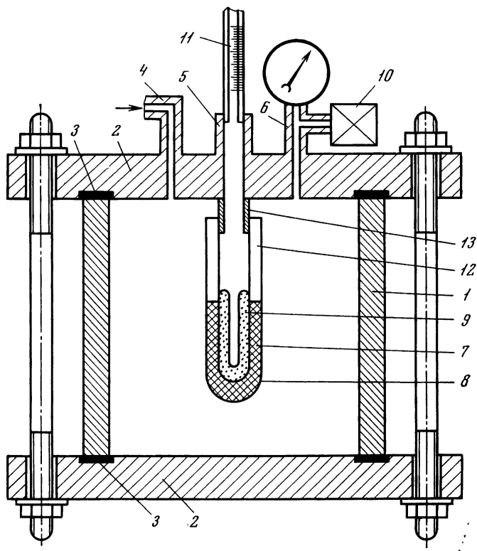
Рис. 7. Мембранный компрессор (вертикальный разрез, схема)
