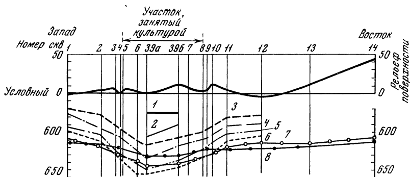
Рис. 26. Депрессия почвенно-грунтовых вод под темной почвой большой падьи с чистой культурой вяза мелколистного. Джаныбек, 1955 г. 1 — 19 апреля; 2 — 24 мая; 3 — 9 июня; 4 — 1 июля; 5 — 30 июля; 6 — 30 августа; 7 — 22 октября; 8 — 2 декабря
