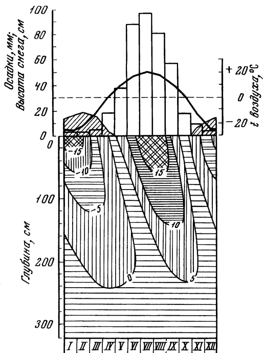
Рис. 8. Термоизоплеты почвы
