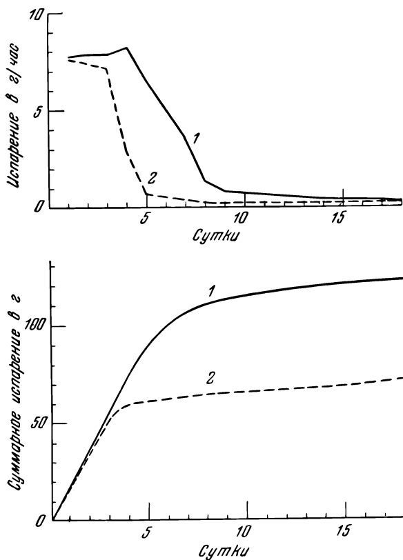
Рис. 65. Ход испарения капиллярно подвешенной влаги из песчаных колонн с разрывами и без них (по данным Малянова).
