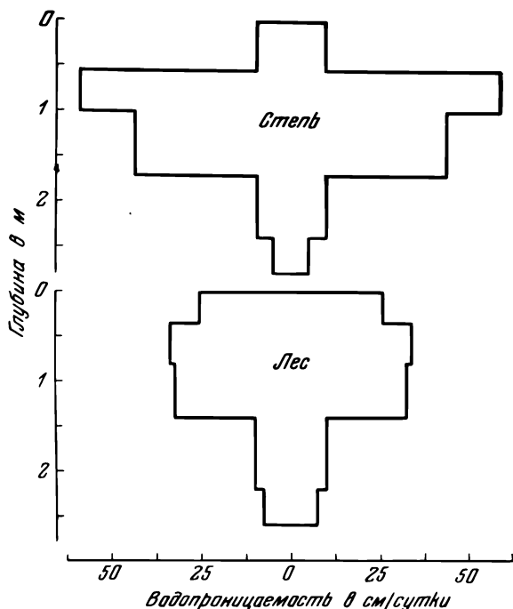
Рис. 73. Изменение водопроницаемости по профилю мощного суглинистого чернозема под целинной степью и под лесом (по данным Долгополовой).
