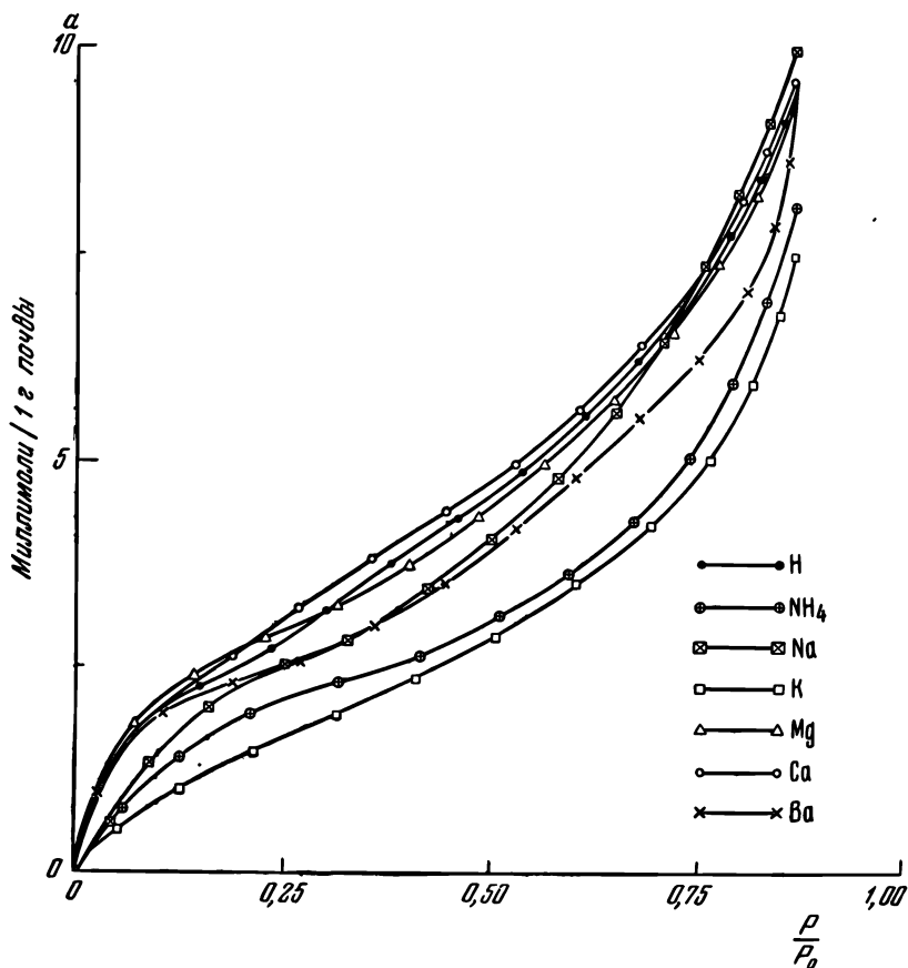
Рис. 25. Изотермы сорбции водяного пара глин, насыщенной различными катионами (данные Курона).
