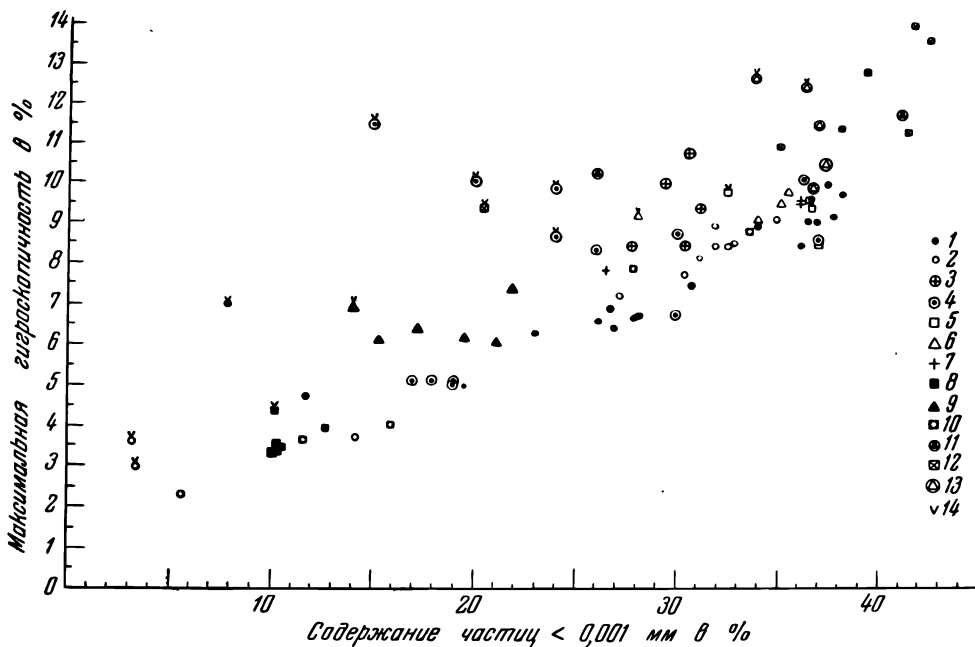
Рис. 29. Зависимость величины МГ от содержания частиц меньше 0,001 мм.
