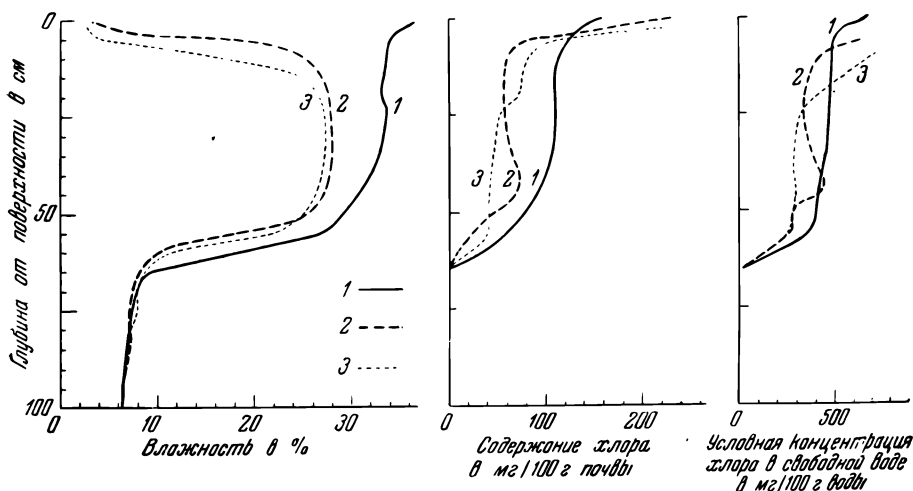
Рис. 58. Изменение распределения подвешенной воды, помеченной ионом хлора, в растертом черноземе в процессе ее испарения (по данным Абрамовой).
