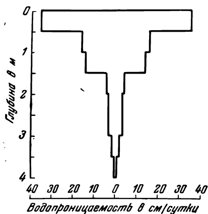
Рис. 72. Изменение водопроницаемости по профилю дерново-среднеподзолистой почвы, развитой на легком покровном суглинке, подстилаемом тяжелым песчаным суглинком (по Васильеву).
