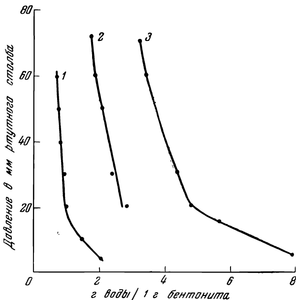
Рис. 40. Зависимость между содержанием воды в бентоните и давлением отсасывания (по данным Маттсона).
