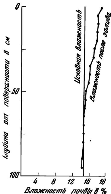
Рис. 60. Ход промачивания колонны легкого суглинки, предварительно увлажненного до величины ВРК (по данным Абрамовой).
