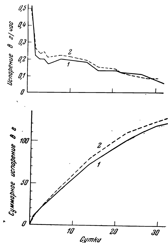
Рис. 66. Ход испарения стыковой влаги из песчаных колонн с разрывами и без них (по данным Малянова).
