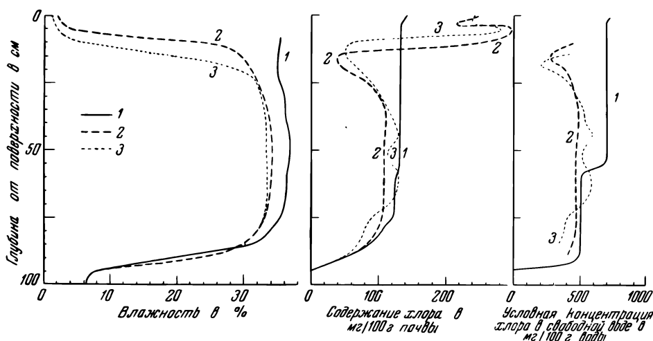
Рис. 57. Изменение распределения в структурном черноземе подвешенной влаги, помеченной ионом хлора, в процессе ее испарения (по данным Абрамовой).
