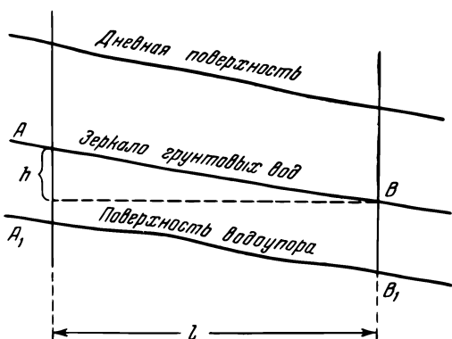
Рис. 85. Боковой внутрипочвенный сток.
