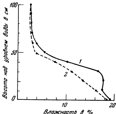
Рис. 64. Распределение воды в песчаной колонне при стекании и при капиллярном подъеме (по Лебедеву).
