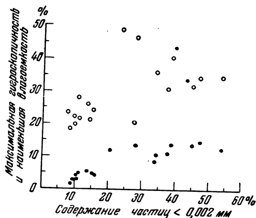
Рис. 51. Зависимость величин МГ и НВ (в насыпных колоннах) от содержания частиц меньше 0,001 мм (составлено по данным Долгова). Точки — максимальная гигроскопичность, кружки — наименьшая влагоемкость.
