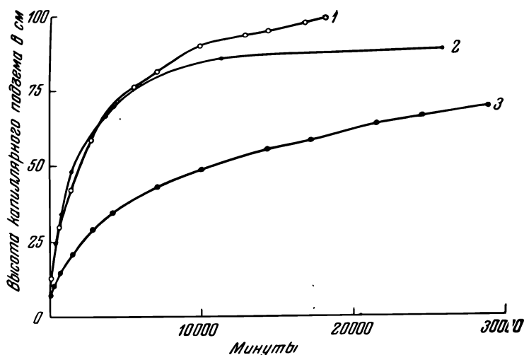
Рис. 82. Зависимость высоты подъема в почвенной толще от времени (по Васильеву).
