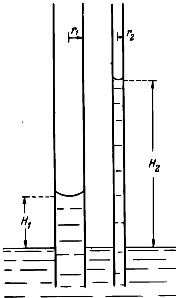
Рис. 12. Равновесное расположение воды в цилиндрических капиллярах различного диаметра.
