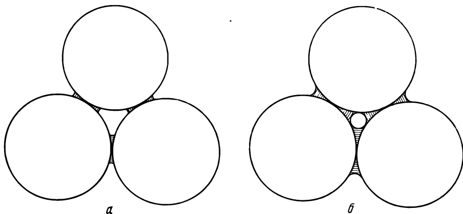
Рис. 18. Возникновение и смывание манжет стыковой воды между шарообразными частицами.
