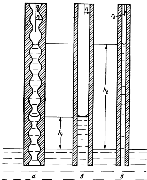
Рис. 14. Равновесие воды в четочном капилляре.
