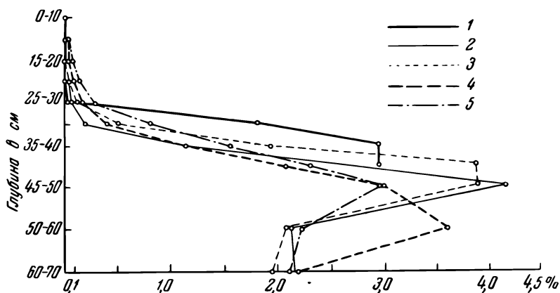
Рис. 53. Распределение NaCl в трубках в опыте Летунова с сотрудниками.
