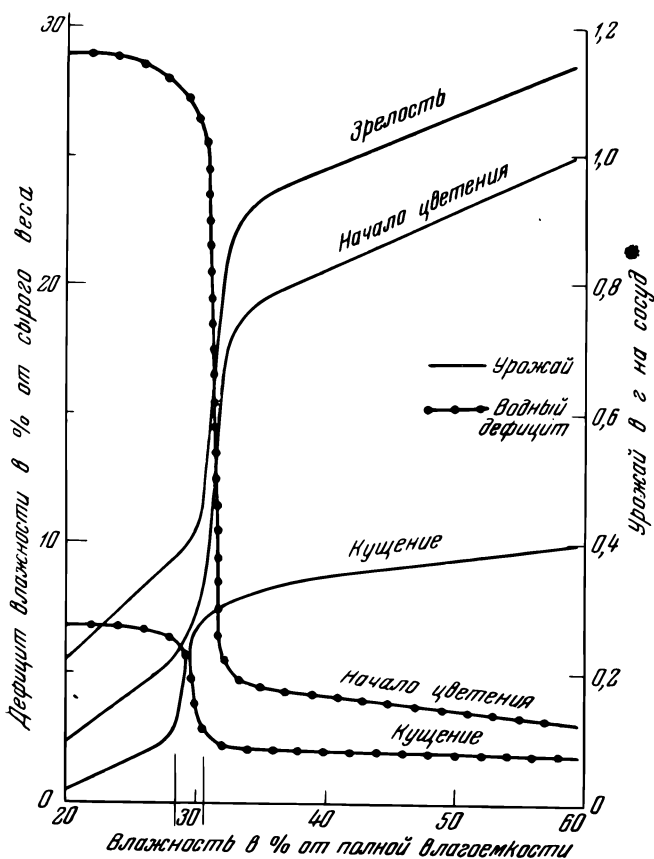
Рис. 94. Зависимость величины урожая и водного дефицита в растениях от влажности почвы (по данным Колотовой).
