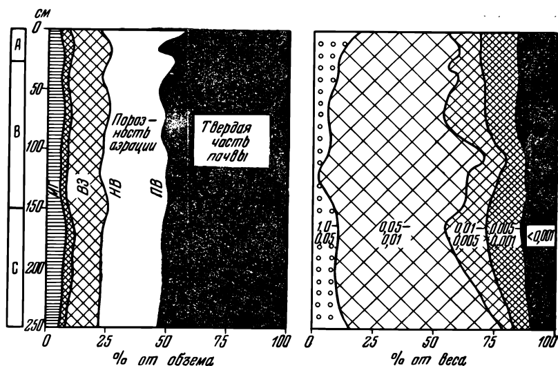
Рис. 107. Водные свойства и механический состав типичного богатого серозема (по данным Большакова)
