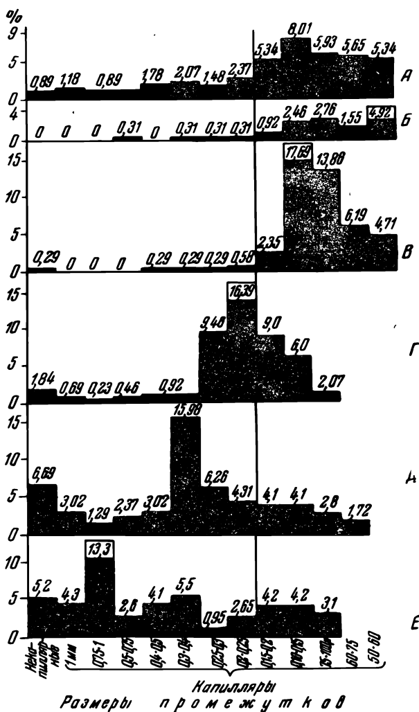
Рис. 93. Содержание пор различного размера (в процентах от общей порозности) в различных структурных фракциях чернозема и в нерассеянной почве (по Дояренко).
