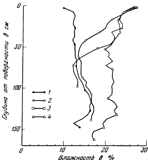
Рис. 49. Распределение воды в почве при различных нормах полива (по данным Иванова).
