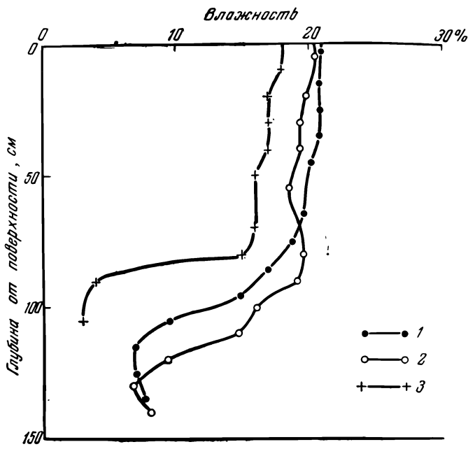
Рис. 48. Распределение подвешенной воды в почвах после полива
