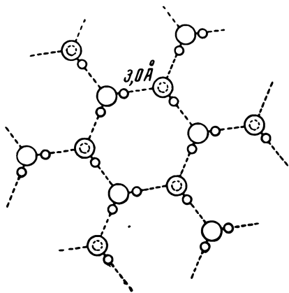
Рис. 41. Плоский слой сорбированных молекул воды, связанных одна с другой в гексагональную сетку (по Хендриксу и Джефферсону).
