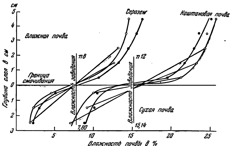
Рис. 96. Влажность почвы на нижней границе промачивания и влажность завядания (по Долгову).
