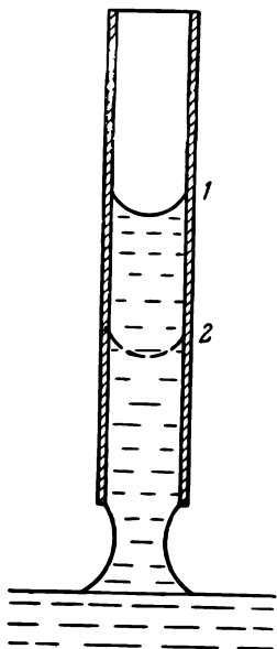
Рис. 63. Понижение верхней границы капиллярной каймы при вынимании нижнего конца колонны из сосуда с водой.
