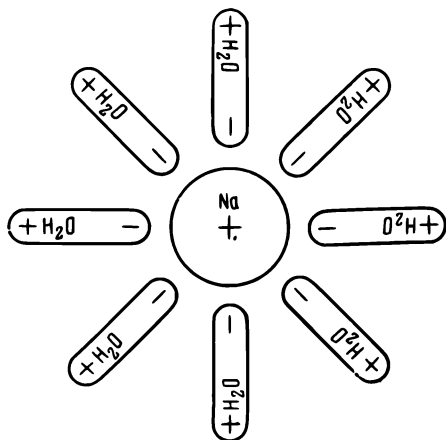
Рис. 7. Гидратированный ион натрия, окруженный дипольными молекулами воды.
