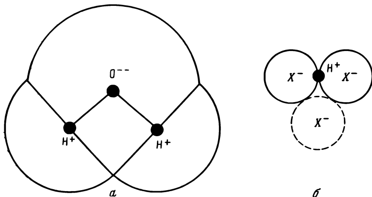
Рис. 8. Строение молекулы (а) и водородная связь по Паулингу (б).
