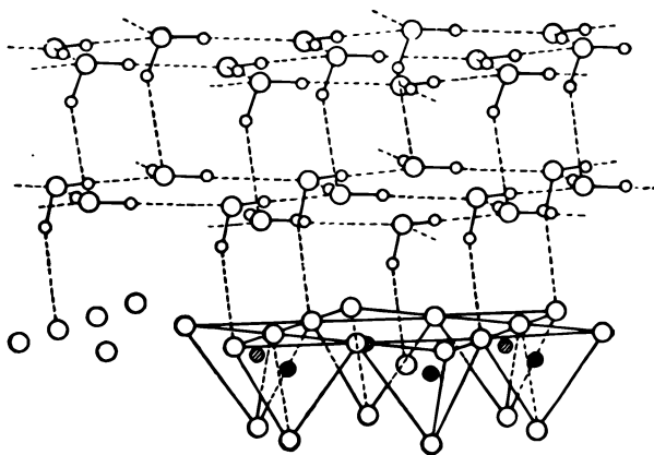
Рис. 42. Слои сорбированных молекул воды над поверхностью кристалла глининого минерала.
