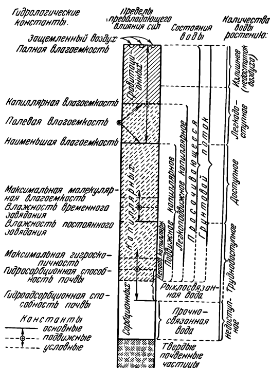
Рис. 97. Подразделение форм почвенной влаги (по Долгову).
