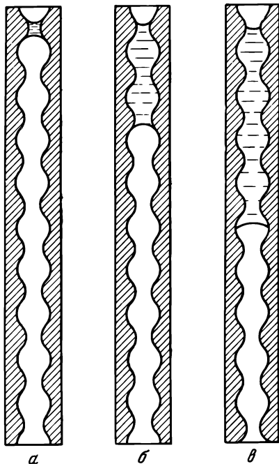
Рис. 15 Капиллярно подвешенная вода в четочном капилляре.
