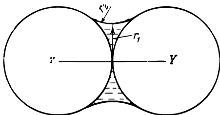
Рис. 17. Водная манжета (стыковая вода) между двумя шарообразными частицами.
