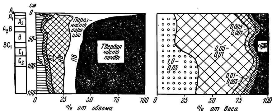
Рис. 104. Водные свойства и механический состав дерново-среднеподзолистой почвы, развитой на легком покровном суглинке, подстилаемом тяжелым песчаным суглинком (по Васильеву)
