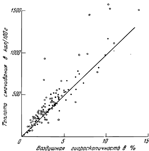
Рис. 37. Зависимость теплоты смачивания от величины воздушной гигроскопичности почв (по данным Андрианова и Пури и Хууна).
