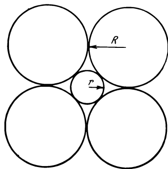
Рис. 2. Соприкосновение четырех шарообразных частиц при кубической упаковке.
