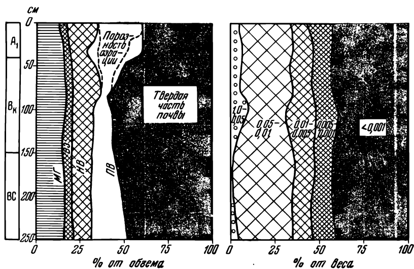
Рис. 106. Водные свойства и механический состав южного солончакового чернозема, развитого на легкой покровной глине (по данным Афанасьевой)
