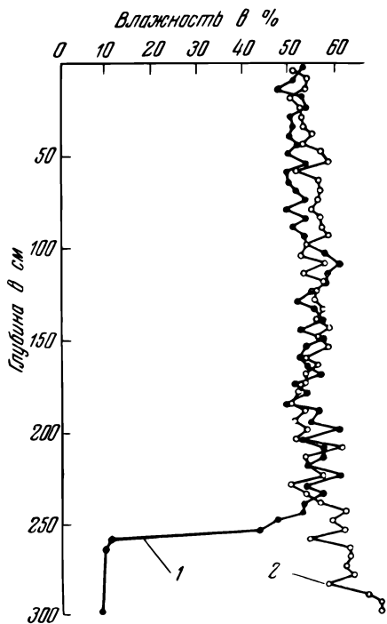
Рис. 50. Распределение воды в насыпных колоннах краснозема (по Долгову).
