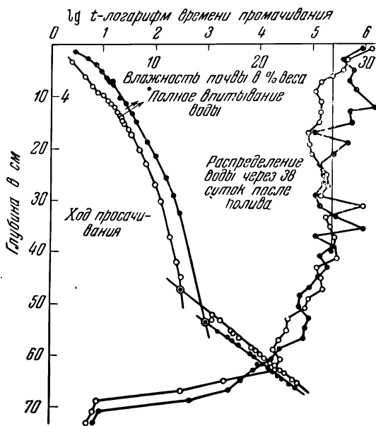
Рис. 47. Ход просачивания воды в слабо оподзоленной окультуренной супесчаной почве и распределение влаги в конце опыта. Два параллельных опыта (по данным Долгова).
