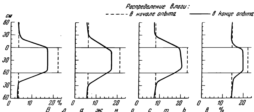
Рис. 100. Передвижение влаги из влажной почвы в сухую. Опыты с паспынными колоннами почвы (по Вимейеру).
