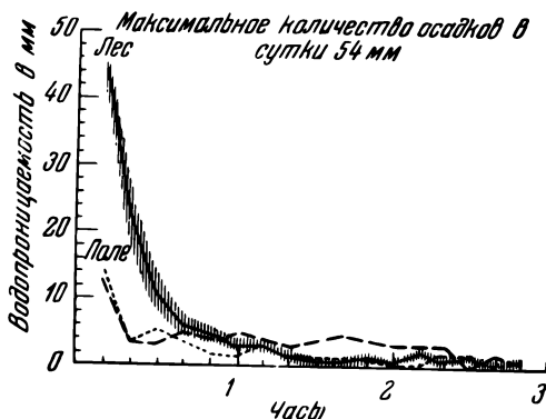
Рис. 70. Изменение во времени коэффициента впитывания тяжелосуглинистой подзолистой почвы на моренном суглинке. Московская область (по Созыкину).
