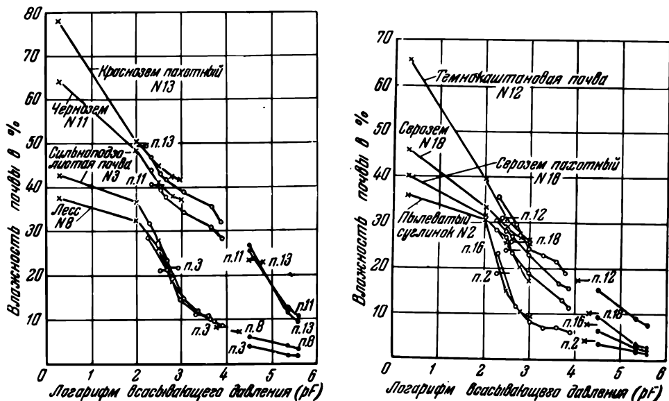
Рис. 90. Зависимость сосущей силы почвы (логарифм всасывающего давления) от влажности почвы (по Долгову).
