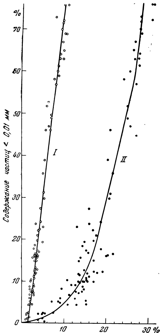
Рис. 52. Зависимость величин наименьшей влагоемкости и влажности завядания от содержания частиц меньше 0,01 мм (по данным Вилькокса и Спилсбюри).
