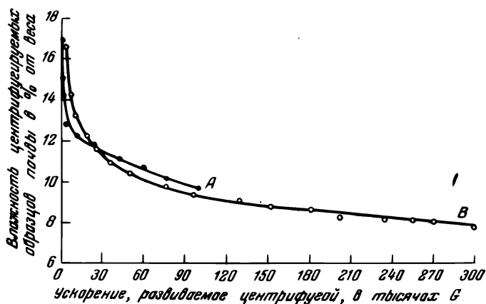
Рис. 31. Зависимость содержания остаточной влаги от ускорения центрифуги (по Олмстэду).
