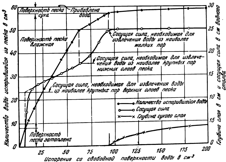
Рис. 67. Ход испарения влаги из песчаной колонны, изменение сосущей силы в процессе испарения и изменения мощности сухого слоя (по Вуудрэффу).
