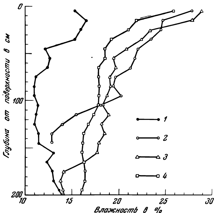
Рис. 46. Распределение подвешенной влаги в почве через различные сроки после полива (по Уласевичу).
