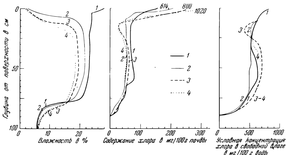
Рис. 59. Изменение распределения подвешенной воды, помеченной ионом хлора, в тяжелом суглинке в процессе ее испарения (по данным Абрамовой).
