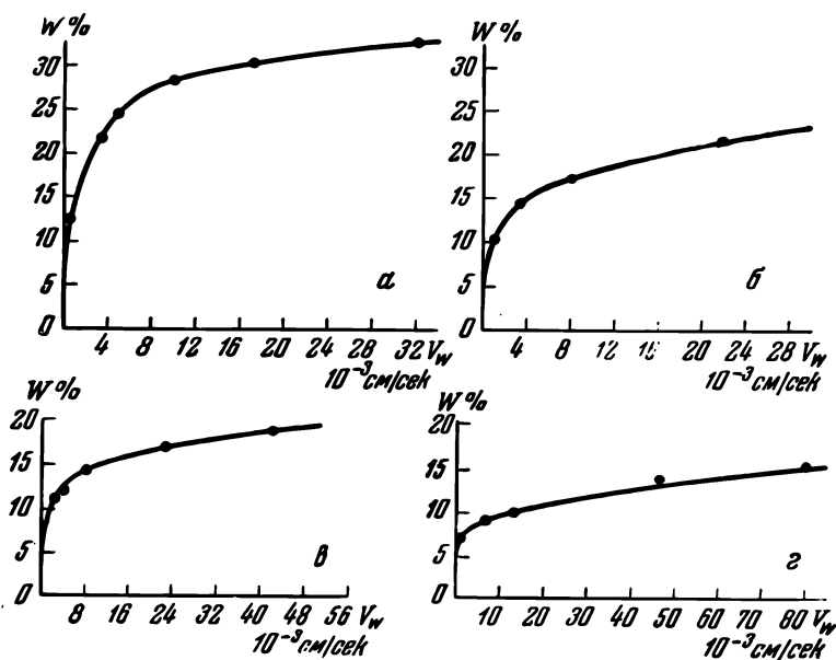
Рис. 75. Кривые зависимости скорости инфильтрации v_w от объемной влажности w для песков разных фракций.
