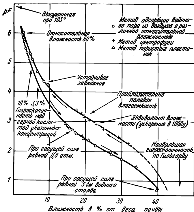
Рис. 91. Зависимость сосущей силы почвы ( pF — логарифм всасывающего давления) от влажности почвы в процессе оводнения (нижняя кривая) и в процессе иссушения (верхняя кривая) (по Скофилд).
