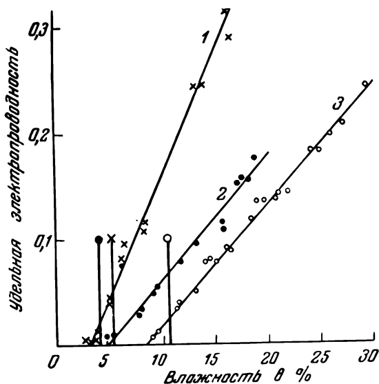
Рис. 34. Зависимость электропроводности почвы от ее влажности. Вертикальными линиями отмечена величина МГ (по данным Долгова).
