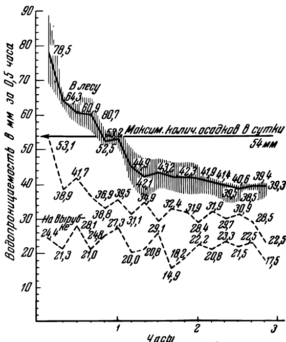
Рис. 69. Изменение во времени коэффициента впитывания супесчаной лесной почвы. Московская область (по Созыкину).
