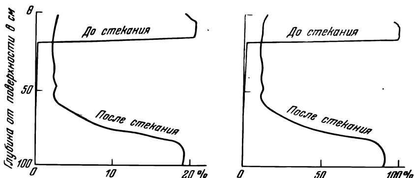
Рис. 44. Распределение капиллярно подвешенной воды в верхнем слое песчаной толщи (по данным Васильева)
