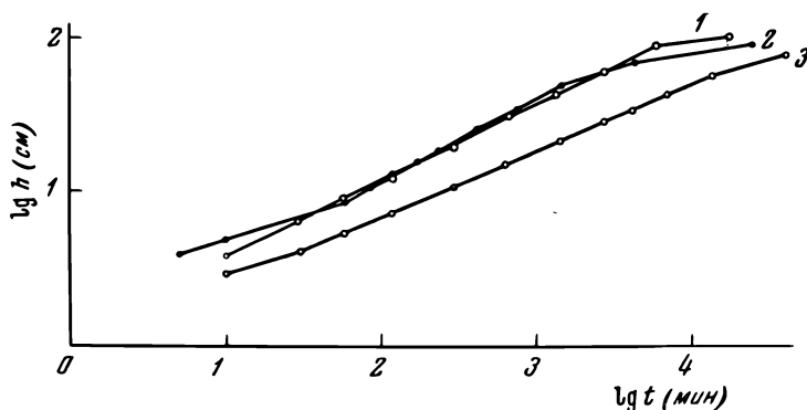
Рис. 83. Зависимость высоты подъема в почвенной толще от времени. Логарифм высоты по логарифму времени (по данным Васильева).
