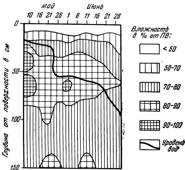
Рис. 76. Колебания уровня почвенно-грунтовых вод на фоне влажности почвы (по данным Васильева).
