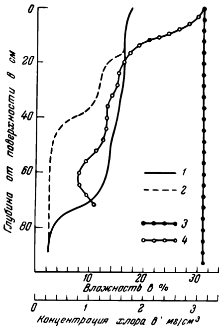
Рис. 98. Вытеснение чистой воды из колонны легкого суглинка раствором хлористого кальция (по данным Абрамовой)
