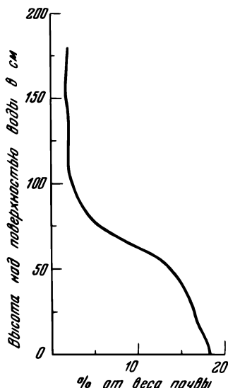
Рис 77. Равновесное распределение влаги в песчаной колонне после стекания избыточной воды (по Прокурникову).
