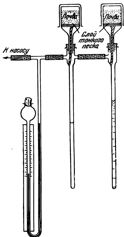
Рис. 88. Вакуум-капилляриметр Секера (рисунок заимствован из книги Долгова)
