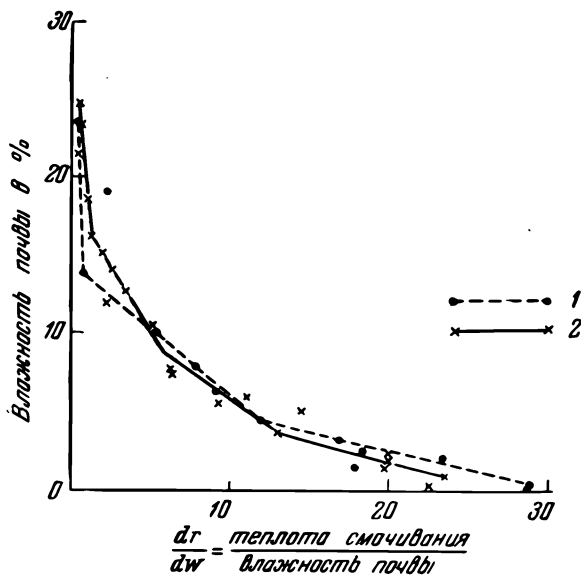
Рис. 36. Зависимость отношения \frac{dr}{dw} от влажности почвы (по данным Митчерлиха)
