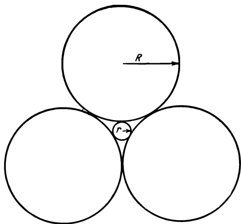
Рис. 5. Соприкосновение трех частиц при гексагональной упаковке.
