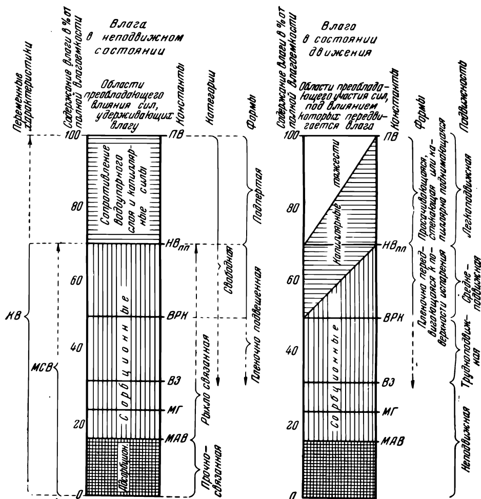
Рис. 102. Подразделение форм почвенной влаги. Почвы и грунты тонкозернистые.
