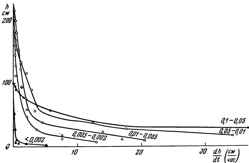
Рис. 81. Изменение скорости подъема в насыпных колонках из частиц разного размера в зависимости от высоты подъема (по данным Новака и Печанека).
