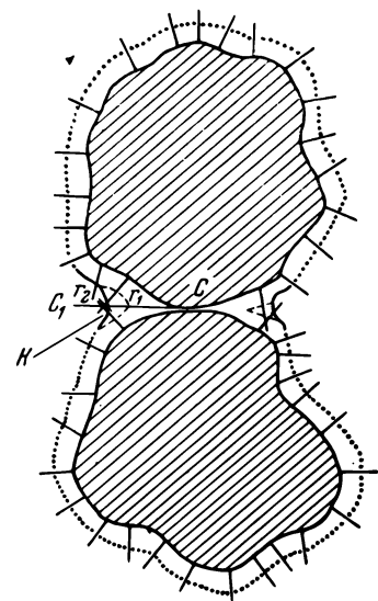
Рис. 24. Образование выпукло-вогнутого мениска в результате слияния пленок адсорбированной воды в точке контакта двух частиц.
