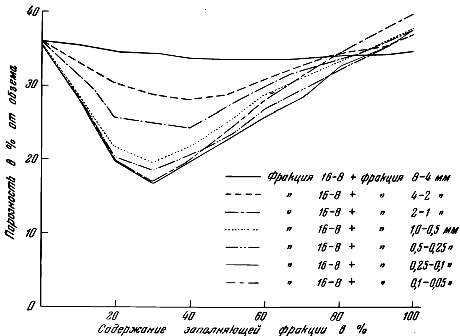
Рис. 6. Порозность в смесях частиц различных фракций (по Охотину).
