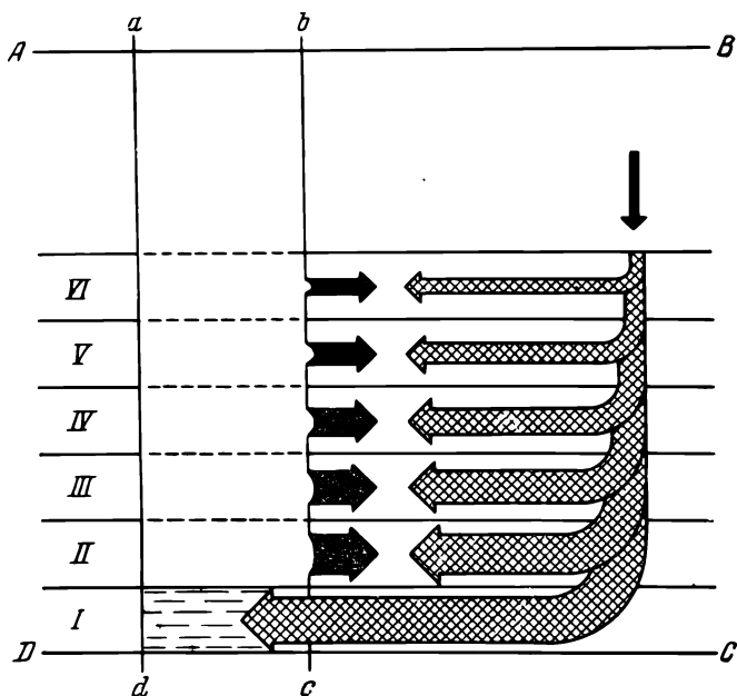
Рис. 68. Схематическое изображение соотношений между гидростатическим и поверхностным давлением над зеркалом грунтовой воды и под ним.
