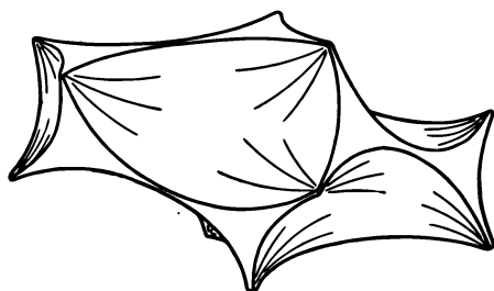
Рис 4. Слпок порового пространства при гексагональной упаковке.
