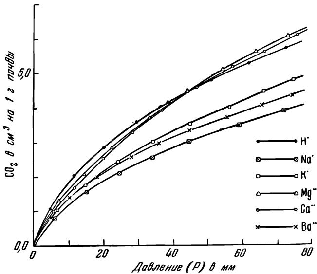
Рис. 28. Изотермы сорбции углекислоты почвой, насыщенной различными катионами (по данным Курона).
