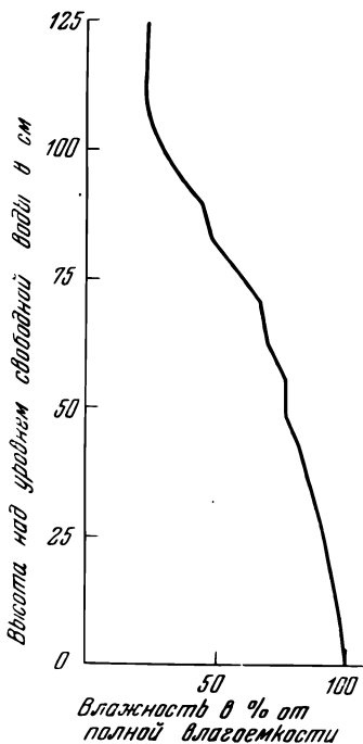
Рис. 78. Распределение капиллярно подпертой влаги в почвенной толще (по данным Васильева)
