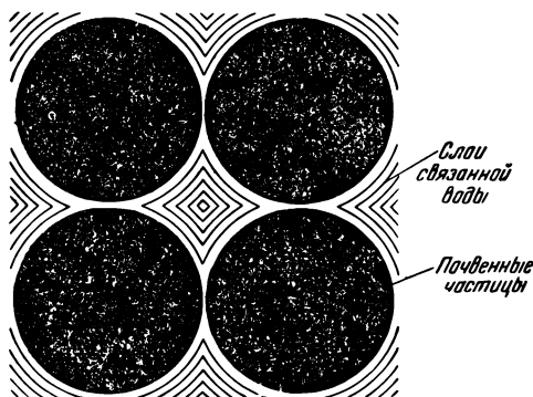
Рис. 61. Схематическое изображение слоев связанной воды, сплошь заполняющих поровое пространство.
