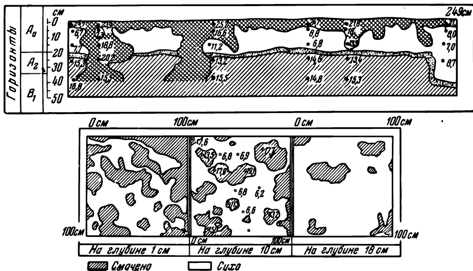
Рис. 71. Неравномерность проникновения дождевой воды в тяжелосуглинистую подзолистую почву.
