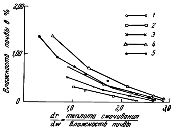
Рис. 35. Зависимость отношения \frac{dr}{dW} от влажности почвы (по данным Митчерлиха).
