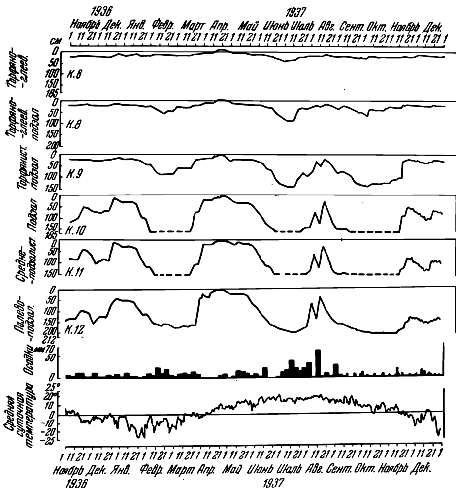
Рис. 84. Колебания уровня почвенно-грунтовых вод в толще подзолистых, болотно-подзолистых и болотных почв (по Роде).
