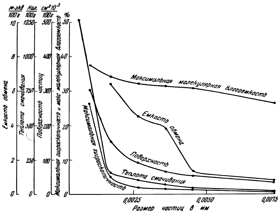
Рис. 32. Зависимость величин ММВ, емкости обмена, суммарной поверхности, теплоты смачивания и МГ от размера частиц (по данным Мельникова).
