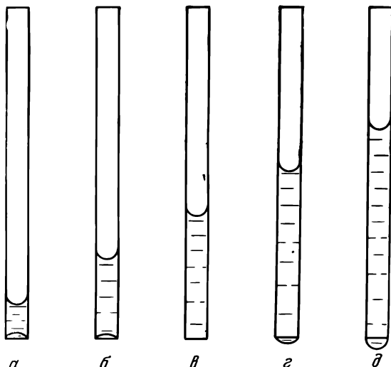
Рис. 13. Подвешенная влага в цилиндрическом капилляре.
