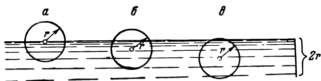
Рис. 9. Поверхностный слой жидкости.
