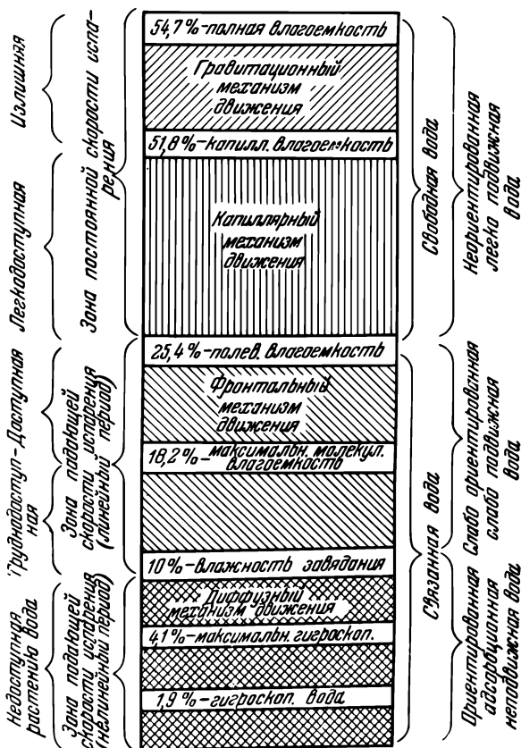
Рис. 99. Схема классификации форм почвенной влаги Колясева. Данные относятся к сильноподзолистой тяжелосуглинистой почве.
