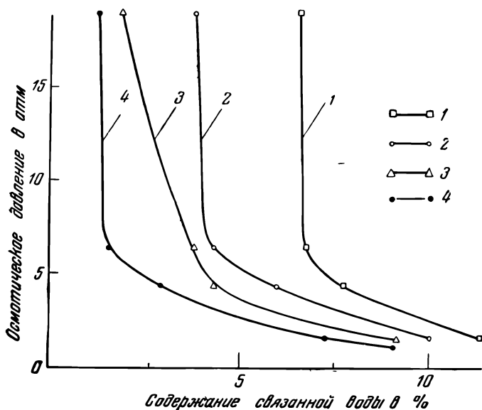
Рис. 33. Зависимость содержания связанной воды в почвах от осмотического давления равновесного раствора сахара (по данным Долгова).
