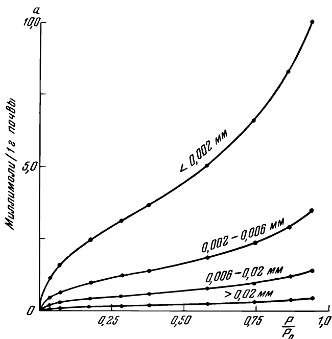
Рис. 20. Кривые зависимости количества парообразования влаги, адсорбированной почвой, от относительной упругости пара. Почва из Версингаве (по данным Курона).
