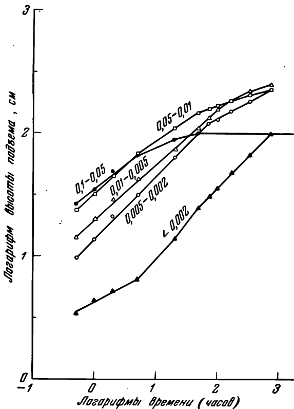
Рис. 80. Капиллярный подъем в насыпных колоннах из частиц разного размера. Логарифм высоты по логарифму времени (по данным Новака и Печанека).
