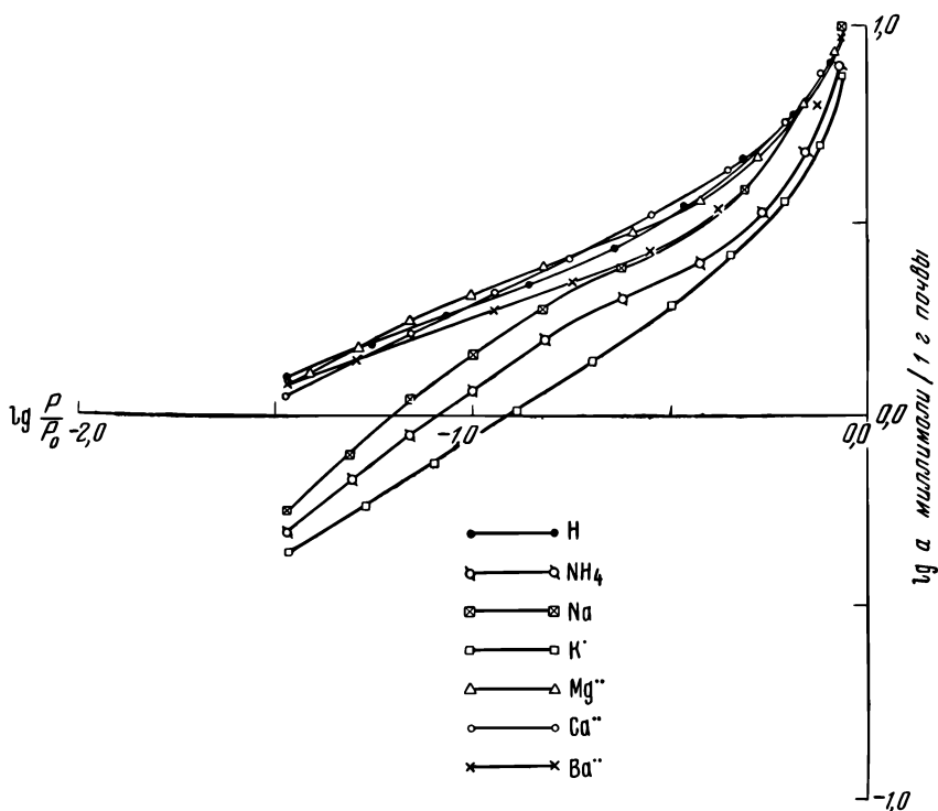
Рис 26 Изотермы адсорбции водяного пара глиной, насыщенной различными катионами, в логарифмической форме (данные Курона)
