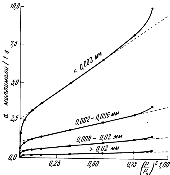
Рис. 22. Кривые зависимости количества адсорбированной почвой парообразной влаги от относительной упругости водяного пара. Почва из Версингаве (данные Курона, обработанные по уравнению Сперанского)
