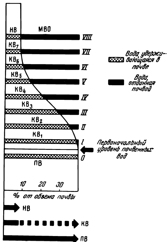
Рис. 86. Соотношение между полной, капиллярной и наименьшей влагоемкостями и водоотдачей (схема).
