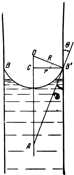
Рис. 11. Мениск в цилиндрическом капилляре.
