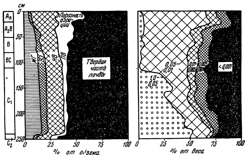
Рис. 103. Водные свойства и механический состав дерново-среднеподзолистой почвы, развитой на тяжелом покровном суглинке, подстилаемом на глубине 240 см валунным суглинком (по Васильеву)
