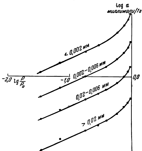
Рис. 21. Кривые зависимости количества паровоздушной влаги, адсорбированной почвой, от относительной упругости водяного пара в логарифмической форме. Почва из Версингаве (по данным Курона).
