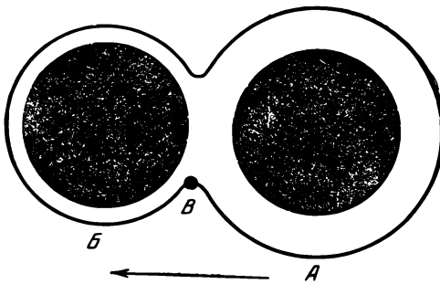
Рис. 30. Передвижение пленочной воды от одной частицы к другой.
