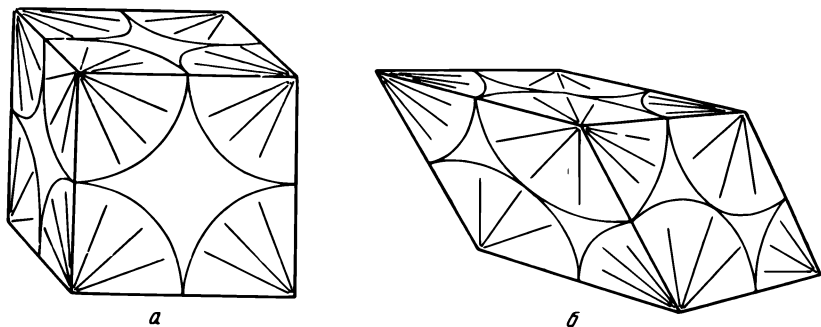
Рис. 1. Шарообразные частицы в кубической (а) и гексагональной (б) упаковке.
