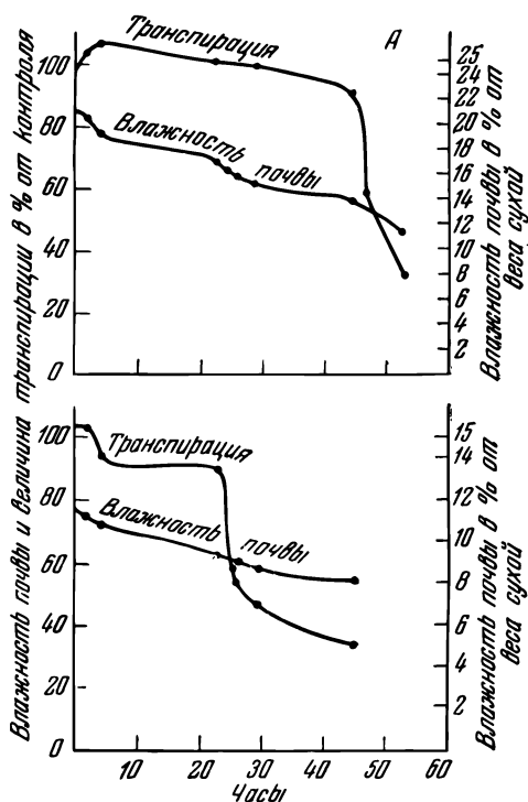
Рис. 95. Зависимость величины транспирации от влажности почвы (по данным Кокиной).
