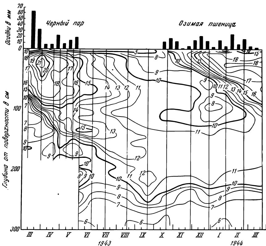
Рис. 54. Изменение влажности богарного серозема под черным паром (по данным Большакова).
