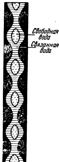
Рис. 62. Скопления свободной, сорбционно замкнутой воды, отделенные друг от друга пробками связанной воды.
