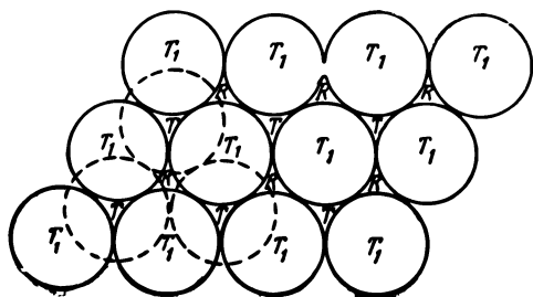
Рис. 3. Расположение ромбоэдрических ( R ) и тетраэдрических ( T ) пор при гексагональной упаковке.
