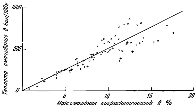
Рис. 38. Зависимость теплоты смачивания почв от величины МГ (по данным Андрианова, Димо и Цункера).
