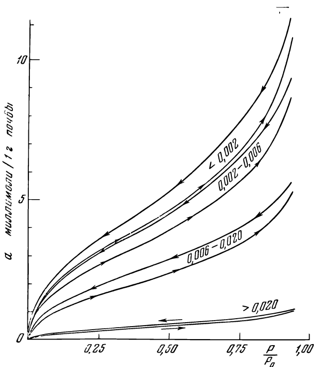
Рис. 23. Гистерезис адсорбции водяного пара почвой (данные Курона).
