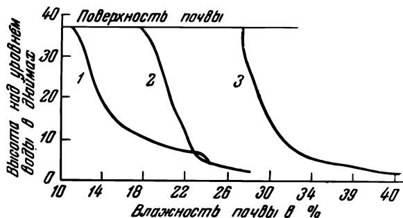
Рис. 87. Зависимость величины капиллярного потенциала от влажности почвы (по Бэкингему). 1 — песчанистый суглинок Норфольк; 2 — суглинок Леонардтоун; 3 — глина Сессиль.
