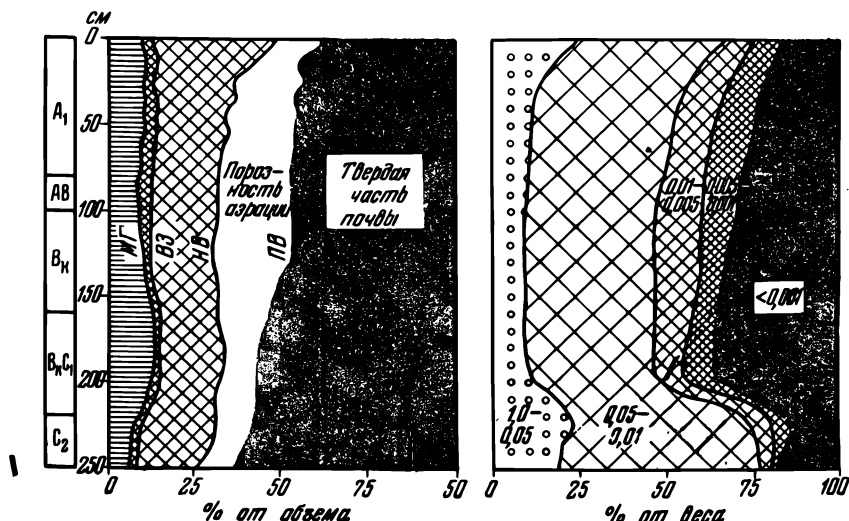
Рис. 105. Водные свойства и механический состав мощного тучного суглинистого чернозема, развитого на тяжелом лессовидном суглинке, подстилаемом с 220 см средним лессовидным суглинком (по данным Афанасьевой и Большакова)
