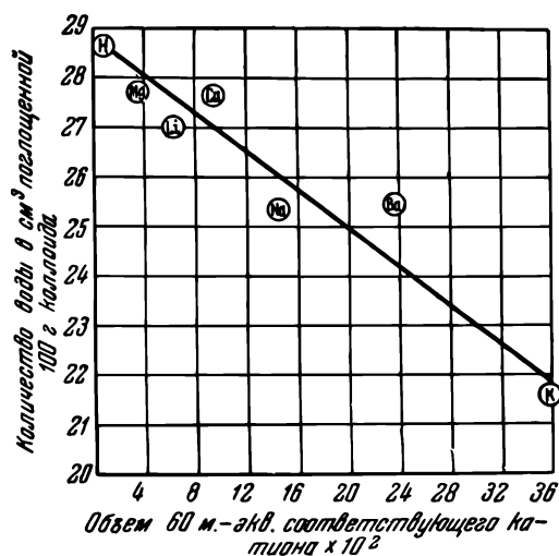
Рис. 27. Зависимость количества влаги, сорбированной почвенными коллоидами, насыщенными различными катионами, от объема обменных катионов (по Бевеу и Хорнеру).
