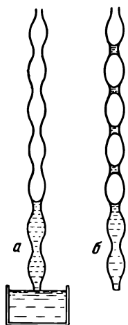
Рис. 43. Расположение воды между гофрированными пластинками (по Коссовичу).
