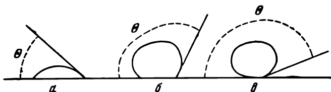
Рис. 10. Хорошее (а), среднее (б) и плохое (в) смачивание.
