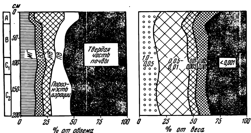
Рис. 108. Водные свойства и механический состав глубоколбчатого солонча (по данным Малянова)
