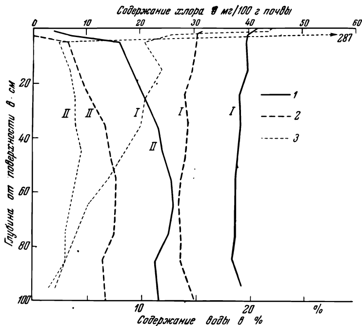
Рис. 55. Изменение содержания влаги и хлора в богарном серо-земле при испарении подвешенной воды (полевой опыт Большакова).
