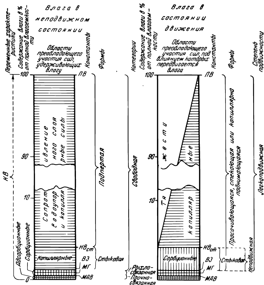
Рис. 101. Подразделение форм почвенной влаги. Почвы и грунты крупно- и среднезернистые.
