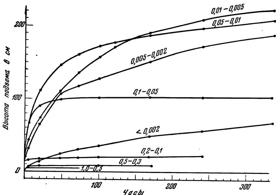
Рис. 79. Капиллярный подъем в насыпных колоннах, составленных из частиц различного размера (по Новаку и Печанеку).
