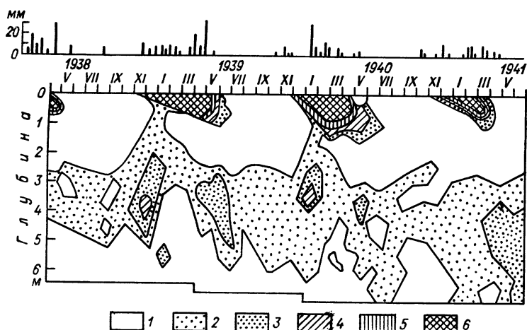
Рис. 7. Изоплеты влажности песка под черносаксаульником [13].
