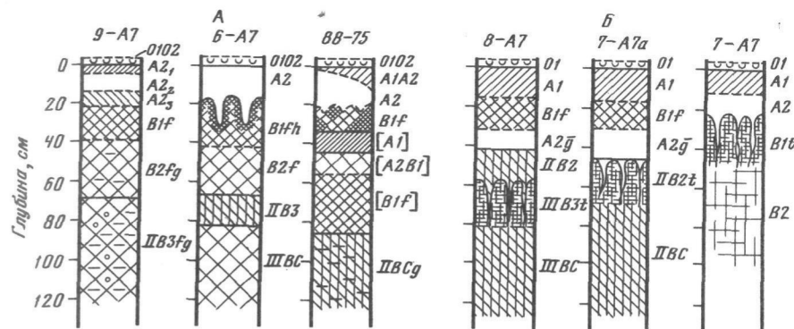
Рис. 13. Строение почвенных профилей в районе метеоритных кратеров А — метеоритный кратер Пыргухауд; Б — то же, Сювахуд
