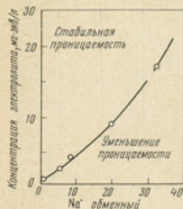
Рис. 19. Концентрация электролита, необходимая для поддержания проницаемости почв при различном содержании обменного Na + (Quirk, Schofield, 1955)
