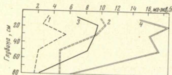
Рис. 18. Динамика щелочности в почвенных растворах орошаемых почв Ферганской долины До полива, 7 июля: 1 — \text{CO}_3^{2-} ; 2 — \text{HCO}_3^- ; после полива 10 июля: 3 — \text{CO}_3^{2-} ; 4 — \text{HCO}_3^- .
