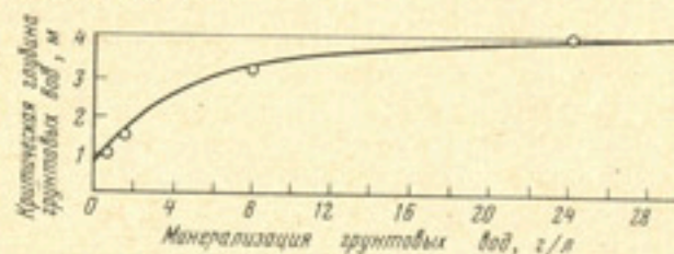
Рис. 2. Влияние минерализации грунтовых вод на засоление почв
