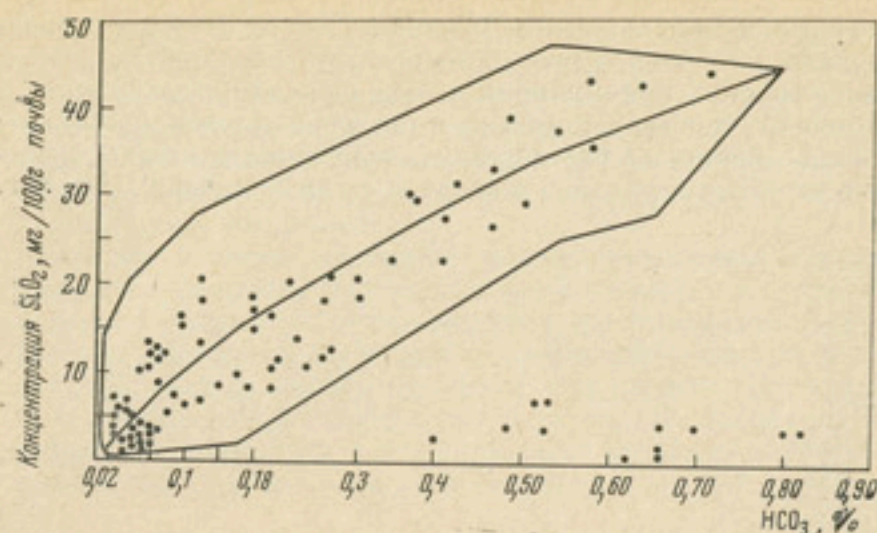
Рис. 6. Зависимость между концентрацией растворимой в воде SiO_2 и общей щелочностью почв
