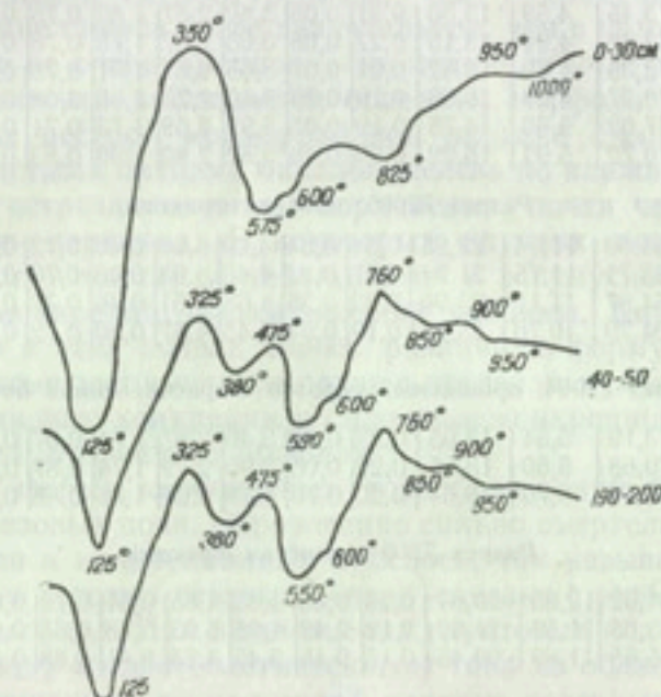
Рис. 14. Гермограммы коллоидно-илстой фракции орошаемого светлого серозема разреза 72005
