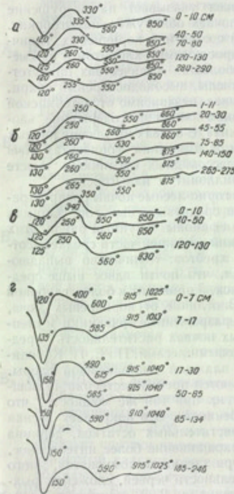
Рис. 15. Термограммы илстой фракции коричневых почв. а — разрез 30, б — разрез 9, в — разрез 35, г — разрез 106.
