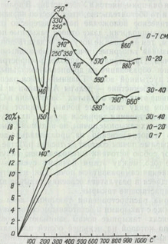
Рис. 5. Термограммы и кривые обезвоживания иллитовой фракции пустынной песчаной почвы разреза 7.
