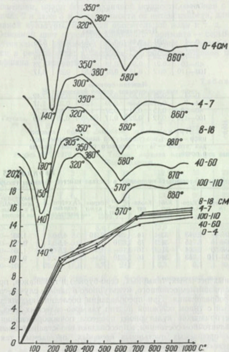
Рис. 8. Термограммы и кривые обезвоживания илистой фракции такыра разреза 8.
