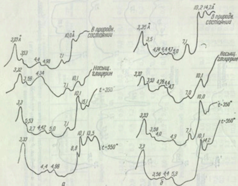
Рис. 10. Дифрактограммы коллоидно-илистой фракции типичного серозема разреза 7200/2 а — 45—55 см, б — 195—205 см.
