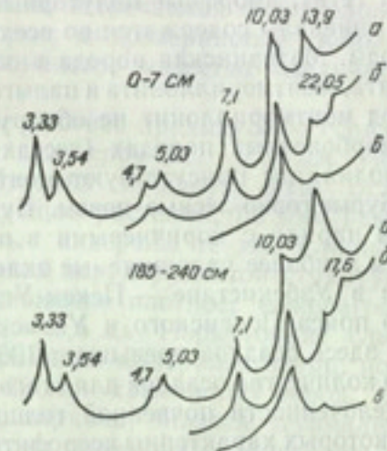
Рис. 16. Рентгенодифрактограммы илстой фракции коричневой почвы разреза 106. а — исходный образец, б — насыщенный тигленг-ликотем, в — нагретый при 550°.
