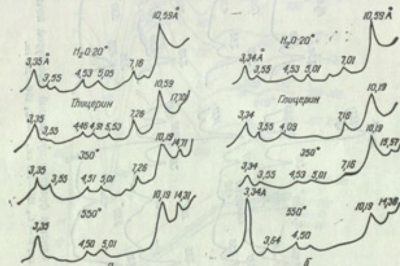
Рис. 1. Рентгенодифрактограммы илстой фракции пустынной серо-бурой почвы разреза 9. а — А, 0—9 см, б — В, 10—20 см.
