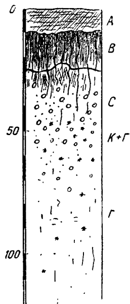
Фиг. 6. Солонец солончаковатый содово-сульфатный.
