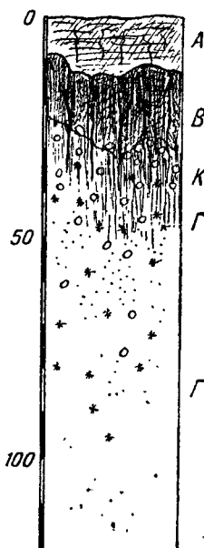
Фиг. 10. Солонец остаточно-солончаковатый.
