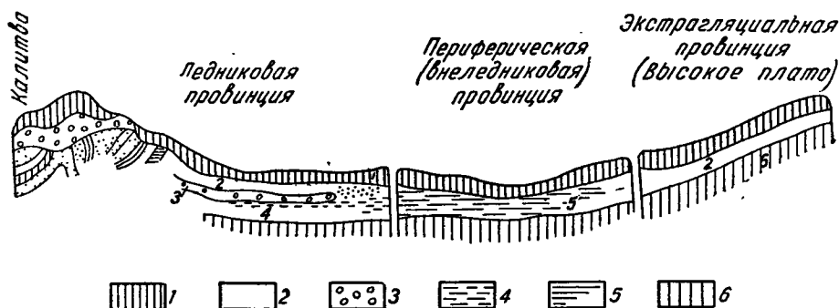
Фиг. 4. Схема соотношения морен и лёссовых ярусов в Днепровском языке 1 — Вюрмский лёсс, 2 — Надморенная часть рисского лёсса, 3 — Морена Днепровского оледенения, 4 — Подморенная часть рисского лёсса, 5 — Пресноводная фация рисского лёсса, 6 — Подрисская часть лёссовой свиты (из работы Л. Лундсбергаузен «О четвертичных отложениях у границы Днепровского языка»)
