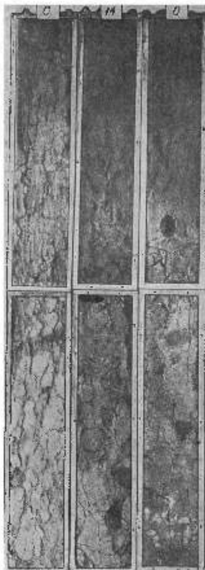
Фиг. 5. Сопоставляем степной и обыкновенный чернозем Украины (по Микшю).
