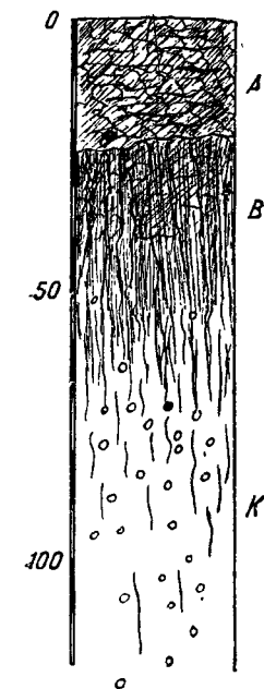
Фиг. 14. Солонец остепненный.
