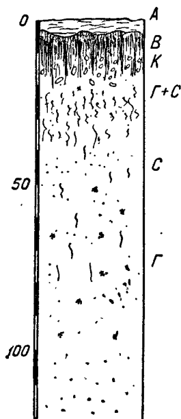
Фиг. 2. Солонец солончаковатый сульфатно-хлоридный.
