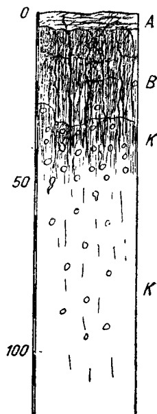
Фиг. 8. Солонец солончаковатый содовый.
