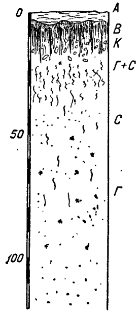
Фиг. 2. Солонец солончаковатый сульфатно-хлоридный.
