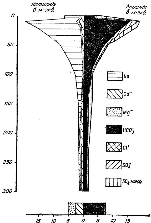
Фиг. 16. Солевой профиль содового солонца-солончака.
