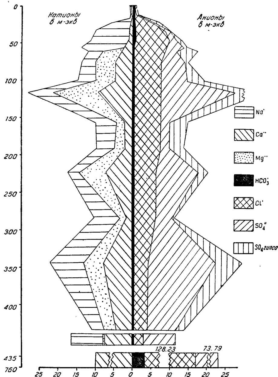
Фиг. 13. Солевой профиль остаточно-слабосолончакового солонца.
