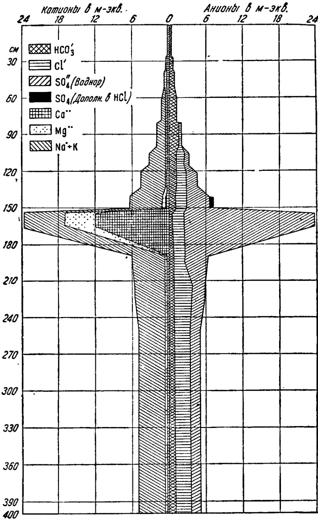
Фиг. 3. Разрез № 1714 (Красный Кут). Солевой профиль.
