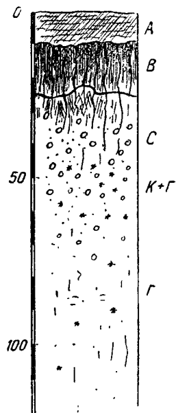
Фиг. 6. Солонец солончаковый содово-сульфатный.
