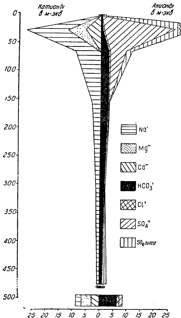
Фиг. 7. Солевой профиль содово-сульфатного солонца.
