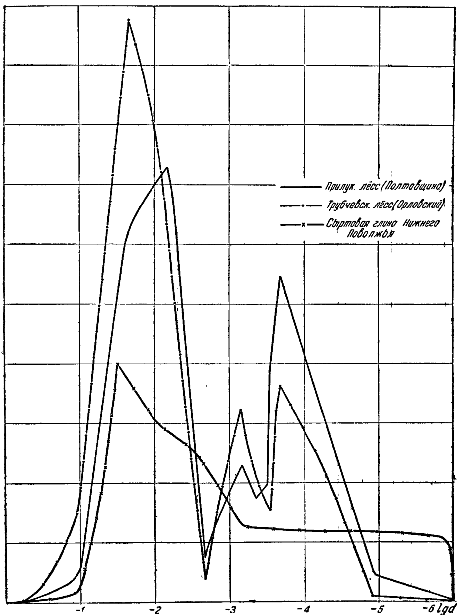
Ф г. 1. Кривые распределения механического состава материнских пород.
