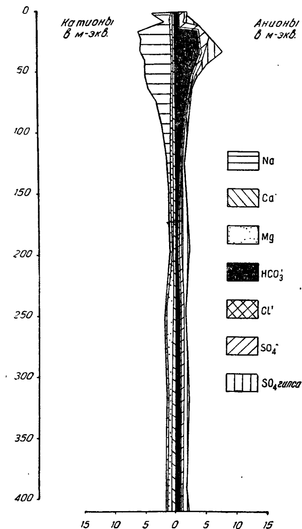
Фиг. 9. Солевой профиль содового солонца.
