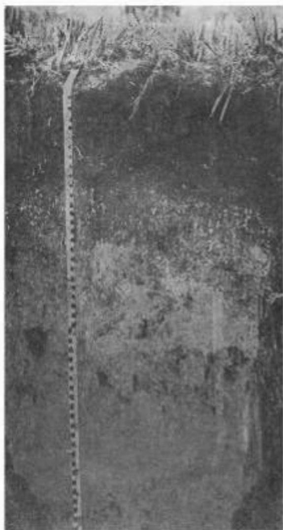
Фиг. 2. Профиль солончака у берегового берега пограничной области на территории г. Владивосток.
