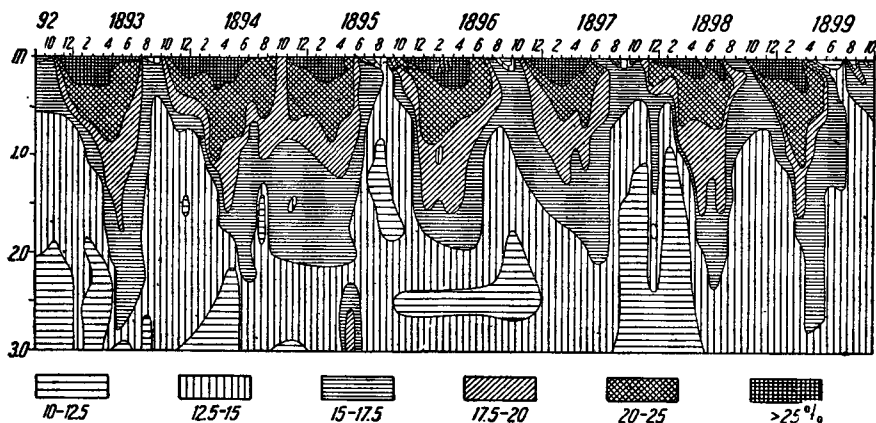
Фиг. 4. Линии равной влажности (хроноизоплеты) чернозема по наблюдениям Г. Н. Высоцкого за 7 лет в Велико-Анадольском степном лесничестве от поверхности до глубины 3 м.
