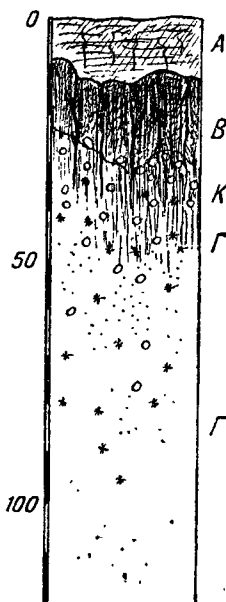
Фиг. 10. Солонец остаточно-солончаковатый.
