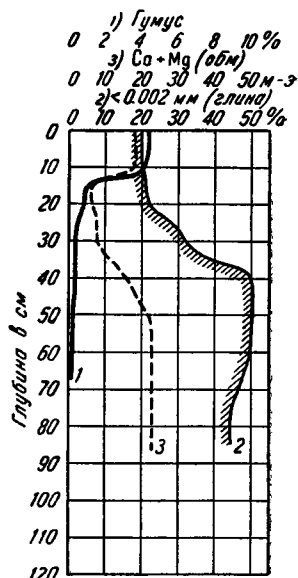
Фиг. 6. Кривые распределения гумуса, глинистой фракции и обменных оснований по профилю сильно оподзоленных почв лесостепи.
