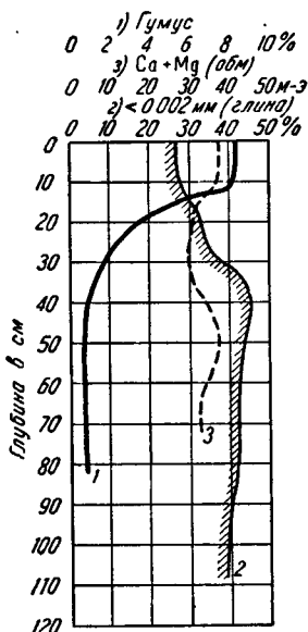
Фиг. 5. Кривые распределения гумуса, глинистой фракции и обменных оснований по профилю серых слабо оподзоленных почв лесостепи.
