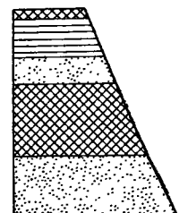
Фиг. 2. Разрез межледниковых отложений Микулино 1
