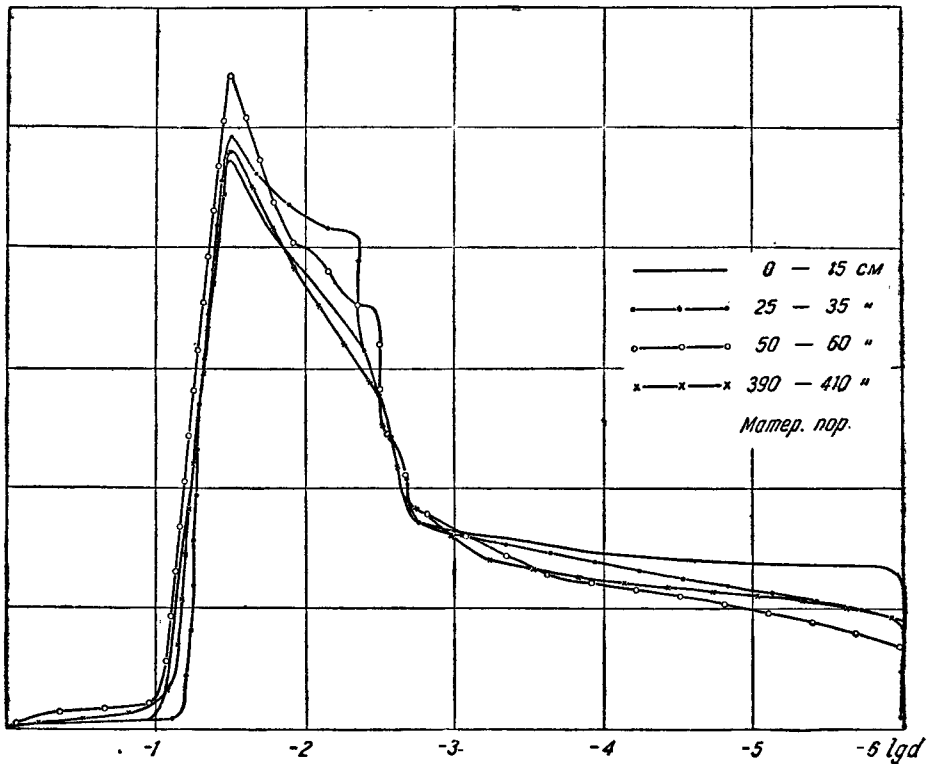
Фиг. 2. Кривые распределения механического состава темнокаштановой почвы.
