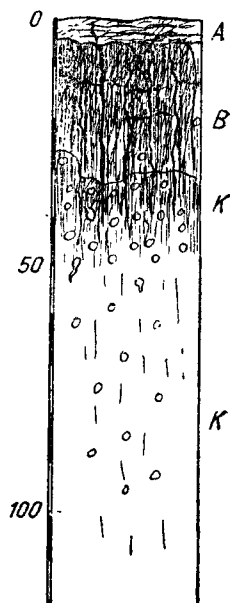
Фиг. 8. Солонец солончаковый содовый.
