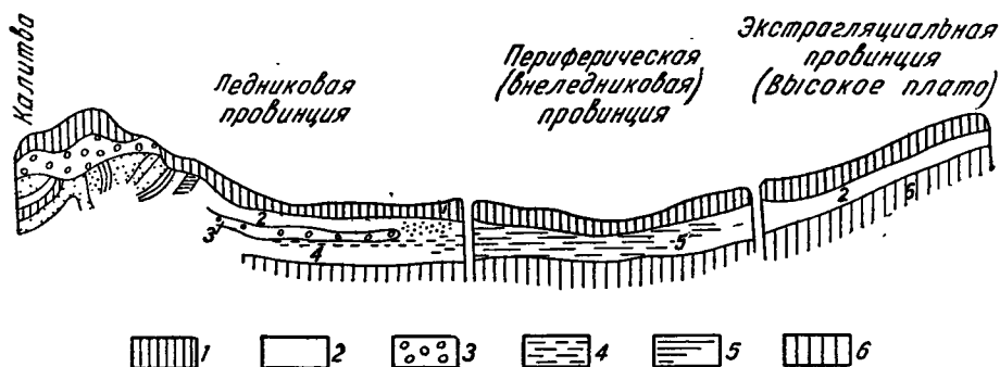
Фиг. 4. Схема соотношения морен и лёссовых ярусов в Днепровском языке 1 — Вюрмский лёс, 2 — Надморенная часть рисского лёса, 3 — Морена Днепровского оледенения, 4 — Подморенная часть рисского лёса, 5 — Пресноводная фация рисского лёса, 6 — Подрисская часть лёссовой свиты (из работы Л. Лундбергаузен «О четвертичных отложениях у границы Днепровского языка»)
