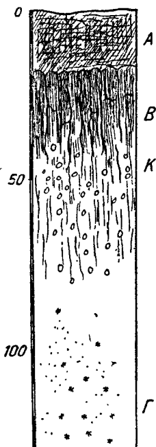
Фиг. 12. Солонец остаточно-слабосолончаковый.
