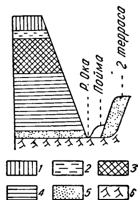
Фиг. 3. Разрез межледниковых отложений у гор Лихвина
