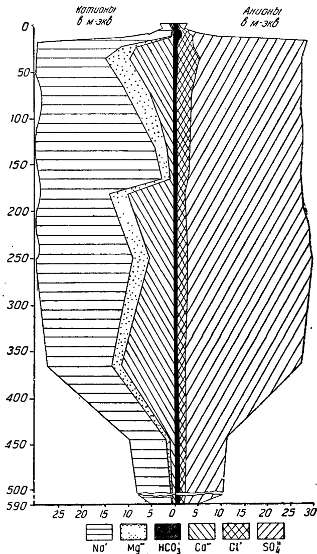
Фиг. 5. Солевой профиль хлоридно-сульфатного солонца.
