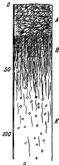
Фиг. 14. Солонец остепненный.
