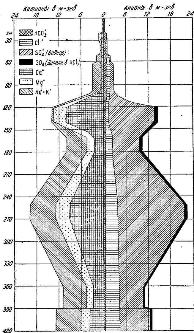
Фиг. 4. Разрез № 36 (Алтата). Солевой профиль.
