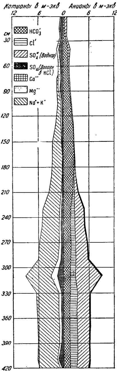
Фиг. 5. Разрез № 26 (Ершов). Солевой профиль.
