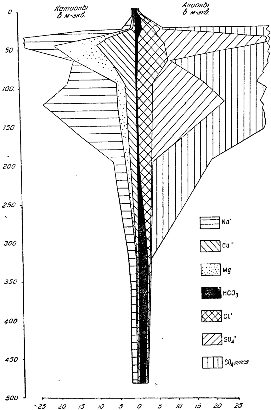
Фиг. 11. Солевой профиль остаточно-солончакового солонца.
