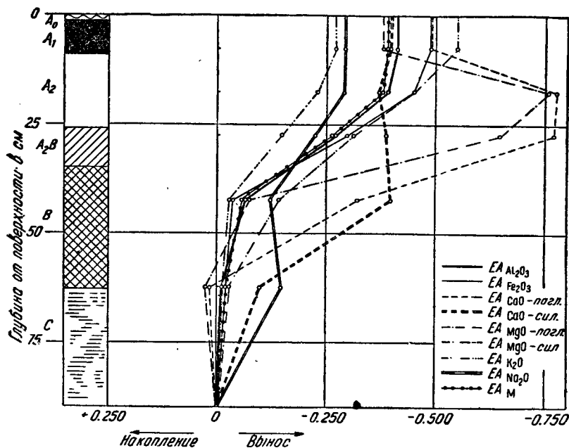
Фиг. 4. Изменения элювиально-аккумулятивных коэффициентов с глубиной в сильно подзолистой почве на ленточной глине № 3Р.
