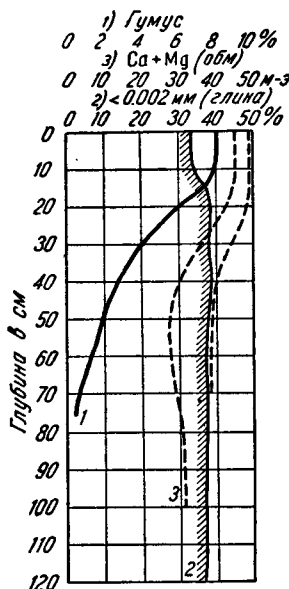
Фиг. 3. Кривые распределения гумуса, глинистой фракции и обменных оснований по профилю деградированных черноземов.
