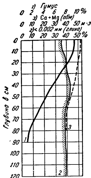
Фиг. 2. Кривые распределения гумуса, глинистой фракции и обменных оснований по профилю выщелоченных черноземов.
