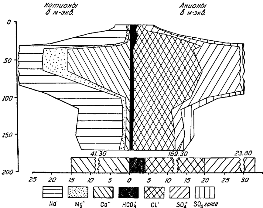
Фиг. 3. Солевой профиль сульфатно-хлоридного солончаковатого солонца.
