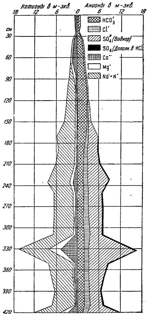
Фиг. 6. Разрез № 27 (Ершов). Солевой профиль.
