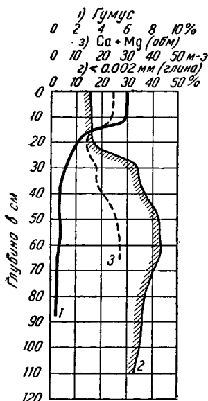
Фиг. 7. Кривые распределения гумуса, глинистой фракции и обменных оснований по профилю сильно подзолистой почвы лесной зоны (по данным А. А. Роде).
