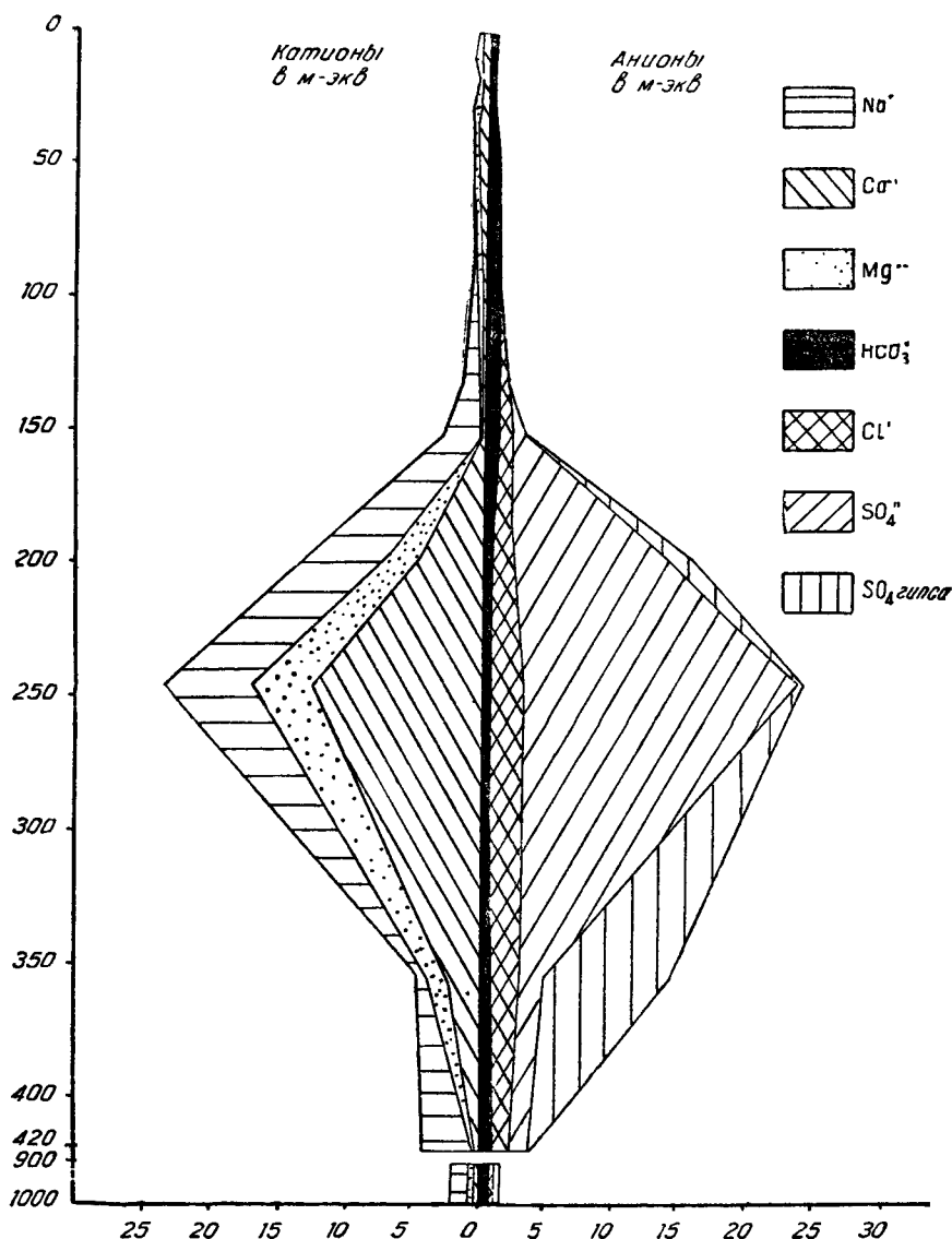
Фиг. 15. Солевой профиль остепненного солонча.
