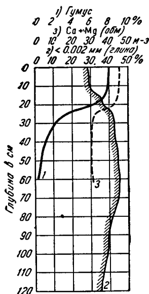
Фиг. 4. Кривые распределения гумуса, глинистой фракции и обменных оснований по профилю темносерых слабо оподзоленных почв лесостепи.
