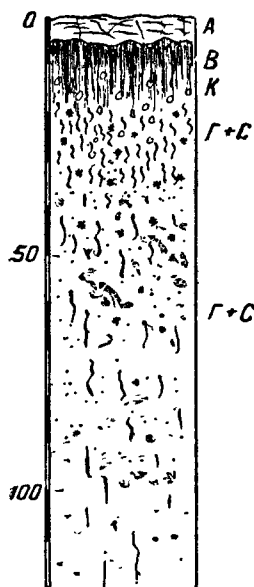
Фиг. 4. Солонец солончаковатый хлоридно-сульфатный.
