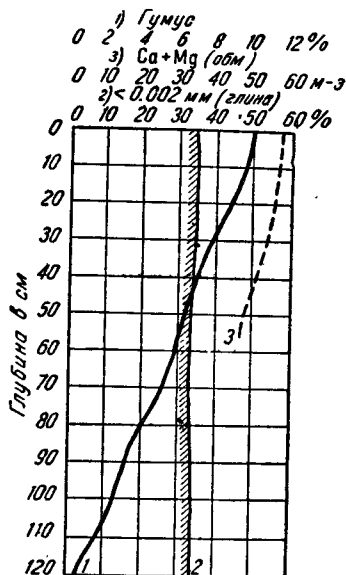
Фиг. 1. Кривые распределения гумуса, глинистой фракции и обменных оснований по профилю типичных мощных черноземов.
