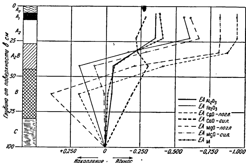
Фиг. 3. Изменение элювиально-аккумулятивных коэффициентов с глубиной в сильно подзолистой почве на ленточной глине № 95Р.
