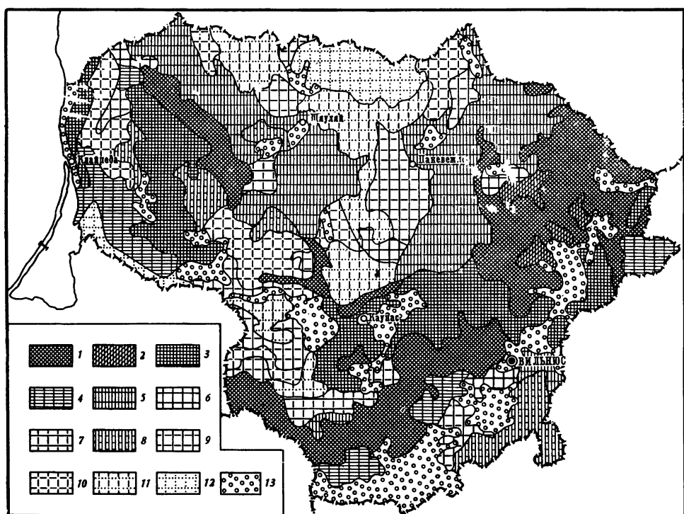
Рис. 2. Схема пестроты и контрастности почвенного покрова Литовской ССР
