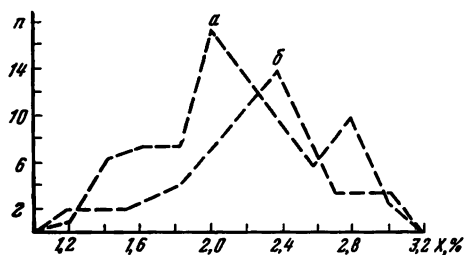
Рис. 3. Полигоны распределения содержания гумуса в пахотном горизонте дерново-подзолистых почв Смоленской области
