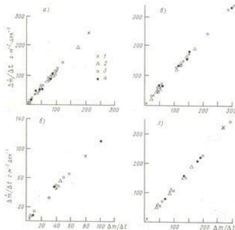
Рис. 5.1. Сравнение расчетных ( \Delta m/\Delta t ) и эмпирических ( \Delta m/\Delta t ) значений ( \text{г} \cdot \text{м}^{-2} \cdot \text{дек}^{-1} ) приростов биомассы отдельных органов растений за декаду. Озимая пшеница, сорт Мироновская 808; Подмосковье.
