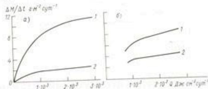
Рис. 6.1. Световые кривые продуктивности посева озимой пшеницы (сорт Мироновская 808) для разных условий подного (а) и теплового (б) режимов. Подмосковье.
