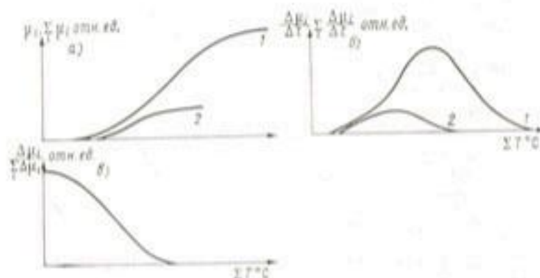
Рис. 4.2. Построение ростовой функции вегетативного периода i -го органа. а — кривые накопления биомассы, б — кривые скорости накопления биомассы, в — ростовая функция i -го органа; 1 — целое растение, 2 — i -й орган.
