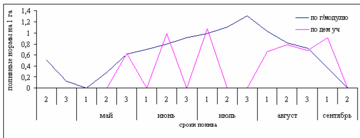
Рис. 30 Сравнительная оценка режима орошения по гидромульному районированию и по демонстрационному участку ф/х Сайед
