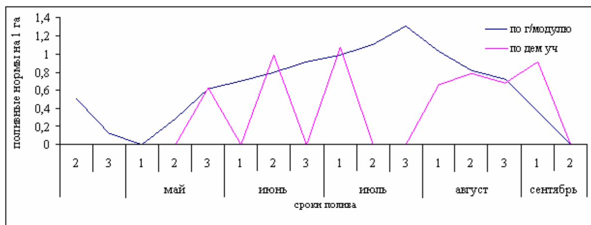
Рис. 31 Сравнительная оценка режима орошения по гидромульному районированию и по демонстрационному участку ф/х Нурсултан-Алы
