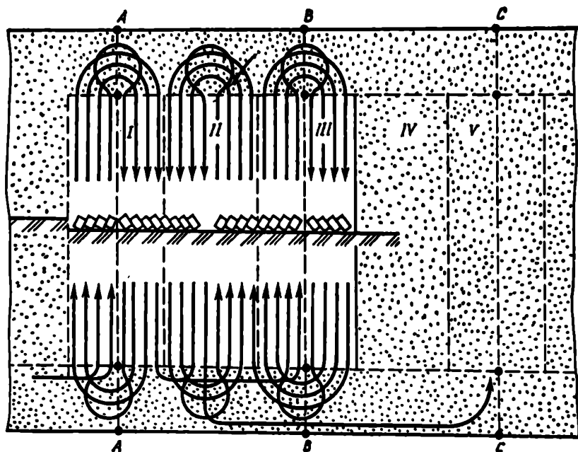
Рис. 8. Схема загональной вспашки с чередованием всвал и вразвал
