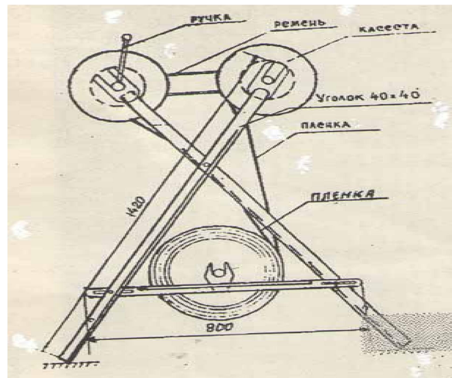
Рис 5 Лентоперематывающее устройство
