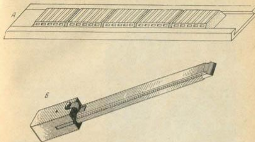
Рис. 1. Педоскоп Перфильева
