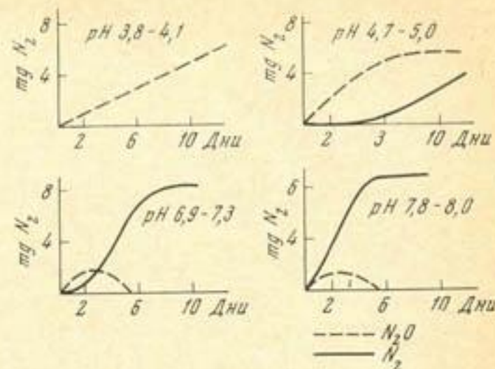
Рис. 81. Влияние реакции среды на образование \text{N}_2 и \text{N}_2\text{O} при денитрификации (по Е. Номмику)
