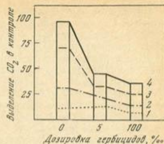
Рис. 73. Влияние разных дозировок трихлорбензойной кислоты на дыхание почвы (по П. Чандра)
