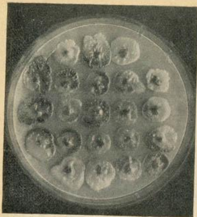
Рис. 35. Колонии Azotobacter chroococcum на твердой питательной среде, не содержащей азота
