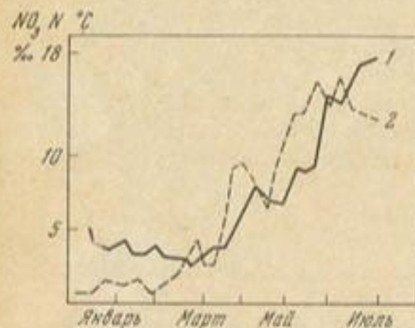
Рис. 49. Изменение температуры и накопление нитратов в почве в течение года (по В. Флайту)
