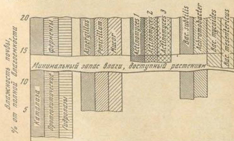
Рис. 47. Критические уровни влажности, прекращающие развитие растений, микроорганизмов и деятельность ферментов в почве
