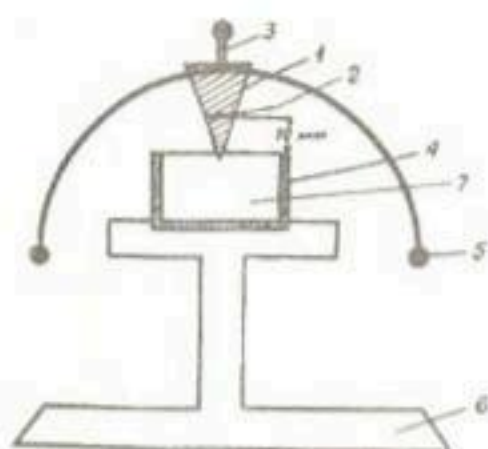
Рис. 13. Балансирный прибор (конус) А.М.Васильева. 1-конус; 2-круговая риска; 3-ручка; 4-формочка; 5-баланси́р; 6-деревянная подставка.
