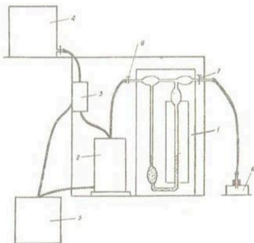
Рис.9. Схема прибора Н.Ф.Добрякова.
