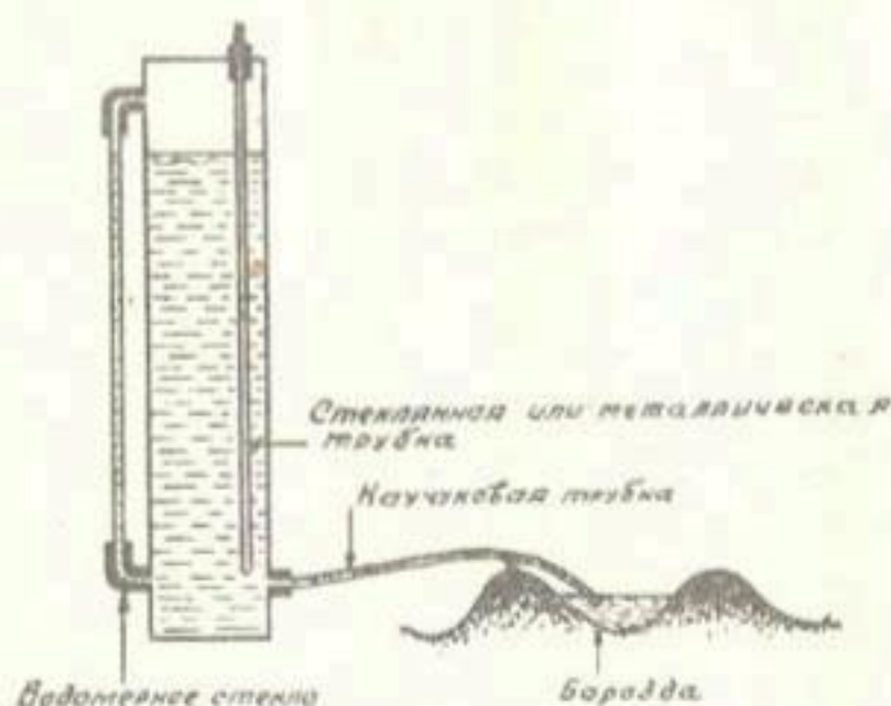
Рис. 8. Схема установки прибора для определения водопрооницаемости в бороздах.
