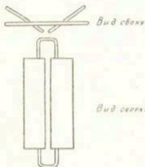
Рис. 3. Прибор Д.Г. Виленского для определения водопрочности комочков почвы.
