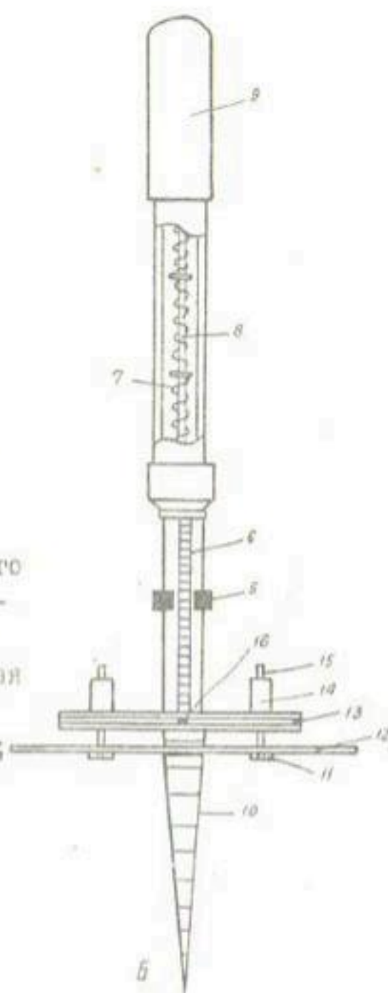
Рис. 14. Плотномер И.Ф.Голусова.
