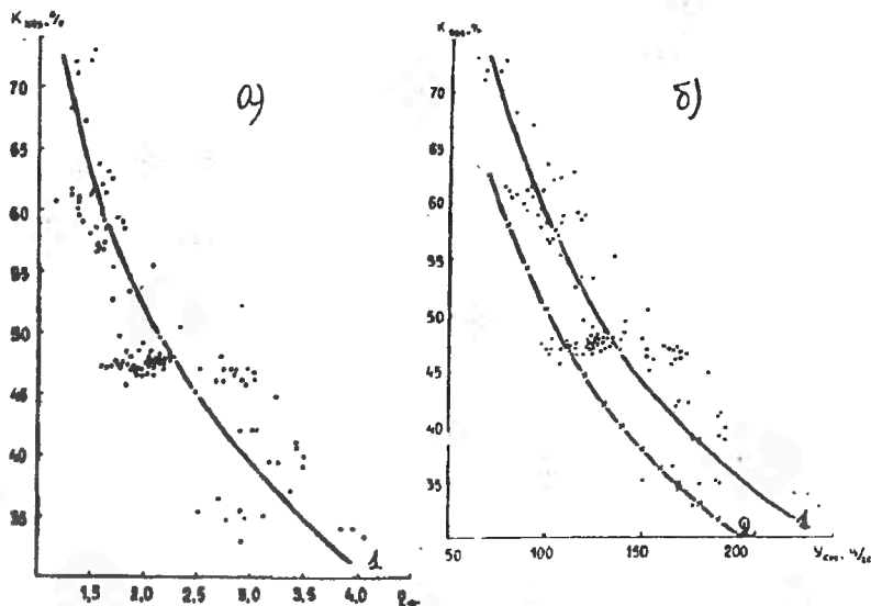
Рис. 11. Зависимость выхода зерна K_{хоз} (%) от: а) КПД посевов по приходящей ФАР \eta_Q (%), б) урожая сухой надземной биомассы 4 см ( ц/га ) на примере озимой пшеницы (1 — зерно при влажности 14 %, 2 — абсолютно сухое вещество).
