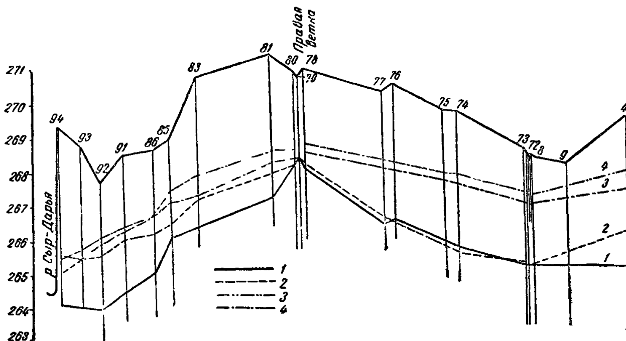
Рис. 34. Динамика уровня грунтовых вод в Присырдарьинской зоне в районе командования правой ветки Голодной Стени за период 1936—1937 гг.:
