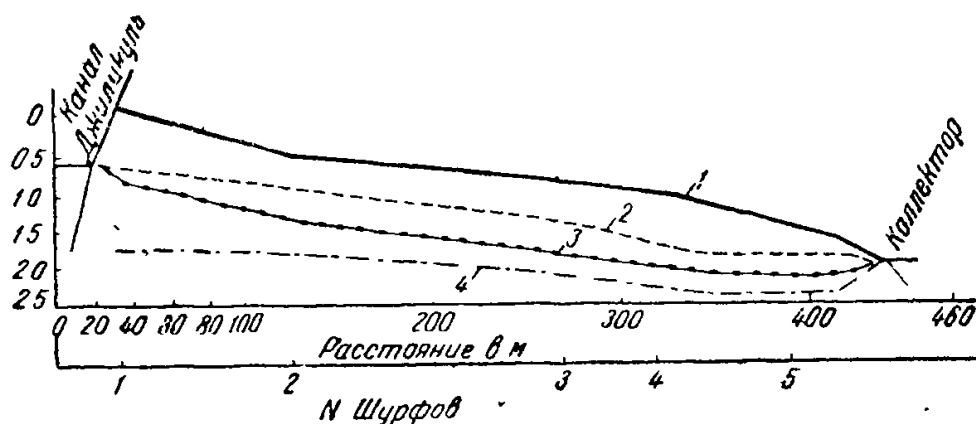
Рис. 9. Питающее влияние канала Джиликуль и коллектора на грунтовые воды в долине р. Вахш (Беспалов):
