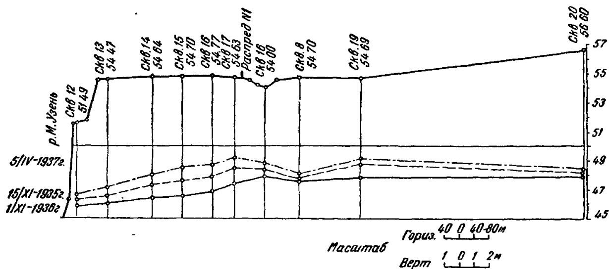
Рис. 17. Дренирующее значение р. М. Узень в ее верхнем и среднем течении. Малоузенский орошаемый участок (Савинов).
