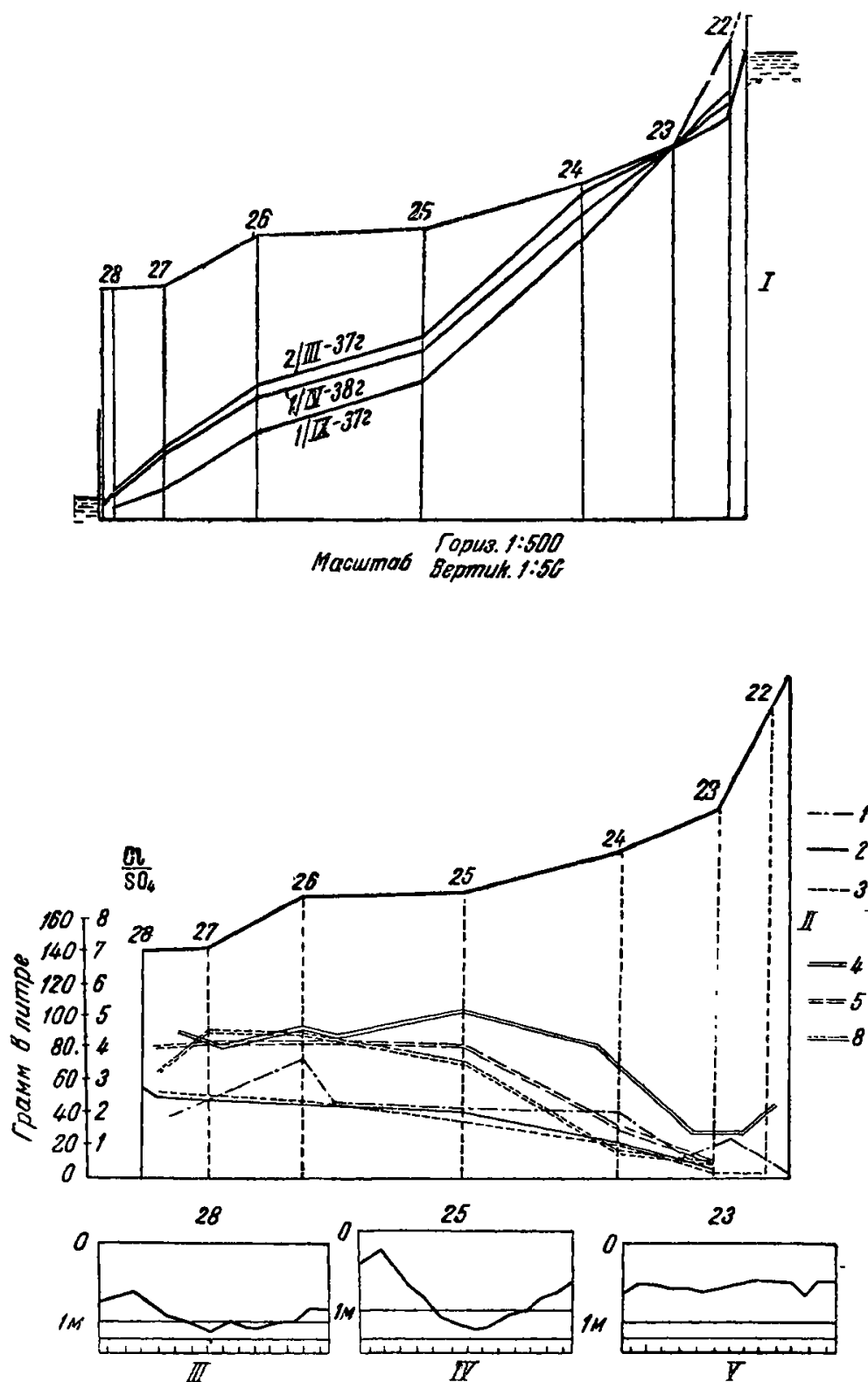
Рис. 23. Динамика уровня грунтовых вод и их минерализации в условиях интенсивного питания и оттока их (Вахш; Кераум и Грабовская):
