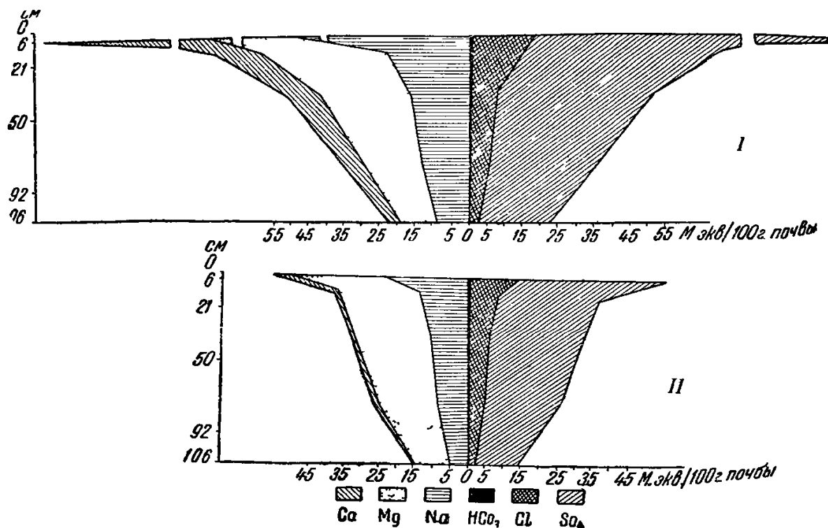
Рис. 21 Соотношение между содержанием солей в солончаках Ферганы
