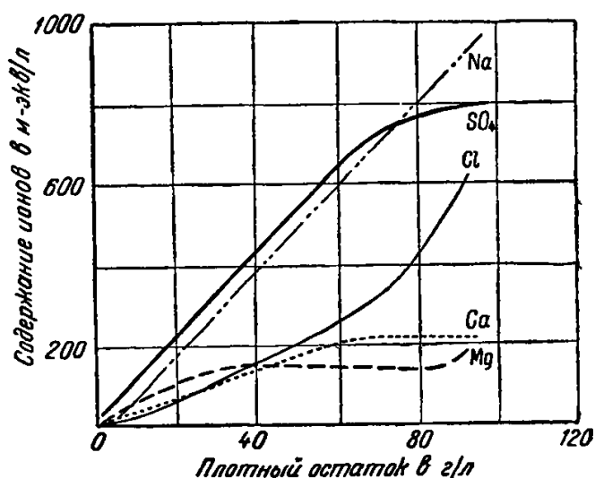
Рис. 12. Зависимость между минерализацией и составом грунтовых вод в Ферганской долине.
