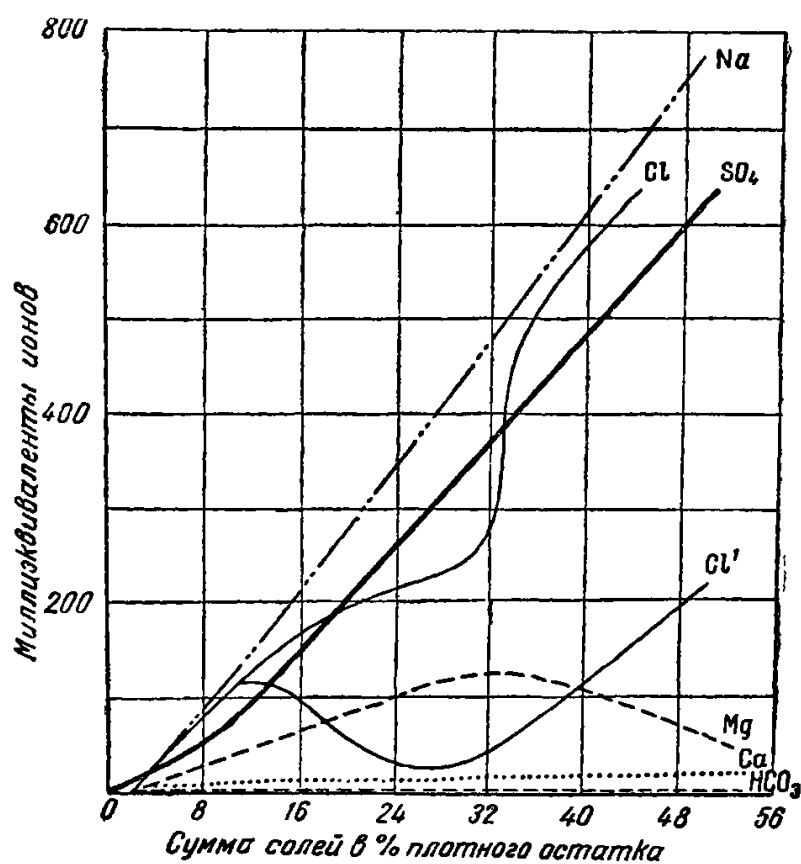
Рис. 37. Зависимость между степенью засоленности и составом солей в почвах низовьев р. Аму-Дарья.
