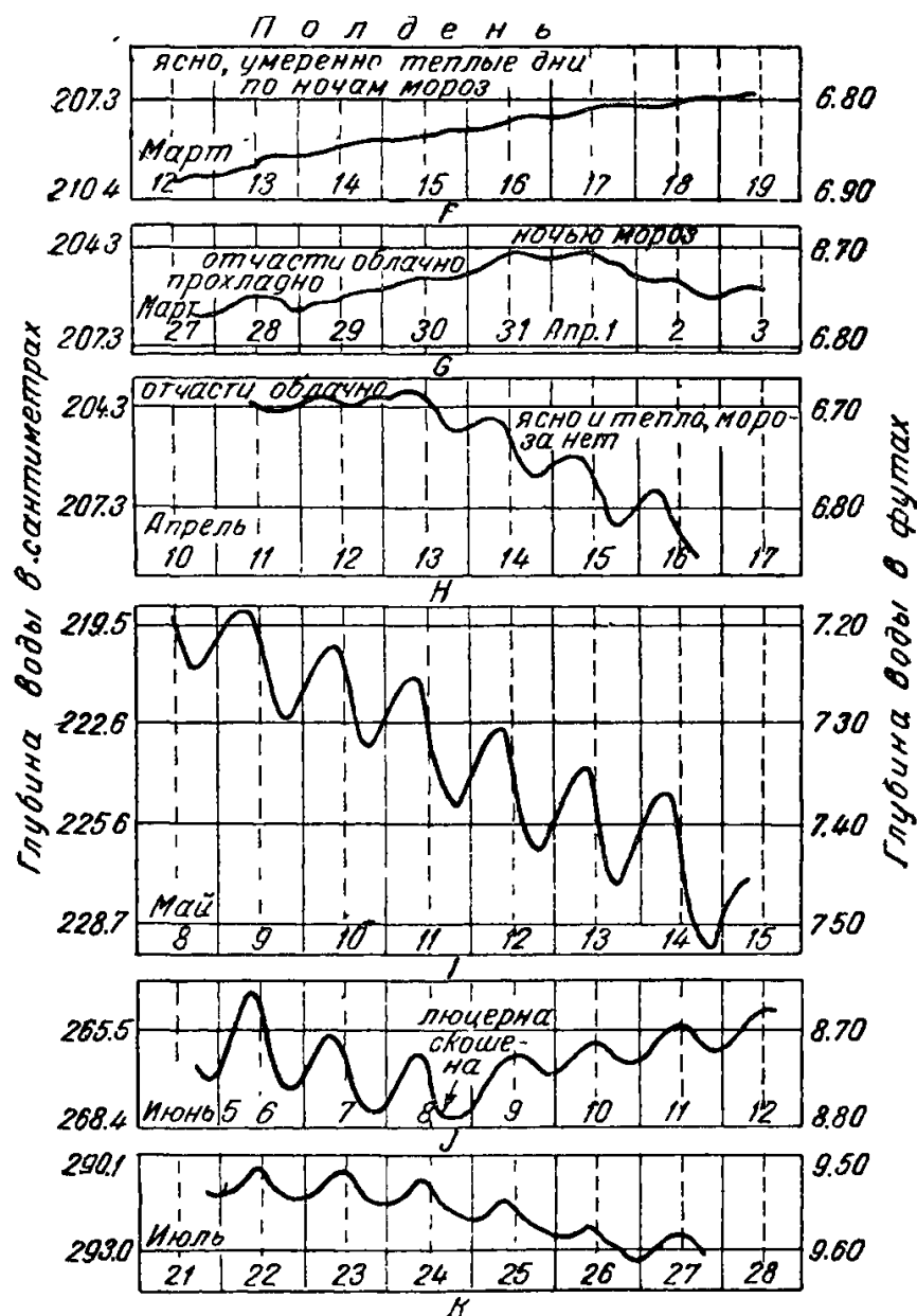
Рис. 16. Суточные колебания уровня грунтовых вод на полях люцерны в зависимости от различных условий (по Уайту).
