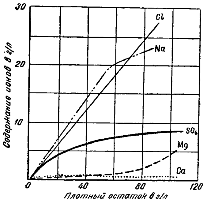
Рис. 7. Зависимость между минерализацией и составом грунтовых вод долины р. Вахш.
