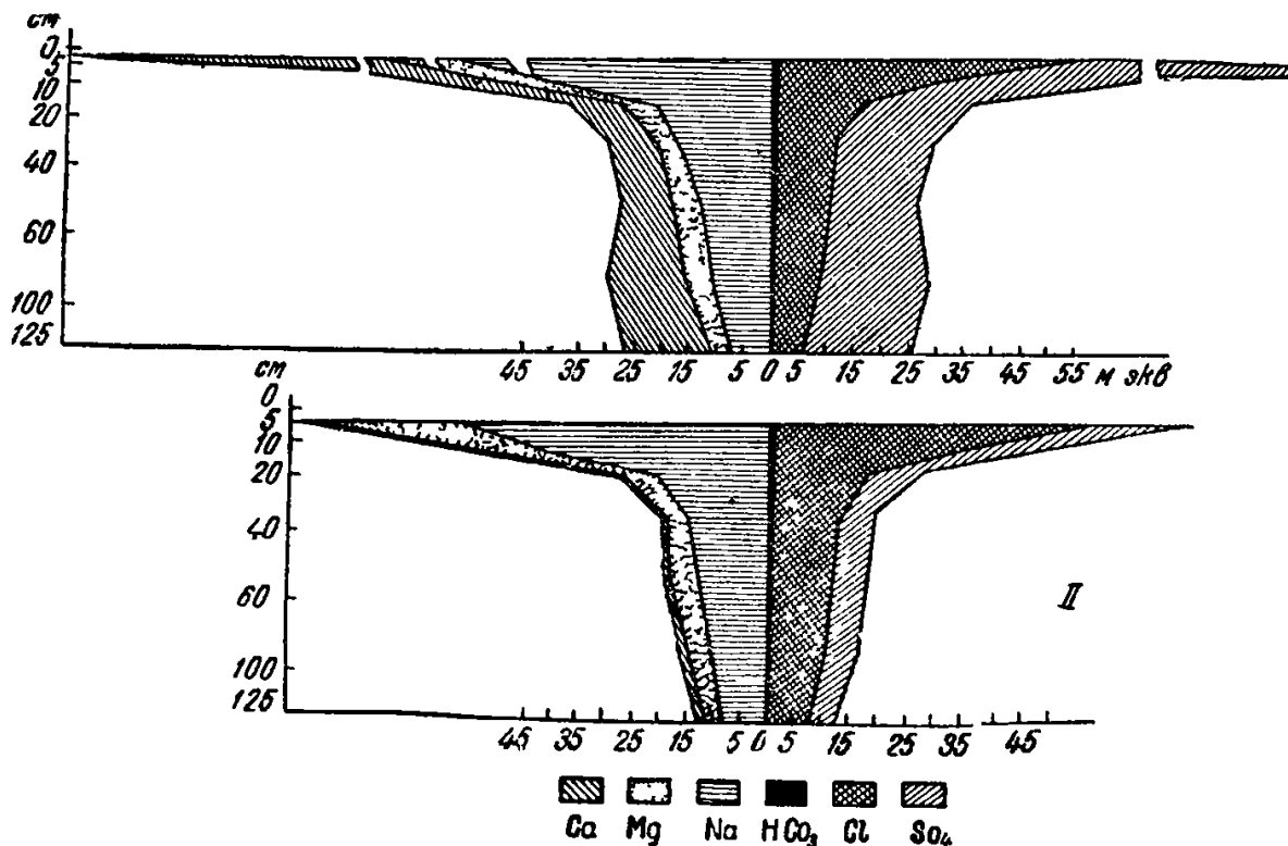
Рис 20. Соотношение между содержанием солей в солончаках Голодной Степи:
