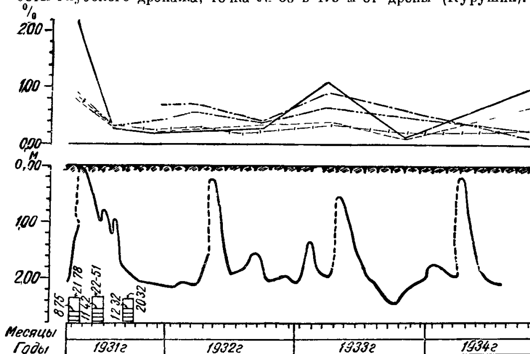
Рис. 44. Динамика солевого режима солончаков Мугани на фоне работы глубокого дренажа; точка № 38 в 175 м от дрены (Курушин).
