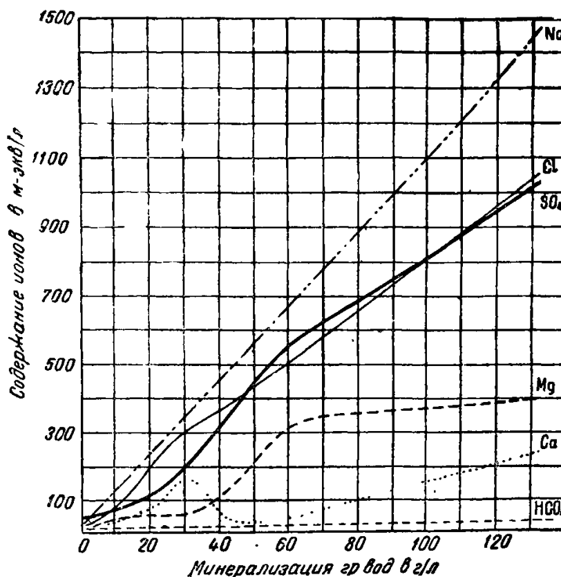
Рис. 13. Зависимость между минерализацией и составом грунтовых вод дельты Аму-Дарьи.
