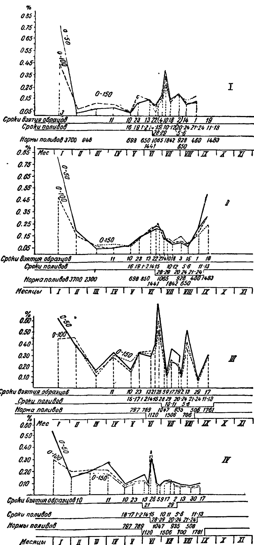
Рис. 42. Реставрация засоленности почв после промывки в зависимости от глубины грунтовых вод (Зайцев):
