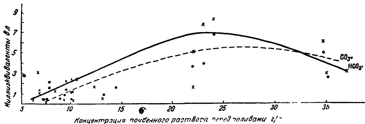
Рис. 27. Зависимость повышения щелочности почвенных растворов от концентрации перед поливами.
