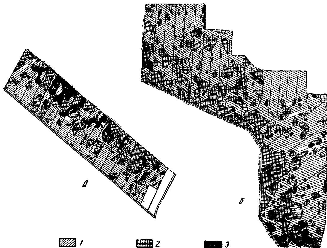
Рис. 51. Засоление почв вдоль ирригационных каналов в первые годы после начала орошения и рассоление их в последующем. (Данные Лебедева; Голодная Степь):
