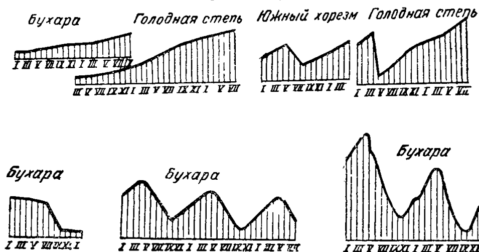
Рис. 22. Типы режима грунтовых вод орошаемых районов СССР (по Кенесарину).
