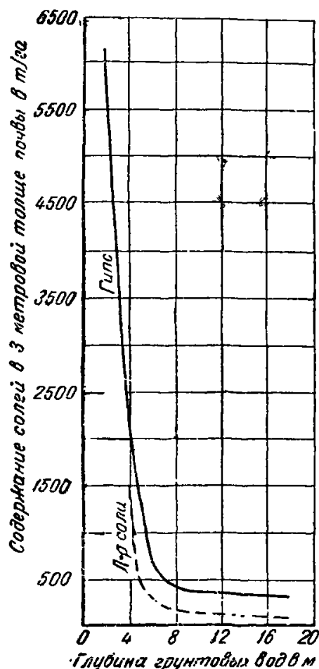
Рис. 30. Накопление легкорастворимых солей и гипса в грунтах и почвах Голодной Степи в зависимости от глубины грунтовых вод.
