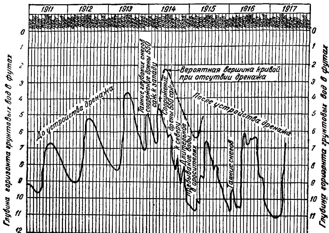
Рис. 36. Динамика уровня грунтовых вод до и после постройки дрена (по Дэвису)
