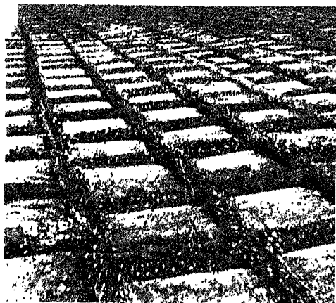
Снегозадержание риджер- ными снегопахами на по- лях Поволжья
