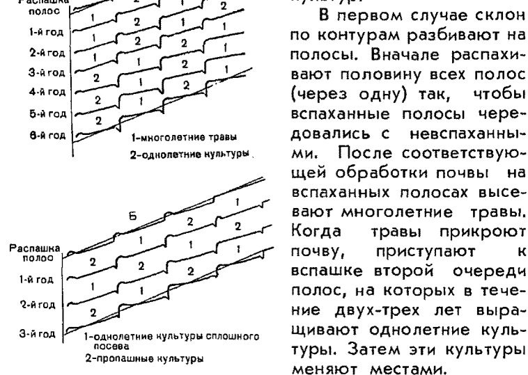
Рис. 15. Схема формирования напашных террас при чересполосном освоении склонов:
