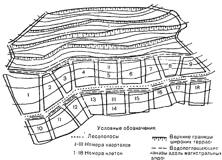
Рис. 17. Схема организации территории виноградника
