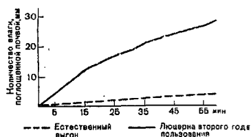
Рис. 13. Водопроницаемость почвы на естественном выгоне и под полосами люцерны второго года пользования
