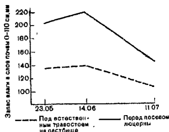
Рис. 12. Запас влаги в почве на вспаханных и невспаханных полосах в период освоения пастбищного склона
