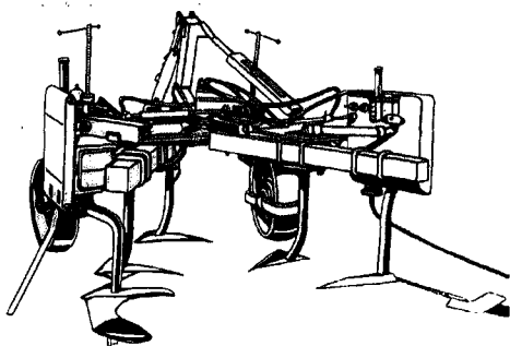
Приспособление к плугу ПРВМ-3 для междукустовой обработки почвы ПРВМ-1 1000. Предназначено для обработки почвы в ряду между кустами и в защитной зоне междурядья. Применяют на плодоносящих виноградниках на равнине и на склонах до 5^{\circ}
