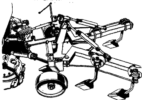
Плуг-рыхлитель виноградниковый универсальный ПРВМ-3. Навесной, предназначен для выполнения работ по культивации, сплошному рыхлению и вспашке междурядий виноградников в условиях равнины, на склонах до 5^{\circ} и террасах
