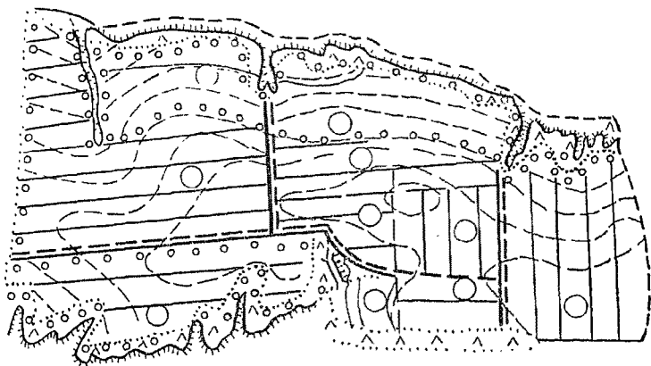
Р и с. 7. Организация пахотного массива прямолинейным способом в совхозе «Слава» Лебедянского района Липецкой области
