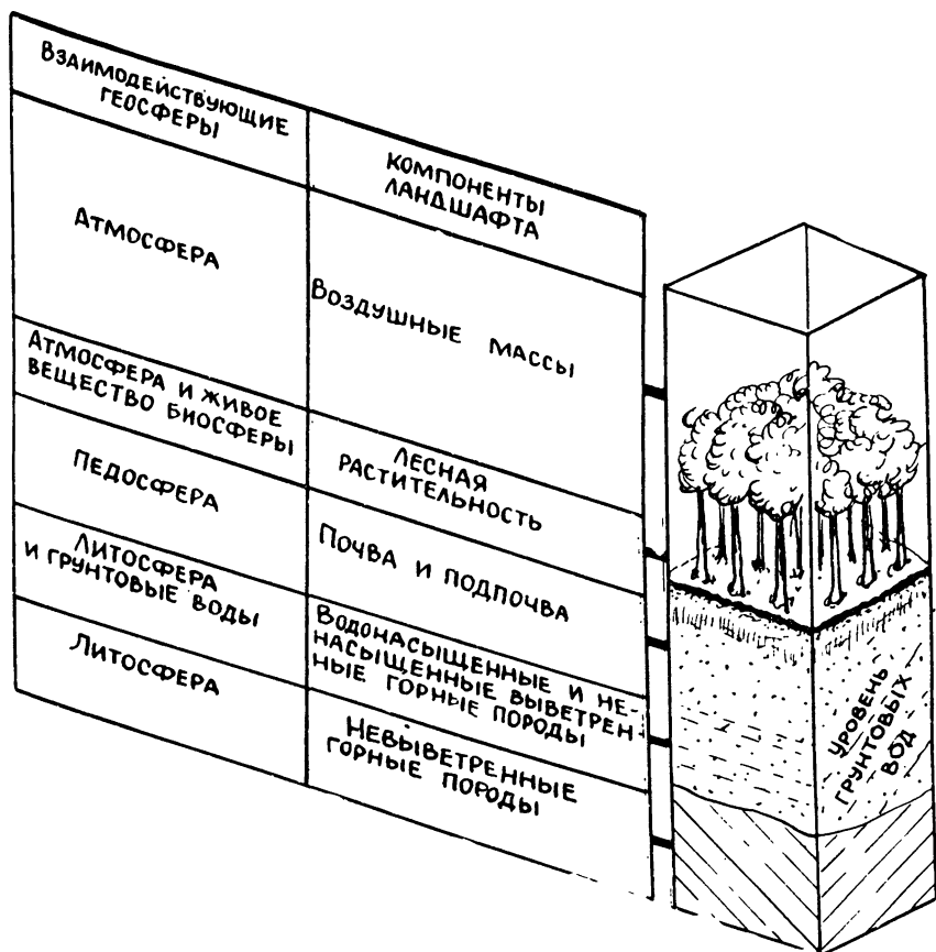
Рис. 2 Большая стратегическая ландшафтная призма, иллюстрирующая взаимосвязи геосфер и компонентов ландшафта в типичной лесной экосистеме (по Фортескью, 1982)
