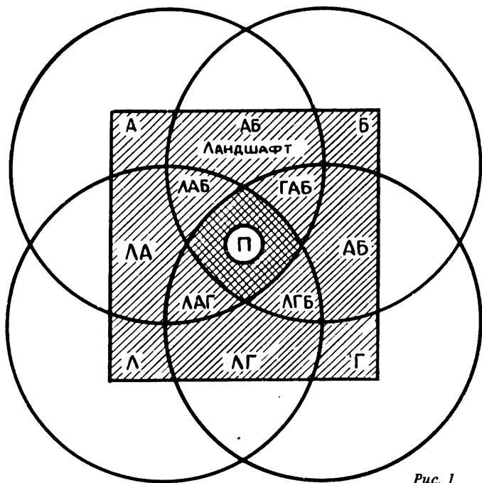
Рис. 1 Возможные взаимодействия между литосферой (Л), гидросферой (Г), атмосферой (А) и биосферой (Б). В результате этих взаимодействий образуется "педосфера" (П) как элемент "ландшафта" (по Mattson, 1938, с изменениями)
