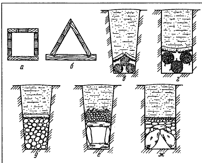
Рис. 29. Виды деревянного и каменного дренажей, выполненных вручную: а, б — деревянные дощатые дренажи; в — железная дренаж; г — фашинная дренаж; д, е, ж — каменные дренажи.
