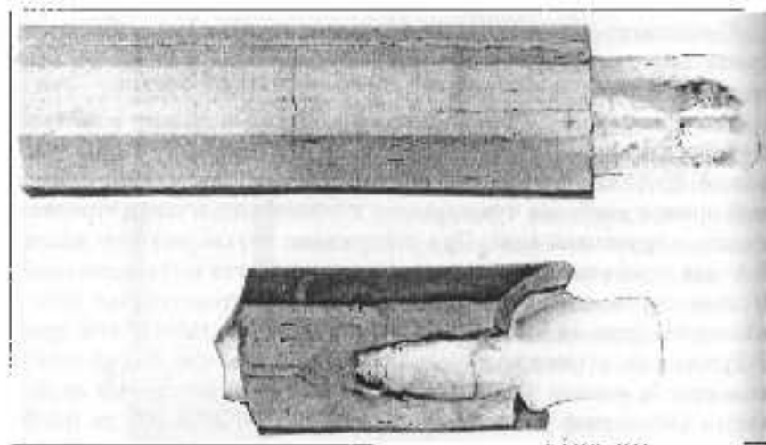
Рис. 32. Закупорки и разрушение керамической дренажа ледяными пробками. Бухаринская низменность, Западная Сибирь (фото Н. И. Логина)
