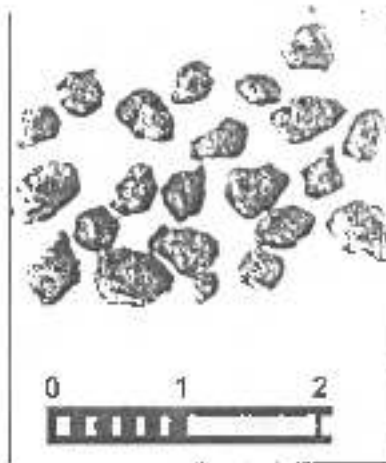
Рис. 11. Бурые железистые ортштейны из гор. A2q дерново-подзолистых суслистых глеевых почв
