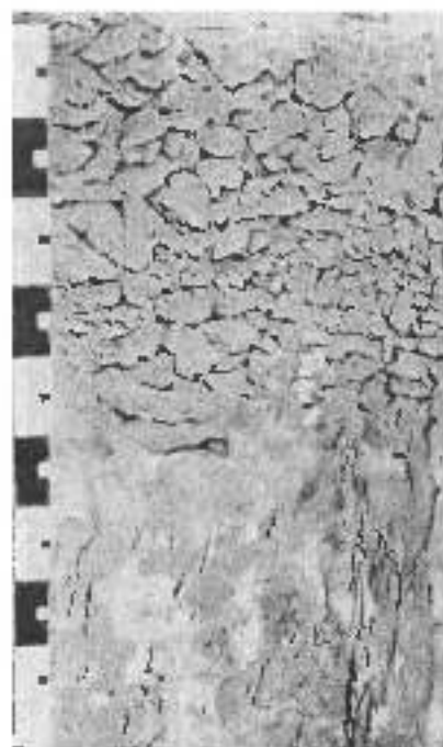
Рис. 8. Железистые коры в профиле луговых сильноокисленных глеевых почв. Окско-Метцерское поле
