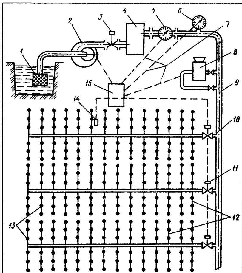
Рис. 48. Система капельного орошения (схема): 1, 2 — водозаборный и напоробразующий узлы; 3 — головная задвижка; 4 — фильтр; 5 — водомерное устройство; 6 — манометр; 7 — канал связи; 8 — устройство для подачи удобрений в поливную сеть; 9 — магистральный трубопровод; 10 — распределительный трубопровод; 11 — дистанционно управляемая задвижка; 12 — поливные трубопроводы; 13 — капельницы; 14 — датчики необходимости полива; 15 — пульт управления
