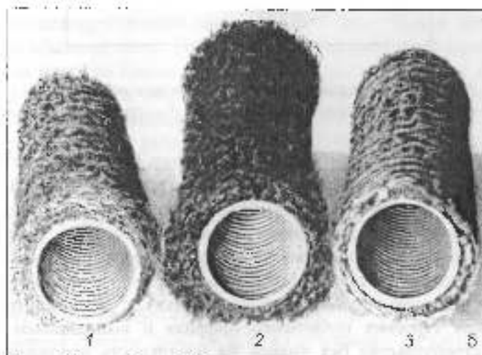
Рис. 27, а — трубчатые перифитесные и б — пластмассовые дренажи с объемными фильтрами из коксового волокна (1), торфа (2) и соломы (3)
