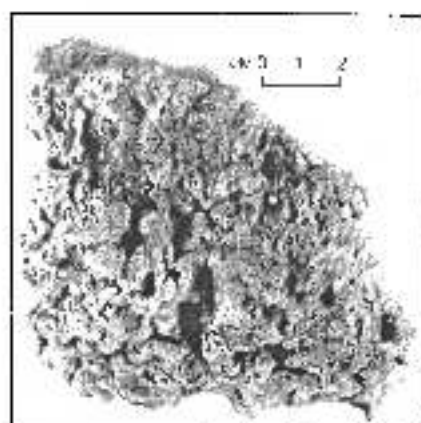
Рис. 7. Рудяковый панцирь (рудяк отделился) из дерново-слабоподзолистой глеевой рудяковой почвы, заболоченной сильно-омежеванными грунтовыми водами. Окстэ-Мещерские поляны
