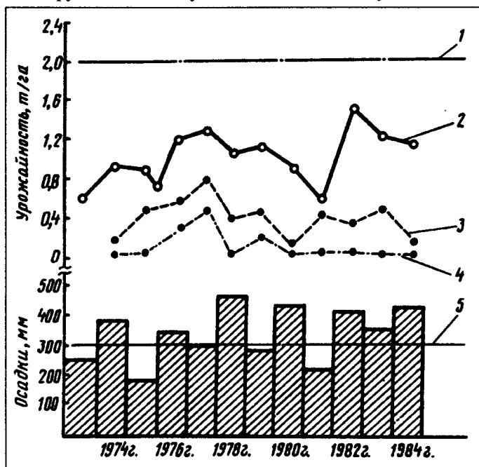
Рис. 20. Влияние степени заболоченности почв на урожай зерновых культур. Средняя урожайность по хозяйствам на незаболоченных и заболоченных почвах: 1 — проектная; 2 — реальная средняя урожайность на дренированных; 3 — дерново-глееватых; 4 — дерново-глеевых почвах; 5 — средняя многолетняя сумма осадков за теплый период (май-сентябрь). Кировская область
