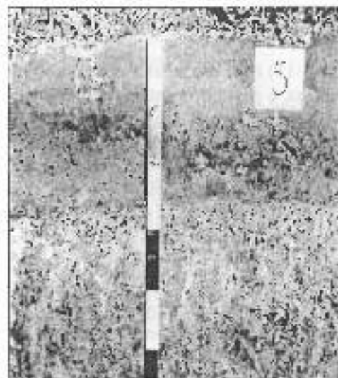
Рис. 10. Темно-серые марганцево-железистые ортштейны из гор. A2 дерново-подзолистых суслистых неглеевых почв
