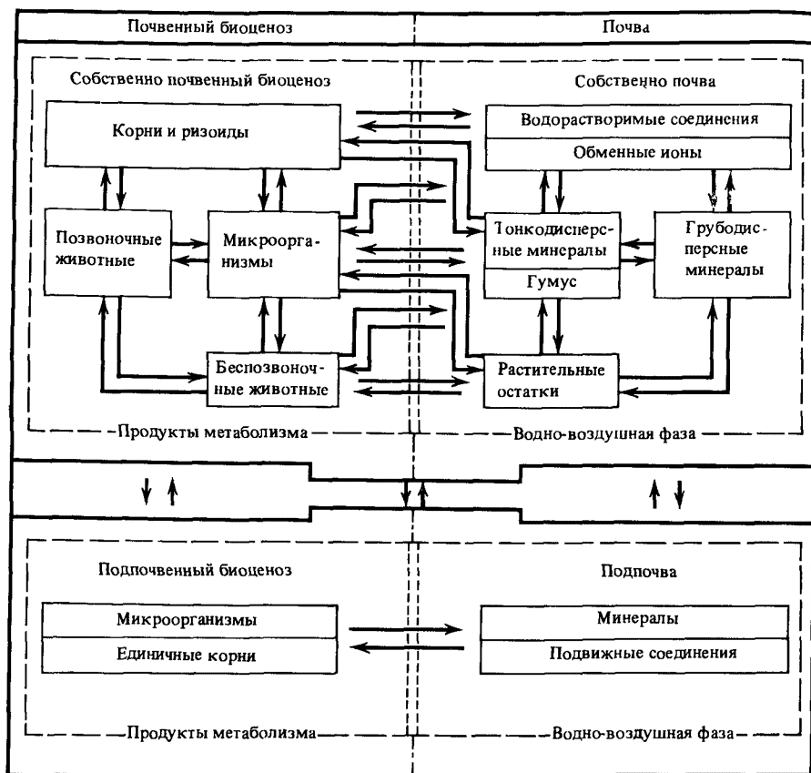
Структурная модель педосистемы (биопедоценоза)
