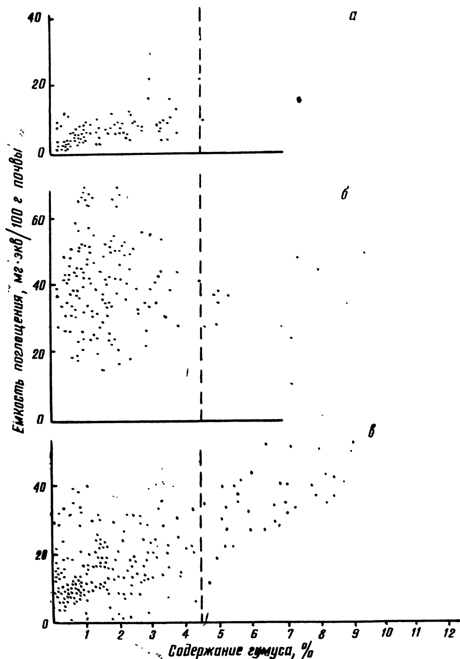
Рис. 38. Распределение отметок образцов почв по величине емкости поглощения при разном содержании гумуса для групп почв основных минеральных фаз: а—сиаллитная; б—глинная; в—ферраллитная.
