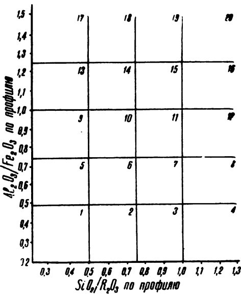
Рис. 26. График для кодирования почв по изменению отношений SiO_2/R_2O_3 и Al_2O_3/Fe_2O_3 в профиле
