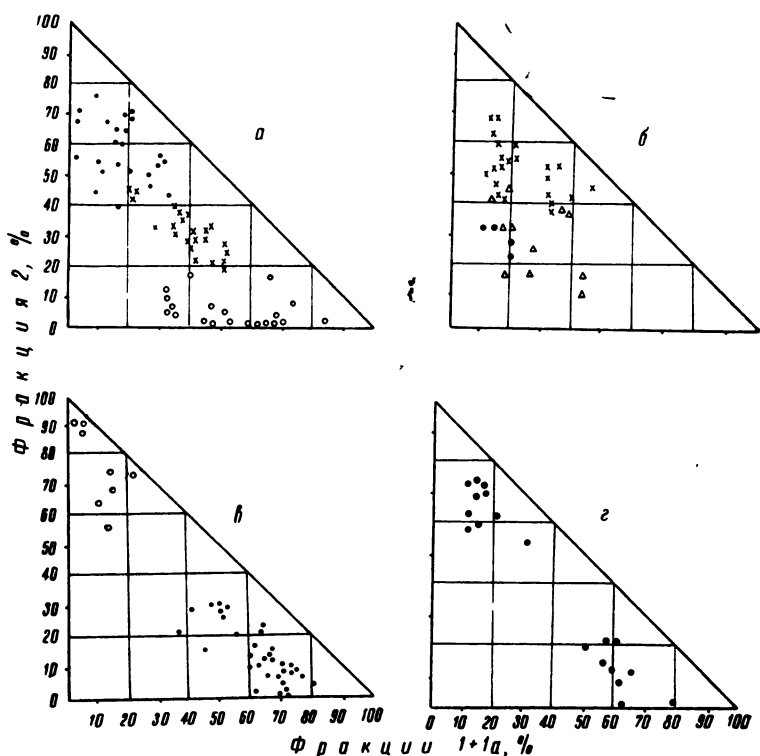
Рис 29. Распределение отметок фракционного состава гумуса некоторых характерных типов почв.
