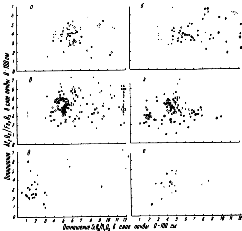
Рис. 24. Распределение отметок по величине отношений SiO_2/R_2O_3 и Al_2O_3/Fe_2O_3 в слое 0—100 см.
