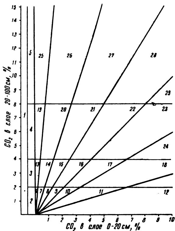
Рис 19. График для кодирования почв по содержанию \text{CO}_2
