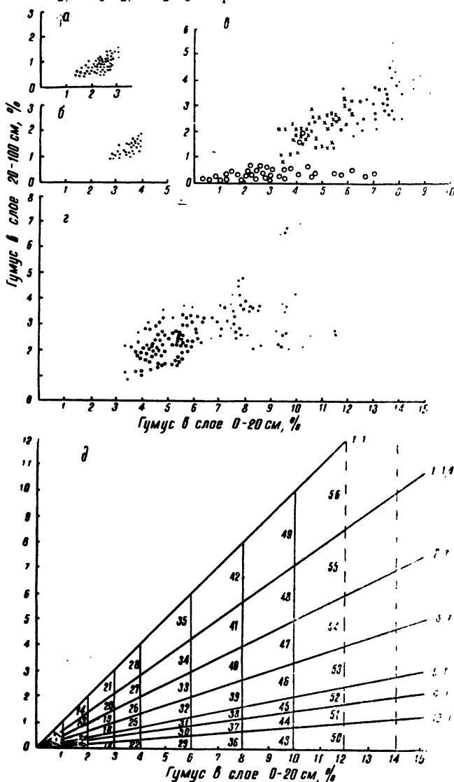
Рис. 14. Распределение отметок содержания гумуса в почвах в слоях 0—20 и 20—100 см и кодовый график по гумусу а—каштановые; б—темно-каштановые; в—черноземы: южные (X), обыкновенные (●), дерново-подзолистые (○); г—все черноземы (учтенные при обработке); д—график для кодирования почв по содержанию гумуса в слоях 0—20 и 20—100 см (номера кода проставлены на поле графика—1—56), справа указаны величины соотношения в содержании гумуса в слоях 0—20 и 20—100 см
