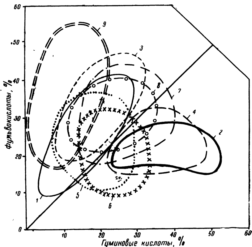
Рис. 3. Распределение отметок группового состава гумуса некоторых характерных типов почв по полю трехвекторного графика: гуминовые кислоты—фульвокислоты—все другие компоненты группового состава (негидролизующий остаток, воскосмолы и др.) (в % от общего углерода гумуса)
