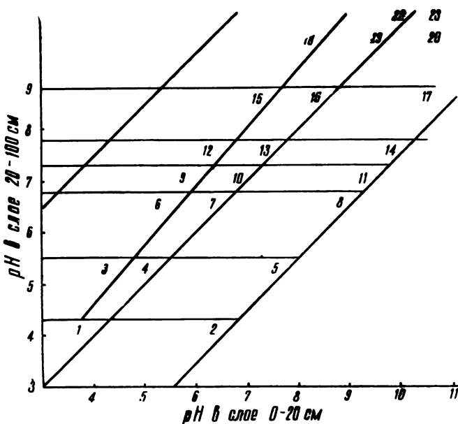
Рис. 21. График для кодирования почв по величине рН в слоях 0—20 и 20—100 см
