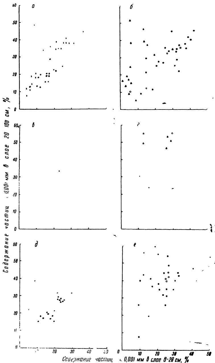
Рис. 22. Распределение отметок почв по содержанию частиц < 0,001 мм в слоях 0—20 и 20—100 см:
