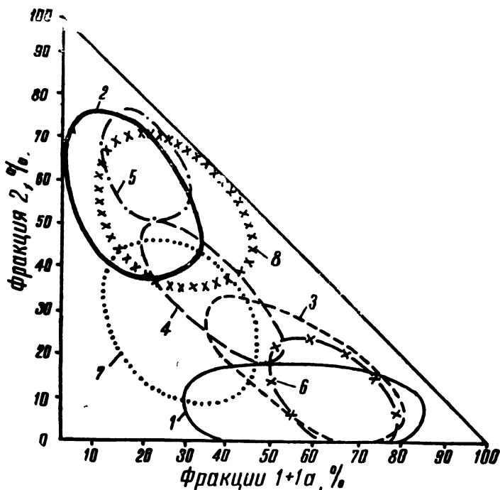
Рис. 4. Распределение отметок фракционного состава гумуса некоторых характерных типов почв по полю трехвекторного графика: сумма фр. 1+1а—фр. 2—фр. 3+гидролизат (в % от общего углерода гумуса)
