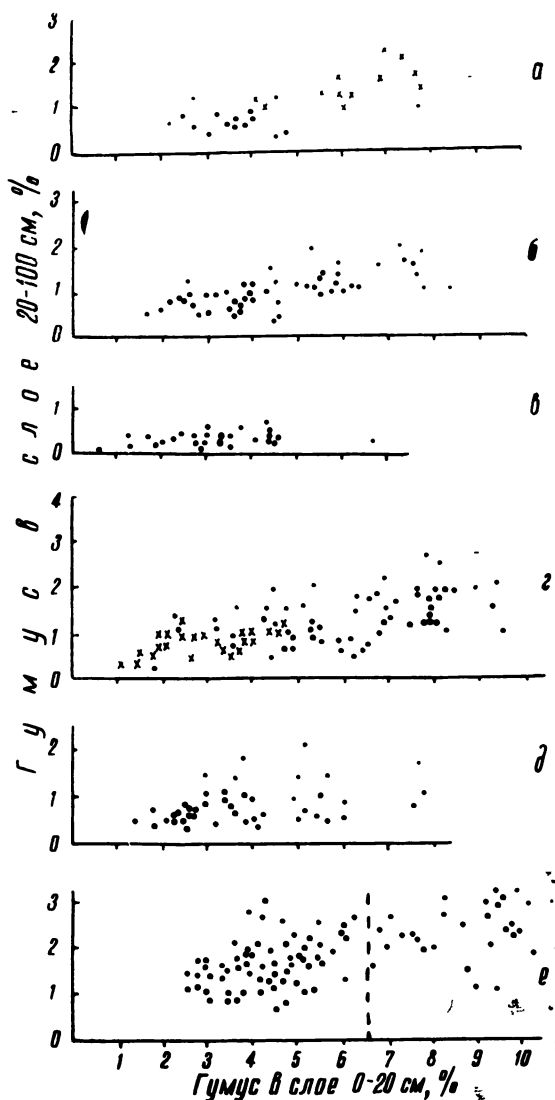
Рис 16. Распределение отметок содержания гумуса в почвах в слоях 0—20 и 20—100 см
