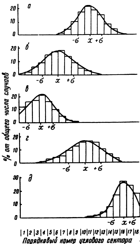
Рис. 30. Кривые распределения почв по градициям отношений Гк/Фк и фр. 1+1а/2 (столбики — исходные данные, линии — вычисленные кривые). \bar{x} — средние значения; \sigma — квадратические отклонения: а, б — с преобладанием в групповом составе соответственно гуминовых и фульвокислот; в — с преобладанием во фракционном составе фр. 2; г — с относительно равным содержанием фр. 2 и 1+1а; д — с преобладанием фр. 1+1а
