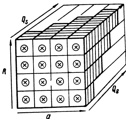
Рис. 13. Энергетическая схема системы почв
