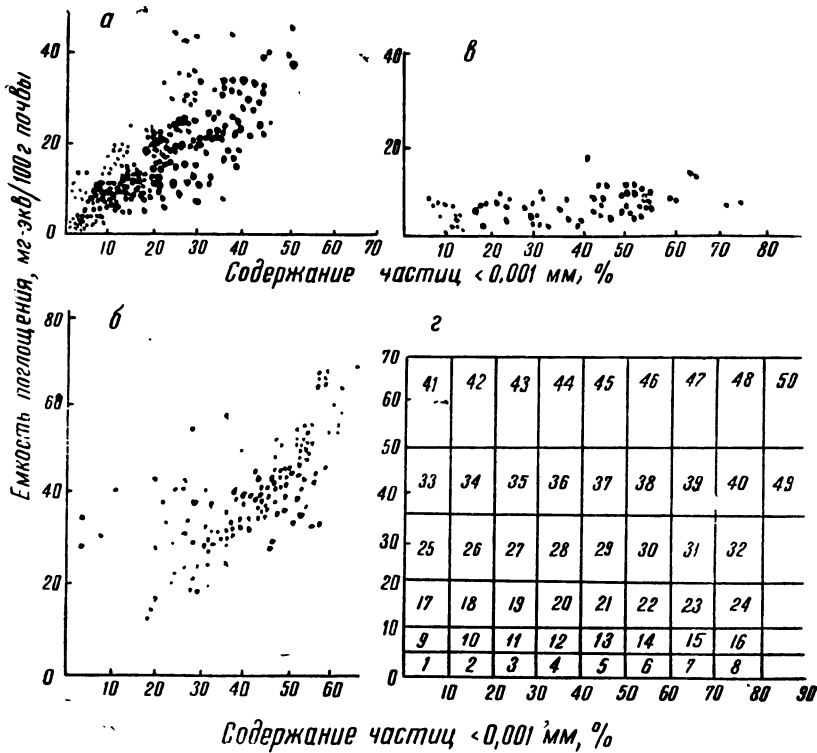
Рис. 39. Распределение отметок образцов почв с содержанием гумуса менее 4,0% в связи с содержанием частиц <0,001 мм по группам основных минеральных фаз:
