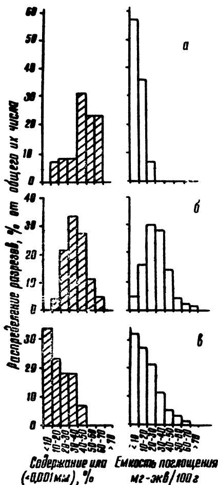
Рис. 8. Распределение разрезов по степени иллитности и емкости поглощения по каждой из трех групп почв согласно значениям отношения \text{SiO}_2/\text{R}_2\text{O}_3 а— <3,5 ; б— 3,5-5,5 ; в— >5,5
