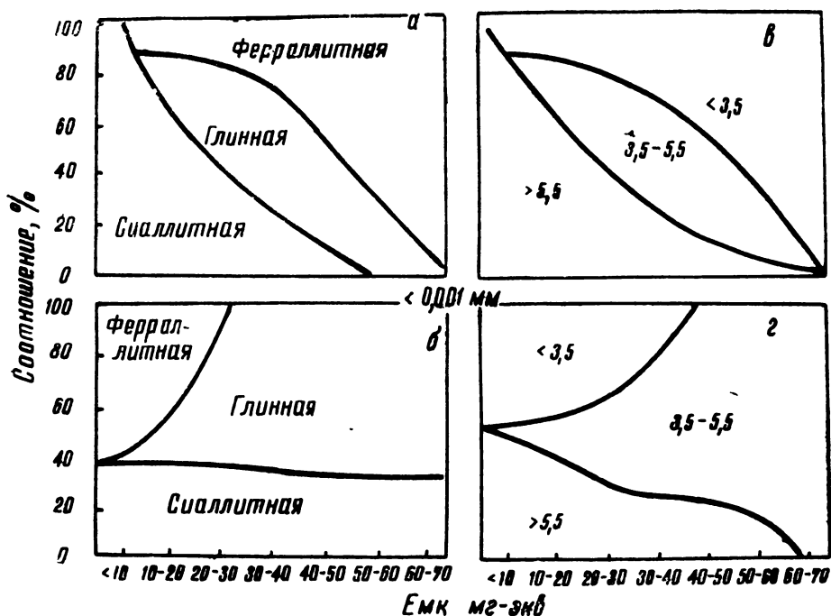
Рис. 37. Изменение вероятного соотношения почв разных фаз минеральных преобразований при разном содержании частиц <0,001 мм и величине емкости поглощения. Графики а и б получены при обобщении по соответствующим группам типов почв, в и г — при обобщении по группам почв, подразделенным по значениям отношения \text{SiO}_2/\text{R}_2\text{O}_3 ( <3,5 ; 3,5-5,5 ; >5,5 )
