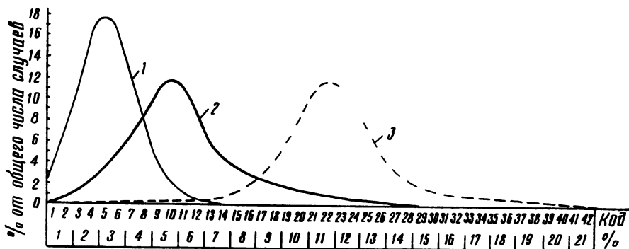
Рис. 36. Кривые распределения числа случаев почвенных образцов с разным содержанием гидратной воды (%) в почвах установленных фаз минеральных преобразований: 1—сиаллитная; 2—глинная; 3—ферраллитная
