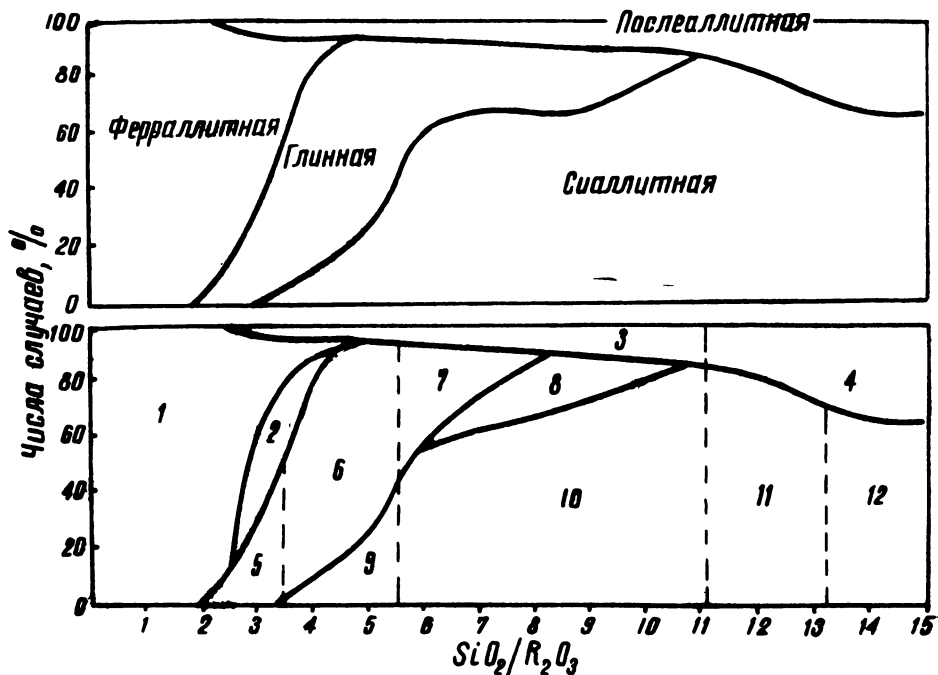
Рис. 34. Изменение вероятного соотношения между минеральными фазами в почвах при разных значениях: \text{SiO}_2/\text{R}_2\text{O}_3
