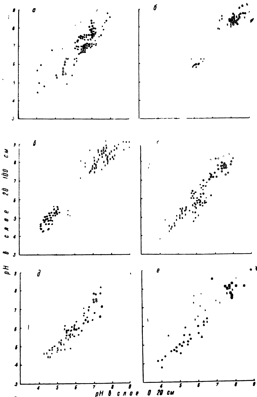
Рис. 20. Распределение отметок pH почв в слоях 0—20 и 20—100 см а—черноземы карбонатные и южные (○), выщелоченные и оподзоленные (×), все другие, в том числе с неуказанным подтипом (● тундровые почвы без подразделения (△); б—сероземы (×), серые лесные (●), пустынные почвы США (○); в—каштановые (×), дерново-подзолистые и подзолы (●); г—коричневые (○), желтоземы (●), красноземы субтропические (×); д—бурые лесные: остаточные карбонатные (○), оподзоленные (×), все другие, в том числе с неуказанным подтипом (●); е—красные влажнотропические (●), желтые влажнотропические (○), опесчаненные влажнотропические (△), смолницы и грумосоли (США) (×), черные тропические (■)
