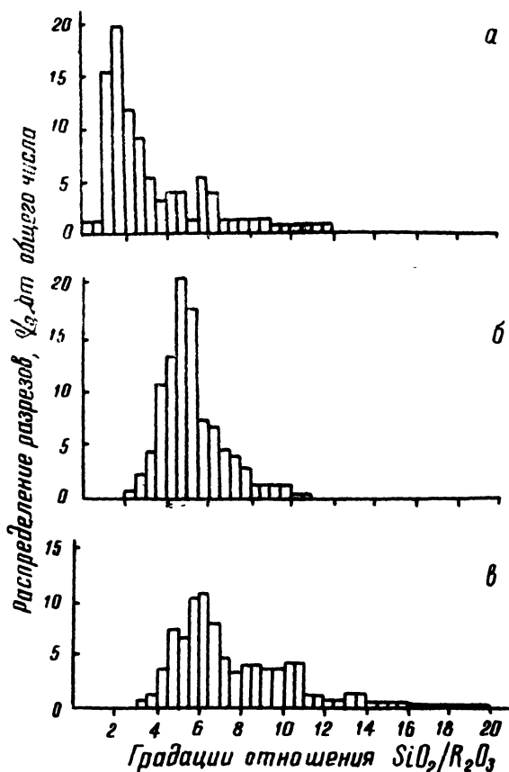
Рис. 7. Распределение почв по величине отношения \text{SiO}_2/\text{R}_2\text{O}_3
