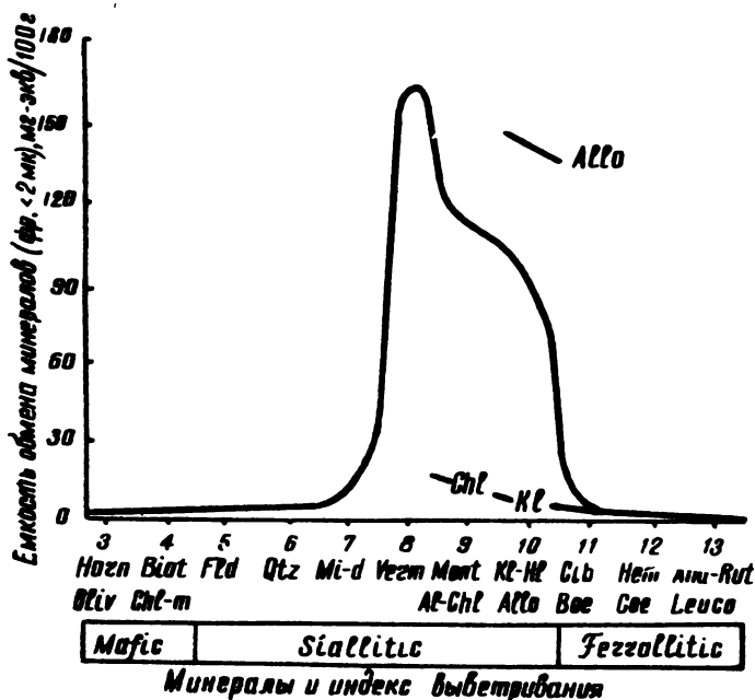
Рис. 9 Величина обменной способности фракции <0,002 мм различных классов минералов с разными номерами индекса выветривания (по Jackson, 1968)
