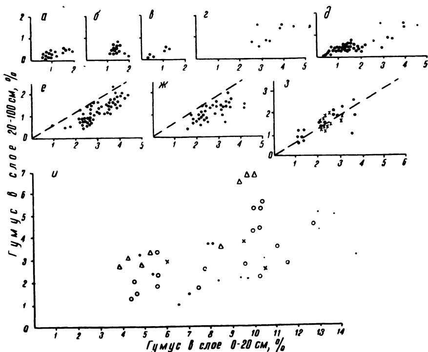
Рис. 15. Распределение отметок содержания гумуса в почвах в слоях 0—20 и 20—100 см
