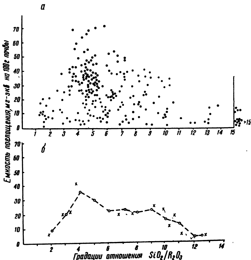
Рис. 6. Изменение емкости поглощения в слое почвы 0—50 (60) см в связи со значением отношения \text{SiO}_2/\text{R}_2\text{O}_3 в слое почвы 0—100 см по почвам Еязии (степные, таежнолесные, субтропические, тропические и др.)
