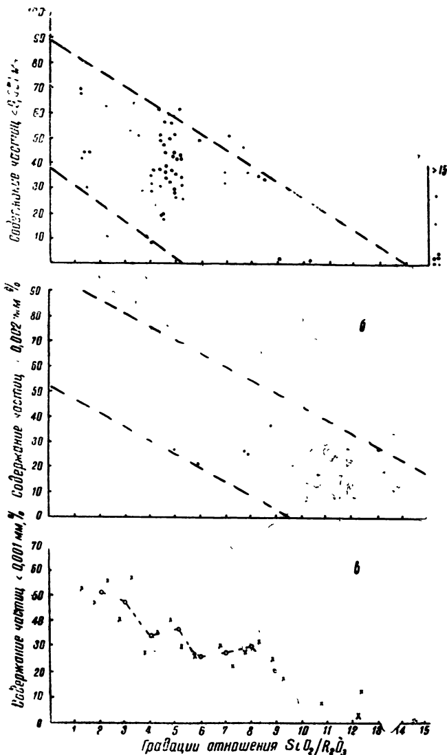
Рис 5. Изменение содержания илистых частиц в связи с значением отношения SiO_2/R_2O_3 в слое 0—100 см почв Евразии (степные, таежнолесные, субтропические, тропические и др.)
