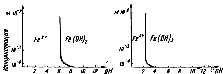
Рис. 10. Диаграммы осаждения ферро- ( \text{Fe}^{++} ) и ферри- ( \text{Fe}^{+++} ) гидроокисей из соответствующих ионных растворов (Segalen, 1964)
