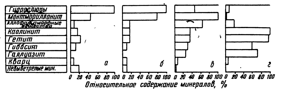
Рис. 35. Относительное содержание минералов в илистой фракции почв (<0,001 мм), сопряженных с выделяемыми фазами минеральных преобразований а—обызвесткованная, б—сиаллитная, в—глинная, г—ферраллитная
