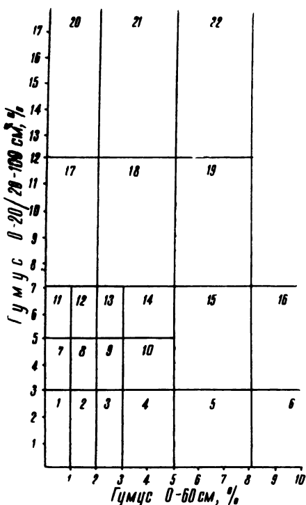
Рис. 17. График для кодирования почв по величине соотношения содержания гумуса в слоях 0—20 и 20—100 см и в слое 0—60 см
