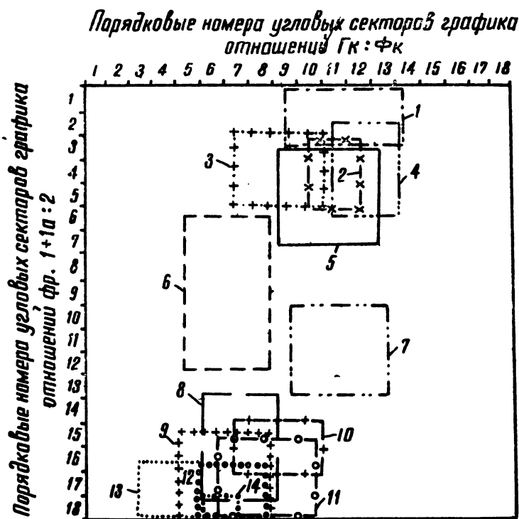
Рис. 32. Размещение вариограмм почв разных генетических типов по групповому и фракционному составу гумуса:
