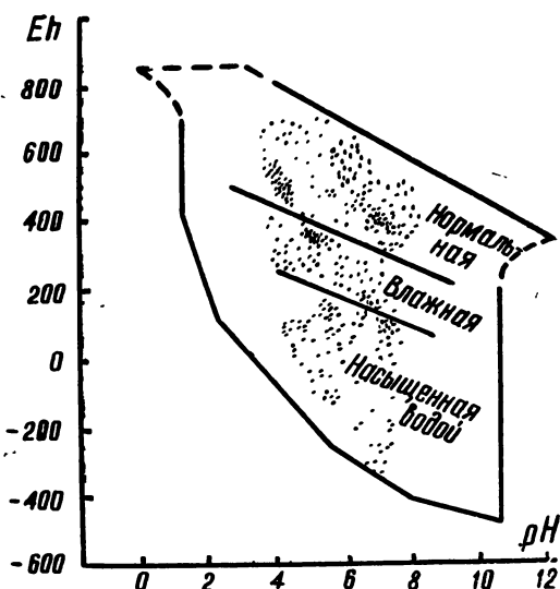
Рис. 1. Eh — pH параметры почв (Баас-Беккингем, Каплан, Мур, 1963)
