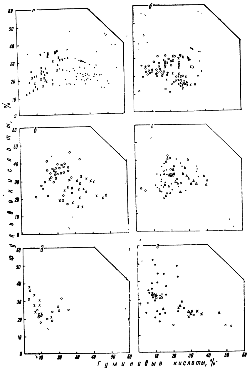
Рис 28. Распределение отметок группового состава гумуса некоторых характерных типов почв: а—черноземы (●), дерново-подзолистые и подзолы (×); б—сероземы (○), каштановые (×), тапкыры (●); в—бурые лесные (○), серые лесные (×); г—коричневые (Δ), желтоземы (●), красноземы субтропические (○), д—тундровые (×), глеево-подзолистые лесотундровые (○), е—смолницы (○), черные почвы тропиков (×), красноземы влажнотропические (●), желтые влажнотропические (Δ)
