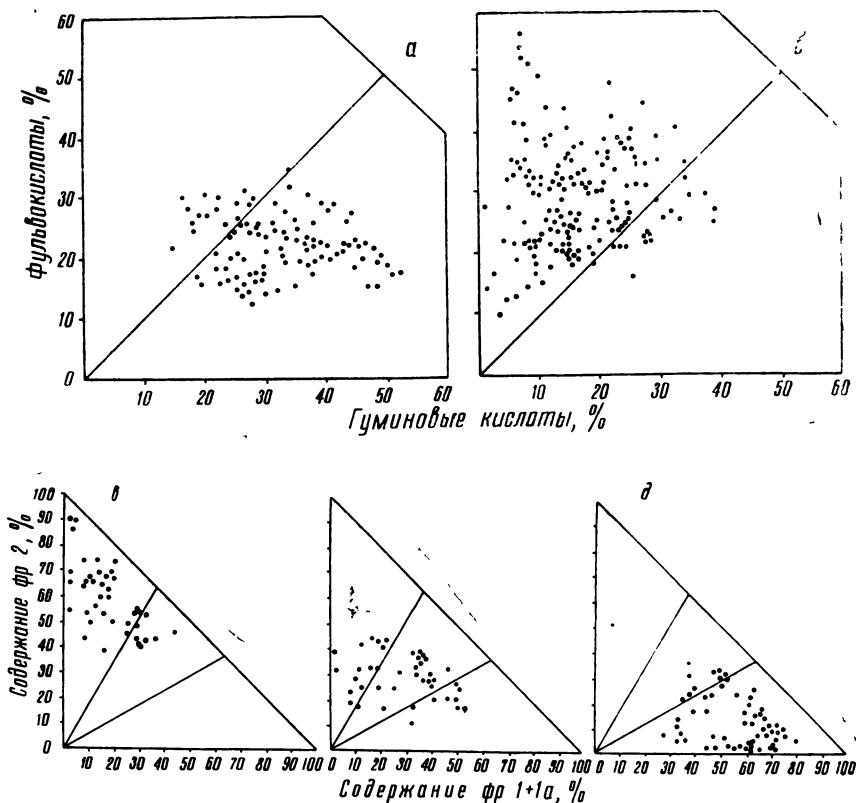
Рис. 31. Распределение отметок характерных совокупностей почв по групповому и фракционному составу гумуса: а —с преобладанием гуминовых кислот (черноземы, серые лесные, каштановые, смолницы, черные почвы тропиков); б —с преобладанием фульвокислот (сероземы, коричневые, желтоземы, бурые лесные, красноземы субтропические, тропические красные, тундровые, лесотундровые); в —с преобладанием фр. 2 (черноземы, смолницы, черные тропические, коричневые насыщенные, каштановые); г —с промежуточным соотношением фр. 1+1а и 2 (сероземы, серые лесные); д —с относительным преобладанием фр. 1+1а (дерново-подзолистые, глеево-подзолистые лесотундровые, коричневые ненасыщенные, бурые лесные, желтоземы, красноземы)
