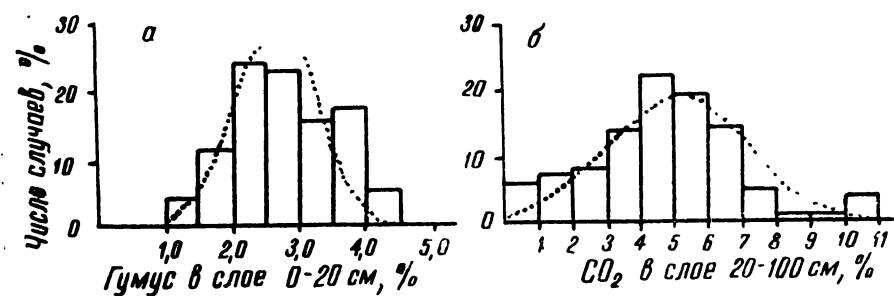
Рис. 27. Примеры статистического исследования репрезентативности данных по содержанию гумуса в слое 0—20 см каштановых почв (а) и содержанию в них CO 2 в слое 20—100 см (б) в совокупности почвенных разрезов, использованных в работе при составлении диагностических таблиц (столбиками показано распределение исходных данных в % к общему числу, точками—вычисленная кривая распределения)
