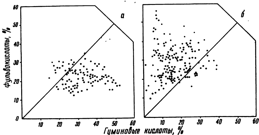
Рис. 2. Групповой состав гумуса образцов почв (Волобуев, 1962)
