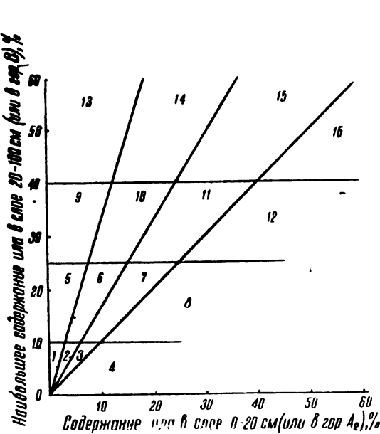
Рис. 23. График для кодирования почв по содержанию ила (частицы <0,001 мм) в слоях 0—20 и 20—100 см
