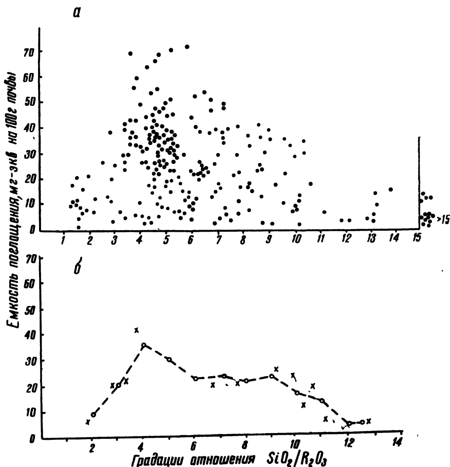
Рис. 6. Изменение емкости поглощения в слое почвы 0—50 (60) см в связи со значением отношения \text{SiO}_2/\text{R}_2\text{O}_3 в слое почвы 0—100 см по почвам Еяразии (степные, таежнолесные, субтропические, тропические и др.)
