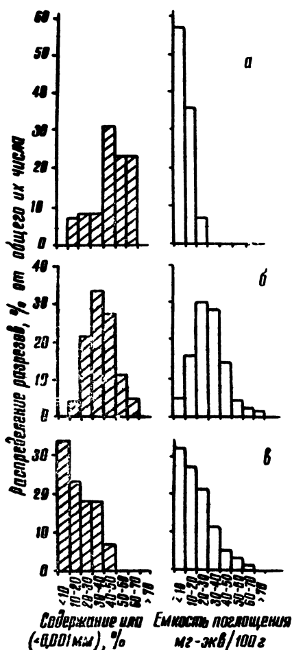
Рис. 8. Распределение разрезов по степени илливости и емкости поглощения по каждой из трех групп почв согласно значениям отношения \text{SiO}_2/\text{R}_2\text{O}_3 а—<3,5; б—3,5—5,5; в—>5,5
