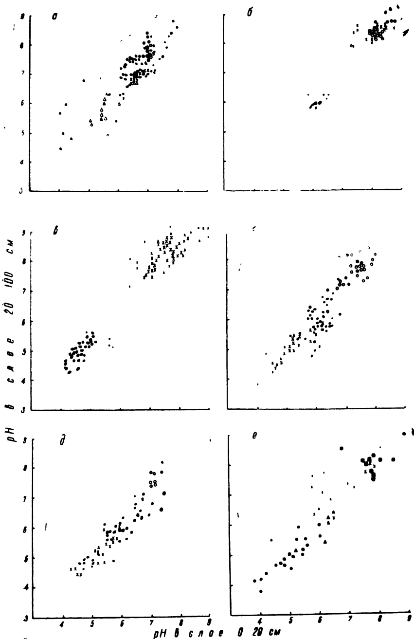
Рис. 20. Распределение отметок рН почв в слоях 0—20 и 20—100 см а—черноземы карбонатные и южные (○), выщелоченные и оподзоленные (×), все другие, в том числе с неуказанным подтипом (● тундровые почвы без подразделения (△); б—сероземы (×), серые лесные (●), пустынные почвы США (○); в—каштановые (×), дерново-подзолистые и подзолы (●); г—коричневые (○), желтоземы (●), красноземы субтропические (×); д—бурые лесные: остаточные карбонатные (○), оподзоленные (×), все другие, в том числе с неуказанным подтипом (●); е—красные влажнотропические (●), желтые влажнотропические (○), опесчаненные влажнотропические (△), смолиницы и грумосоли (США) (×), черные тропические (■)
