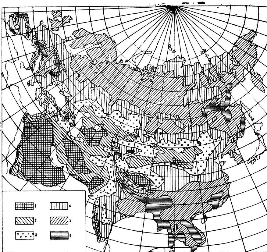
Рис. 40. Климатические зоны увлажнения Евразии.
