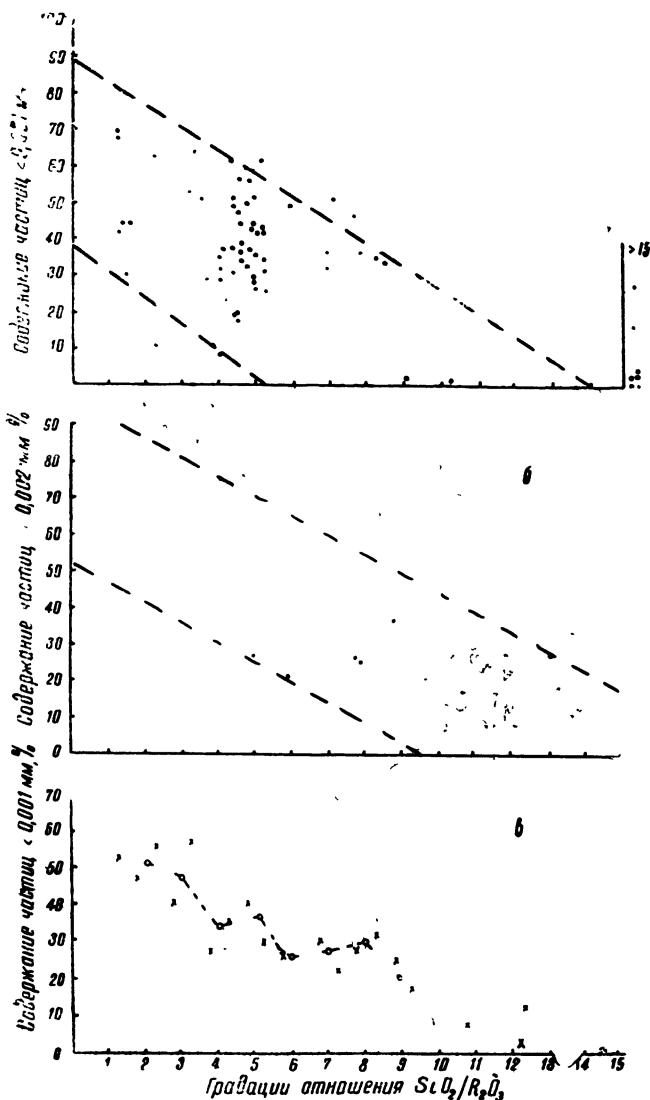
Рис 5. Изменение содержания илистых частиц в связи с значением отношения SiO_2/R_2O_3 в слое 0—100 см почв Евразии (степные, таежнолесные, субтропические, тропические и др.)
