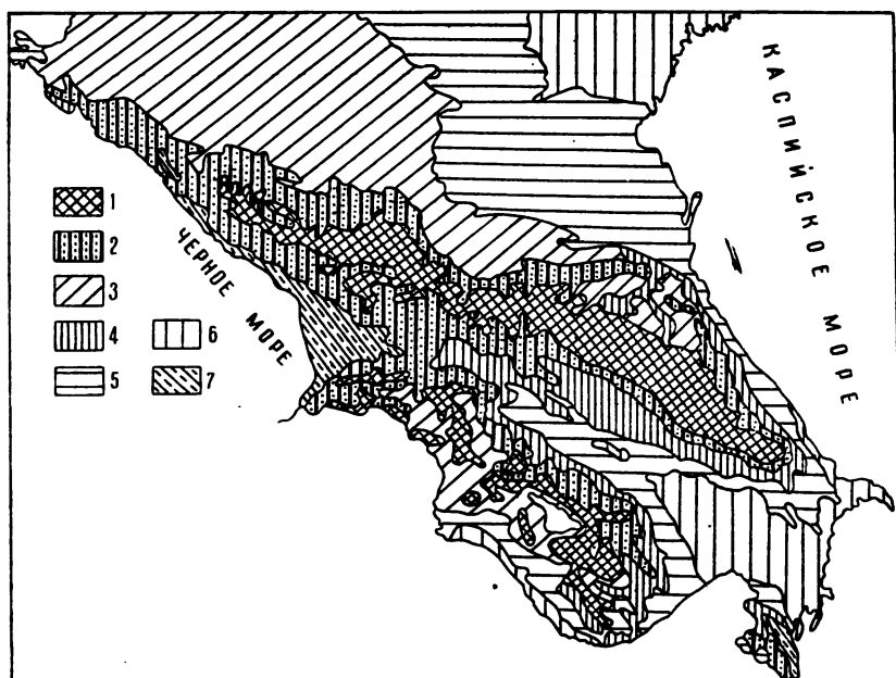
Рис. 50. Главные почвенные зоны Кавказа: 1—холододерновой общности; 2—дерново-подзолистой общности; 3—черноземной общности; 4—коричнево-земной общности; 5—каштановоземной общности; 6—сероземной общности; 7—желтоземной общности
