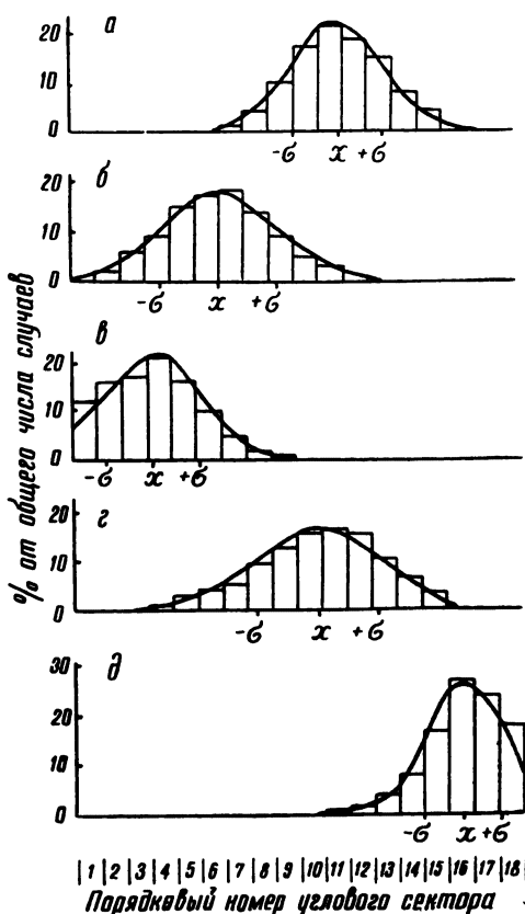
Рис. 30. Кривые распределения почв по градации отношений Гк/Фк и фр. 1+1а/2 (столбики — исходные данные, линии — вычисленные кривые). x — средние значения; \sigma — квадратические отклонения: а, б — с преобладанием в групповом составе соответственно гуминовых и фульвокислот; в — с преобладанием во фракционном составе фр. 2; г — с относительно равным содержанием фр. 2 и 1+1а; д — с преобладанием фр. 1+1а
