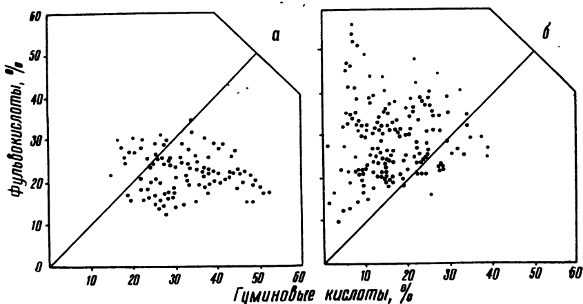
Рис. 2. Групповой состав гумуса образцов почв (Волобуев, 1962) а — дерновые, б — лесные почвы
