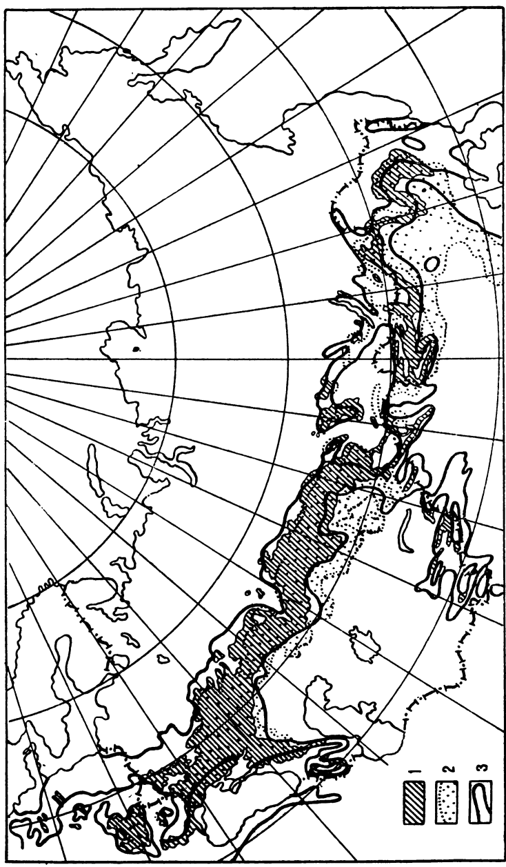
Рис. 43. Ареал чернозема и фитоклиматические условия его распространения на пространстве северной части Евразии: 1—районы луговых и типичных степей, 2—внешние границы зоны увлажнения D, DE в пределах зон тепла III, IV, V
