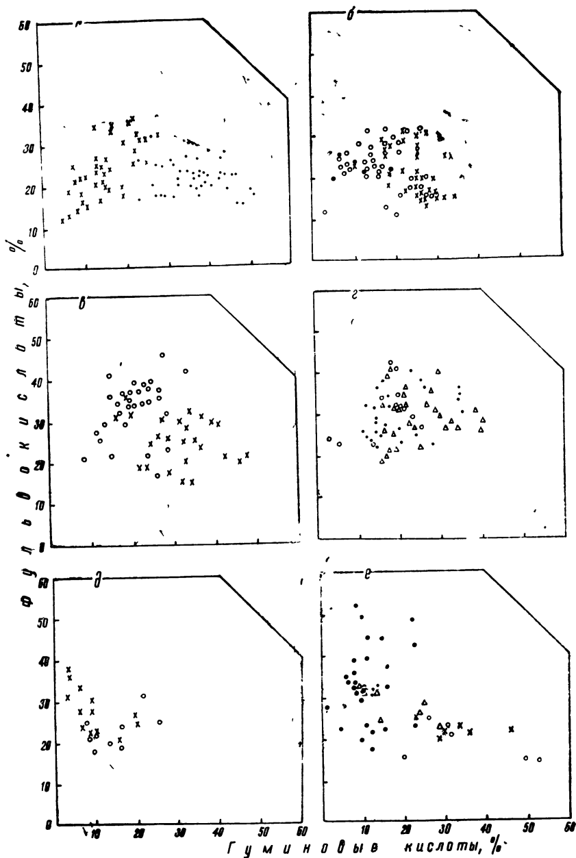
Рис 28. Распределение отметок группового состава гумуса некоторых характерных типов почв: а—черноземы (●), дерново-подзолистые и подзолы (×); б—сероземы (○), каштановые (×), тапкы (●); в—бурые лесные (○), серые лесные (×); г—коричневые (△), желтоземы (●), красноземы субтропические (○), д—тундровые (×), глеево-подзолистые лесотундровые (○), е—смолницы (○), черные почвы тропиков (×), красноземы влажнотропические (●), желтые влажнотропические (△)
