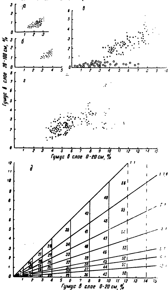
Рис. 14. Распределение отметок содержания гумуса в почвах в слоях 0—20 и 20—100 см и кодовый график по гумусу а—каштановые; б—темно-каштановые; в—черноземы: южные (×), обыкновенные (●), дерново-подзолистые (○); г—все черноземы (учтенные при обработке); д—график для кодирования почв по содержанию гумуса в слоях 0—20 и 20—100 см (номера кода проставлены на поле графика—1—56), справа указаны величины соотношения в содержании гумуса в слоях 0—20 и 20—100 см
