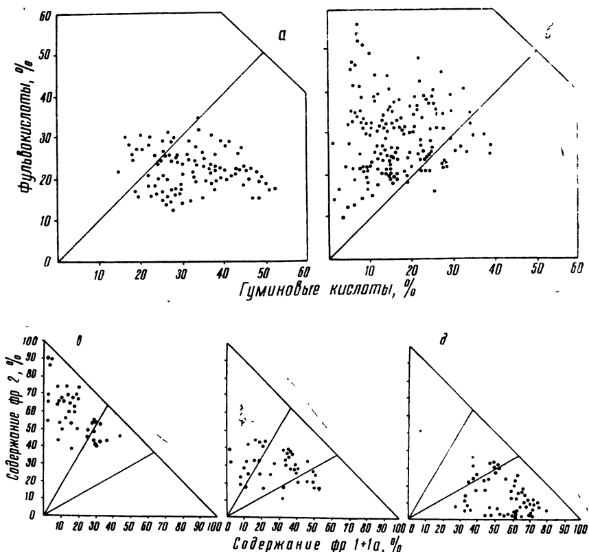
Рис. 31. Распределение отметок характерных совокупностей почв по групповому и фракционному составу гумуса: а—с преобладанием гуминовых кислот (черноземы, серые лесные, каштановые, смолницы, черные почвы тропиков); б—с преобладанием фульвокислот (сероземы, коричневые, желтоземы, бурые лесные, красноземы субтропические, тропические красные, тундровые, лесотундровые); в—с преобладанием фр. 2 (черноземы, смолницы, черные тропические, коричневые насыщенные, каштановые); г—с промежуточным соотношением фр. 1+1а и 2 (сероземы, серые лесные); д—с относительным преобладанием фр. 1+1а (дерново-подзолистые, глеево-подзолистые лесотундровые, коричневые ненасыщенные, бурые лесные, желтоземы, красноземы)
