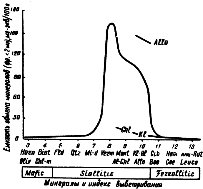
Рис. 9 Величина обменной способности фракции <0,002 мм различных классов минералов с разными номерами индекса выветривания (по Jackson, 1968)
