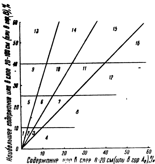
Рис. 23. График для кодирования почв по содержанию ила (частицы <0,001 мм) в слоях 0—20 и 20—100 см
