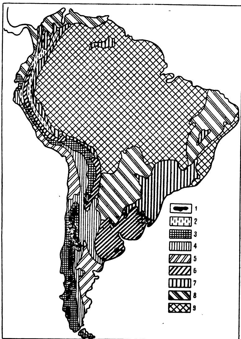
Рис. 58. Главные почвенные зоны Южной Америки:
