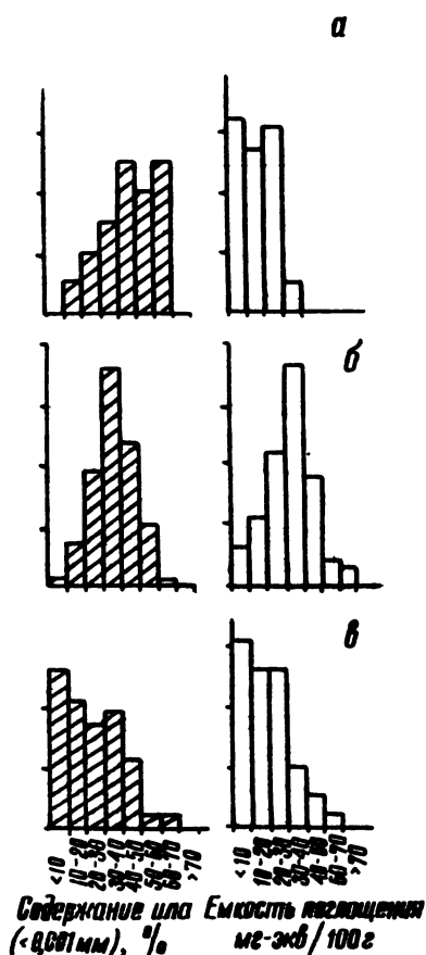
Рис. 8А. Распределение разрезов характерных групп почв по степени илливости и емкости поглощения а—красноземы тропические и субтропические, латеритизированные почвы и др.; б—коричневые, бурые лесные, желтоземы, смолиницы, регеры и др.; в—черноземы, серые лесные, каштановые, сероземы, дерново-подзолистые, подзолы и др.
