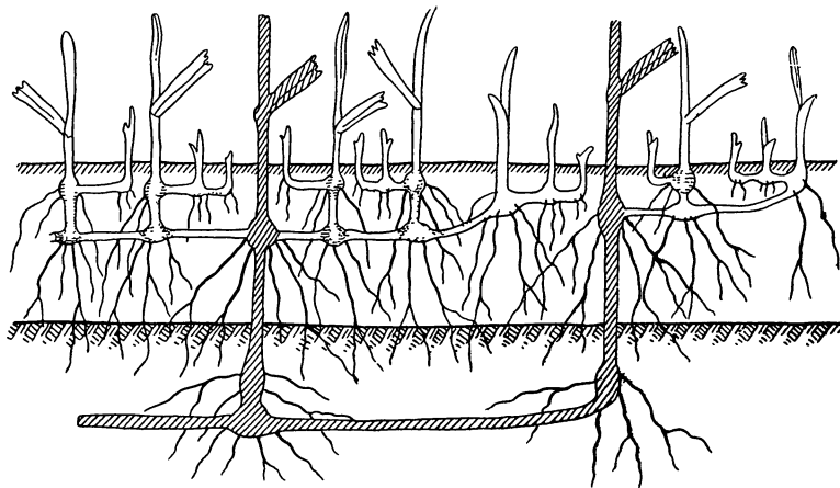
Рис. 10. Схема возобновления вегетативных органов корневицевого злака после заноса его отложениями зернистой поймы.
