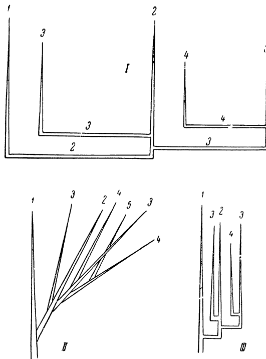
Рис. 14. Диаграмма трех основных типов кущения злаков:
