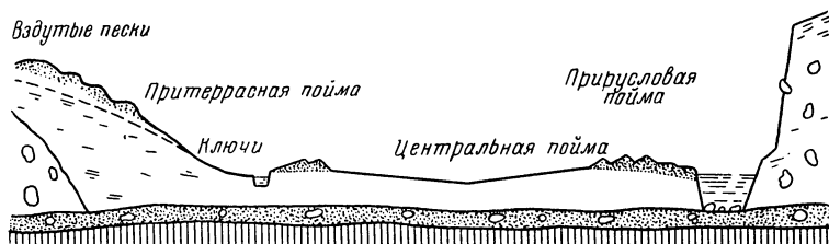
Рис. 2. Схема поперечного разреза участка зернистой поймы.
