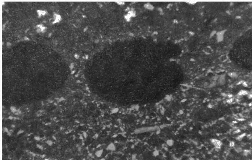
Фото 2. Лужайковые поры у по- верхности почв торрифлювент, штат Аризона. Скрещенные николи, ув. 71х.
