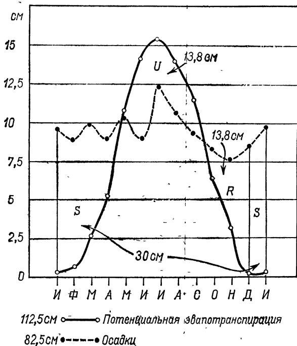
Рис. 47. Среднегодовой баланс влаги в почве уинстон-сейлем, штат Северная Каролина.
