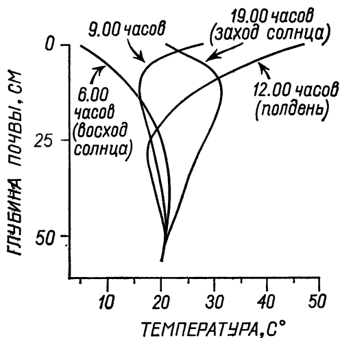
Р и с. 15. Зависимость дневных температур почвы от глубины.
