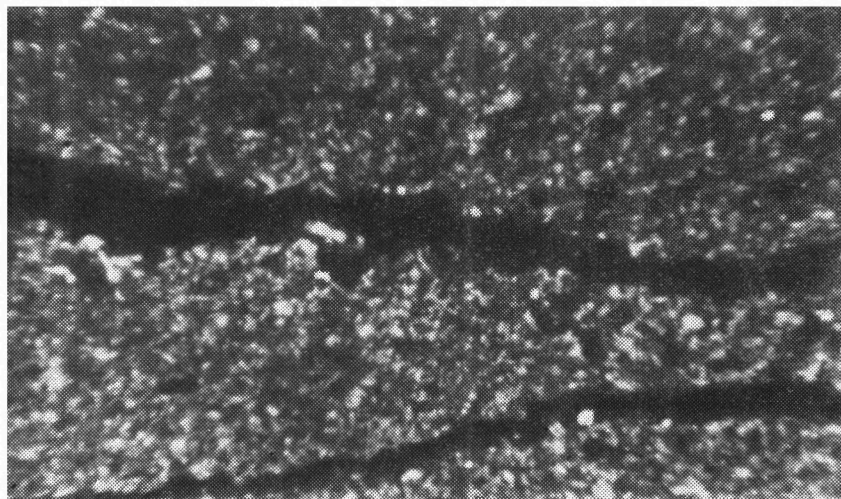
Фото 3. Прямые трещины в поверхностных горизонтах почв торрифлювент, штат Аризона. Скрещенные трещины, ув. 71х.
