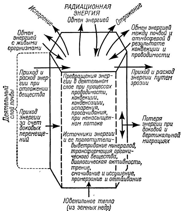
Р и с. 1. Схематическое изображение источников энергии и преобразования энергии в деятельном слое почвенного педона.
