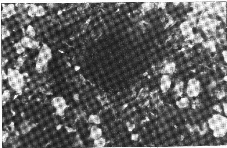
Фото 10. Аржиллан с низкой степенью ориентации на песчаных зернах. Погасание скорее пятнистое, чем отчетливо полосчатое. Скрещенные николи, ув. 71х.
