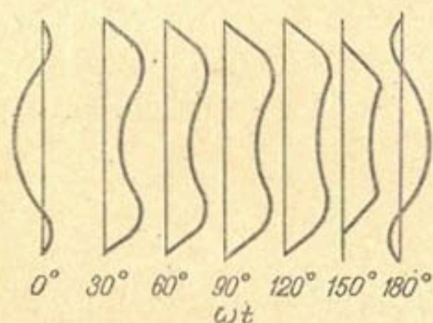
Рис. 17. Характер изменения эиур скоростей во времени при гармоническом законе изменения перепада давления в капилляре [72]
