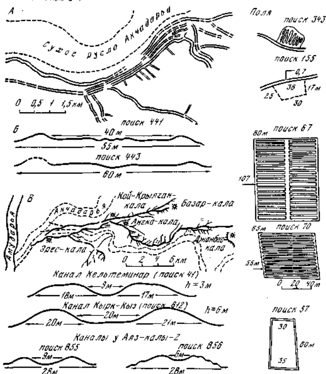
Рис. 19. Историческое развитие систем орошения в низовьях Амударьи (VII в. до н. э. — начало XIII в. н. э.):
