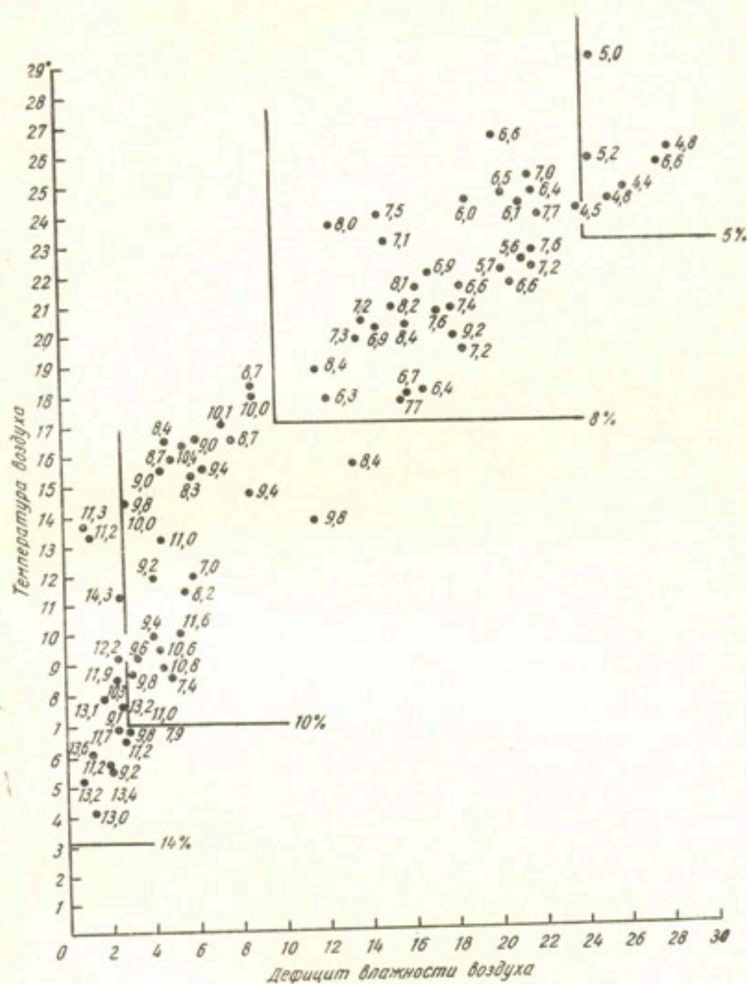
Рис. 1. Зависимость влажности хлопка-сырца от температуры и дефицита влажности воздуха.
