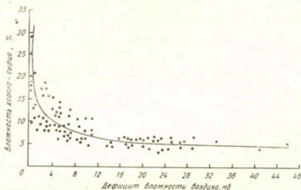
Рис. 2. Зависимость влажности хлопка-сырца от дефицитов влажности воздуха.
