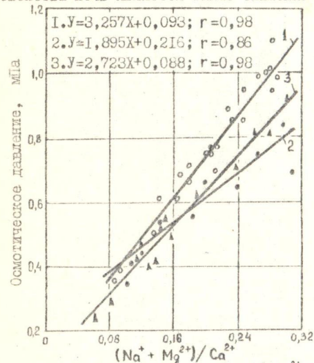
Рис. 2. Зависимость P_{осм} = f\left(\frac{Na^+ + Mg^{2+}}{Ca^{2+}}\right) (1 - контроль; 2 - навоз; 3 - лигнин)
