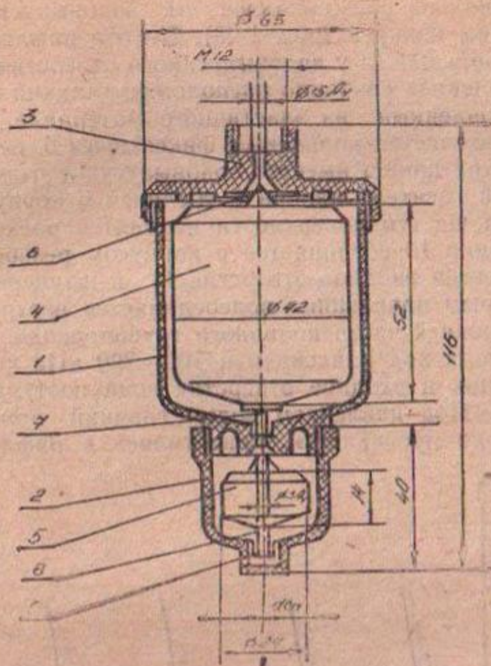
Рис. 1.24. Капельница «Узгипроводхоз-2»
