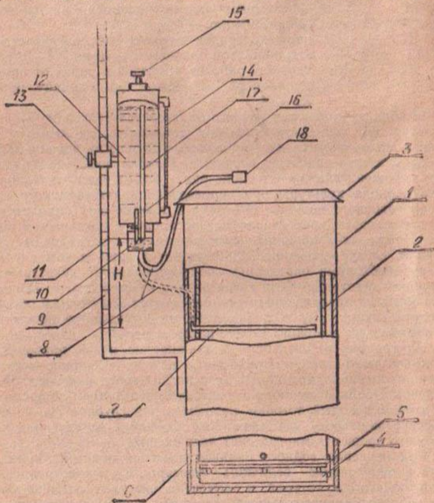
Рис. 2.1. Испаритель
