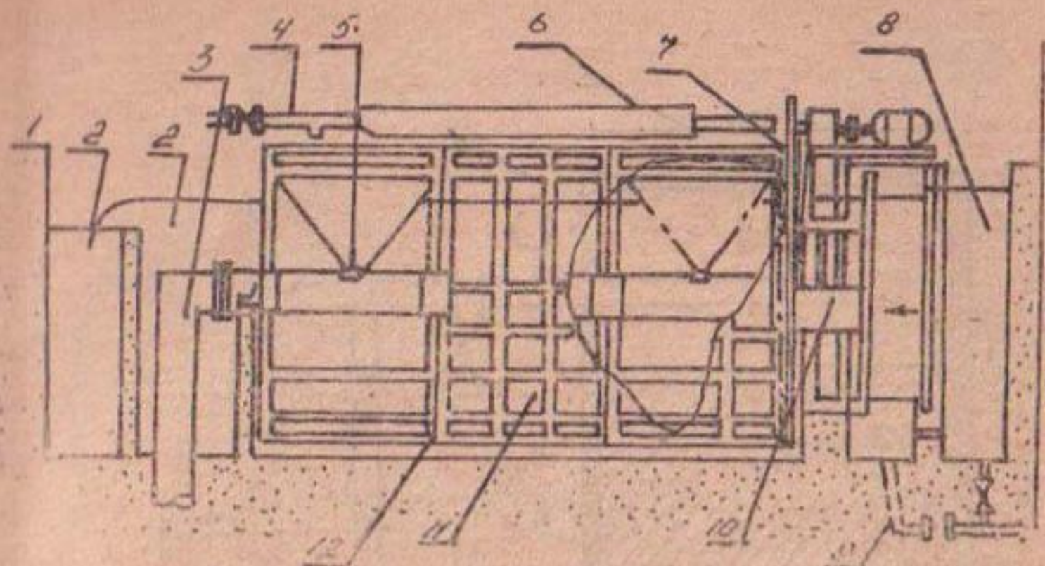
Рис. 1.8. Конструктивная и монтажная схема микрофильтра
