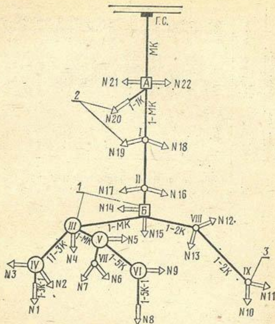
Рис. 12. Схема оросительной системы:
