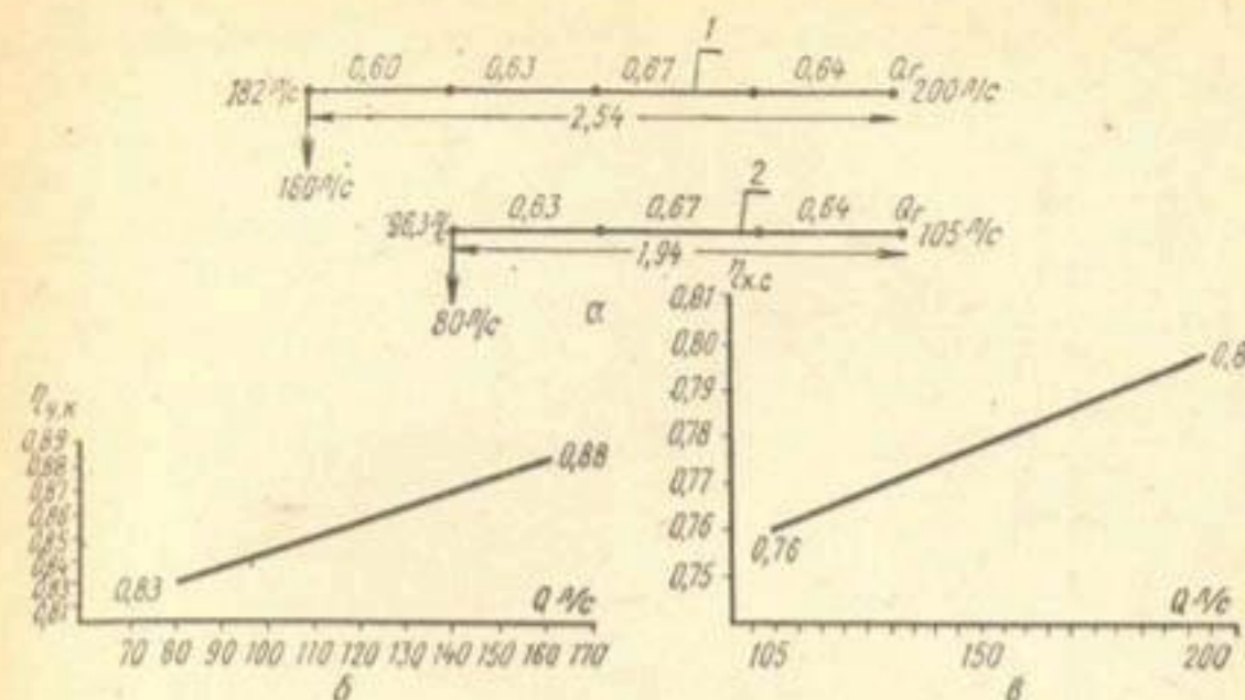
Рис. 2. Расчетная схема распределения расходов (а) по длине хозяйственного распределителя 1-МК и графики к. п. д. участковых (полевых) каналов (б) и внутрихозяйственной сети (в):
