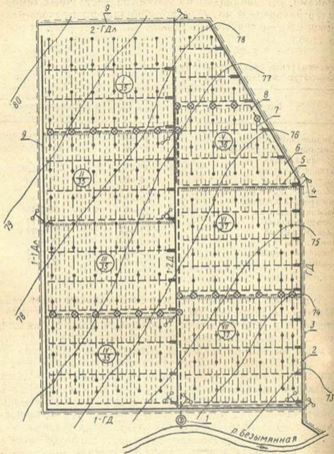
Рис. 47. Осушительно-оросительная сеть в колхозе «Победа»:
