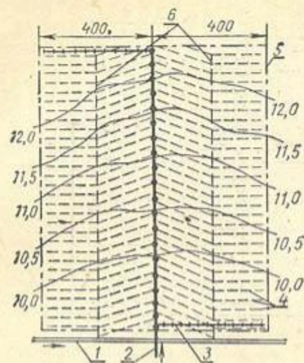
Рис. 28. Осушительно-оросительная система при поливе дождевальной машиной ДКШ-64 («Волжанка»):
