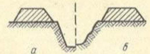
Рис. 42. Деформация канала от давления кавальера на откос:
