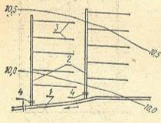
Рис. 30. Осушительно-увлажнительная система с увлажнением почвы из открытой сети за счет воды собственного водосбора:
