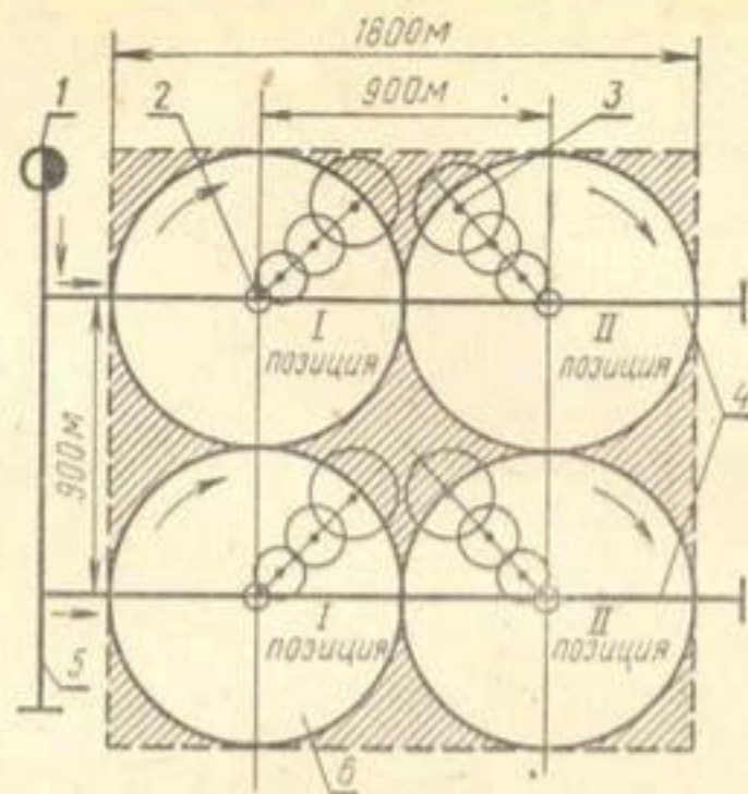
Рис. 5. Схема работы самоходного дождевального агрегата «Фрегат»:
