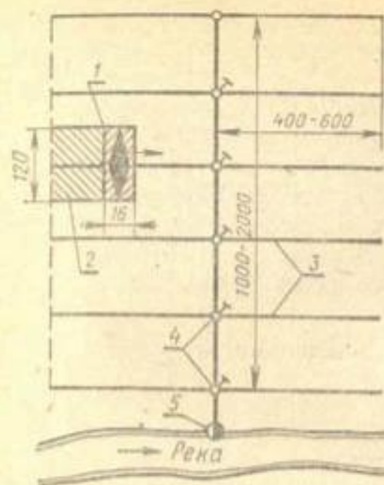
Рис. 3. Схема комбинированной оросительной сети для полива сельскохозяйственных культур агрегатом ДДА-100М: 1 — агрегат ДДА-100М; 2 — поливная площадь; 3 — открытые оросители; 4 — гидранты-водоупуски; 5 — насосная станция (размеры в м).
