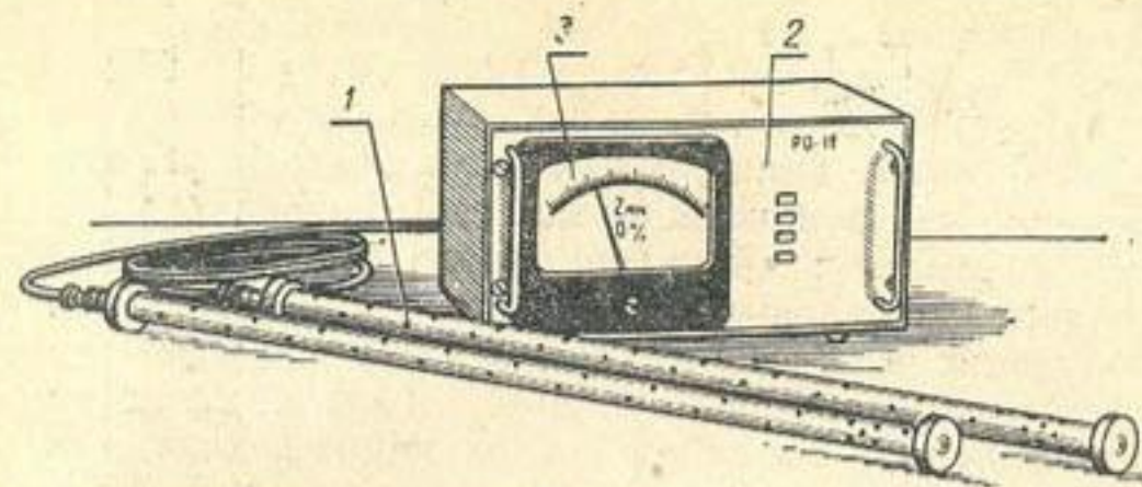
Рис. 11. Общий вид водомера РО-1Е:
