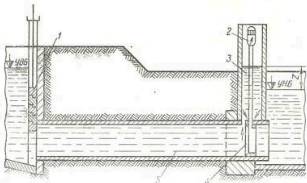
Рис. 14. Трубчатый водомер-водоотпуск (ТВС):
