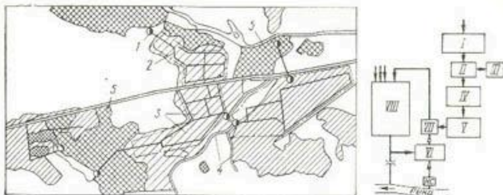
Рис. 46. Схемы сельскохозяйственных полей орошения (1 — насосные станции; 2 — сеть трубопроводов; 3 — ЗПО; 4 — реки; 5 — поселки, из которых используются сточные воды) и оборотного водопользования (I — животноводческий комплекс; II — механическая очистка; III — торфокомпост; IV, V, VI — отстойники-накопители; VII — смеситель; VIII — поля орошения).
