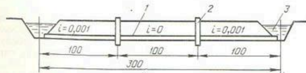
Рис. 51. Схема совмещенного действия коллектора на осушение и орошение:
