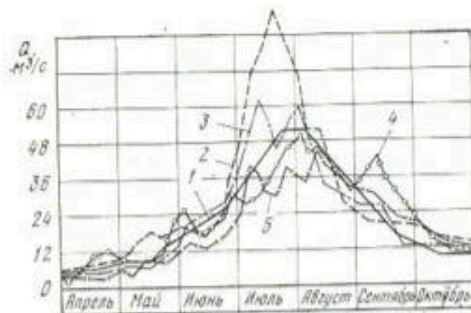
Рис. 20. Расчетные и фактические расходы реки: 1 — расчетные расходы обеспеченности 50 %; 2, 3, 4, 5 — фактические расходы за отдельные годы.
