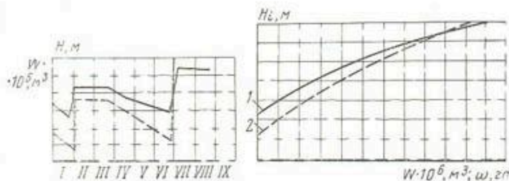
Рис. 35. Графики работы водохранилища: 1 — объемы воды; 2 — площади поверхности водохранилища.
