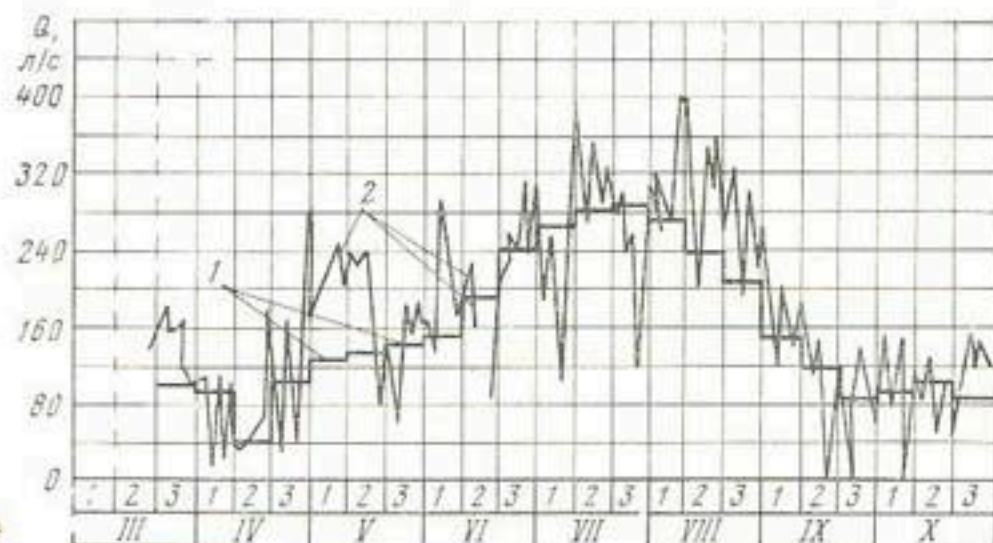
Рис. 8. График поступления воды в точку выдела на массив площадью 223 га:
