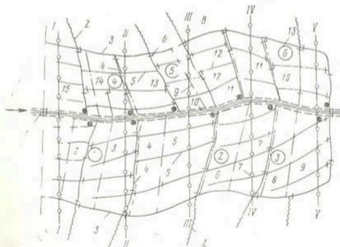
Рис. 4. Схема осушительной системы: 1 — водоприемник; 2 — притоки (ручьи); 3 — нагорные каналы; 4 — магистральные каналы; 5 — сборники и соединительные каналы; 6 — шлюзы и гидротехнические сооружения; 7 — скважины; 8 — створы скважин; 9 — границы хозяйств; 10 — дамбы; 11 — насосные станции; 12 — массивы; 13 — массивы; 1...V — створы; 1...15 — хозяйства; 1...6 в кружках — массивы.
