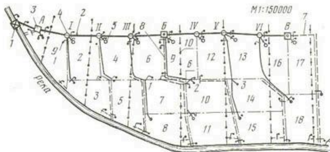
Рис. 2. Схема межхозяйственной оросительной системы хлопковой зоны: 1 — головное сооружение; 2 — магистральный канал; 3 — узлы командования А, Б, В; 4 — узлы распределения 1, II, ..., VI; 5 — точки выдела воды 1... 18; 6 — пропорциональные подделители 1, 2, 3; 7 — сбросы; 8 — межхозяйственные распределители; 9 — посты учета воды; 10 — скважины для наблюдений за грунтовыми водами.
