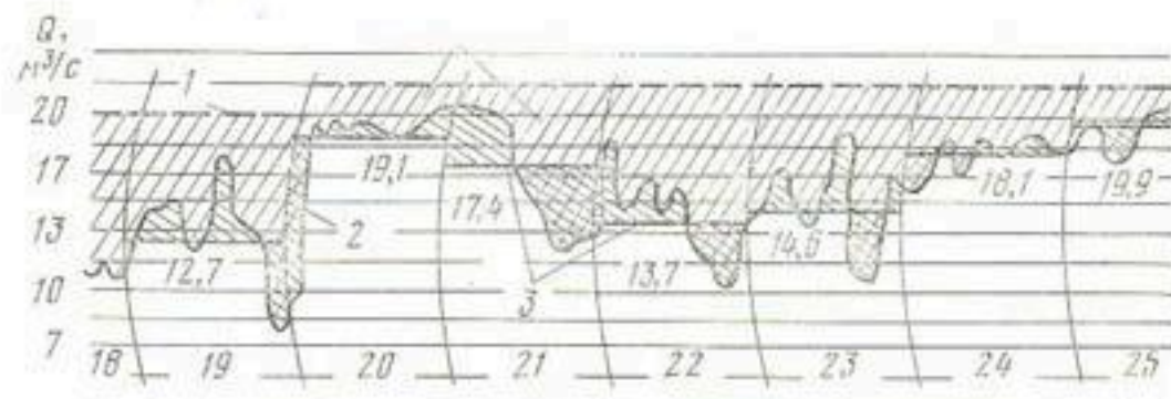
Рис. 7. График забора воды в систему в критический период (июнь): 1 — план забора воды; 2 — фактические расходы; 3 — среднесуточные расходы; 4 — недостаток воды.
