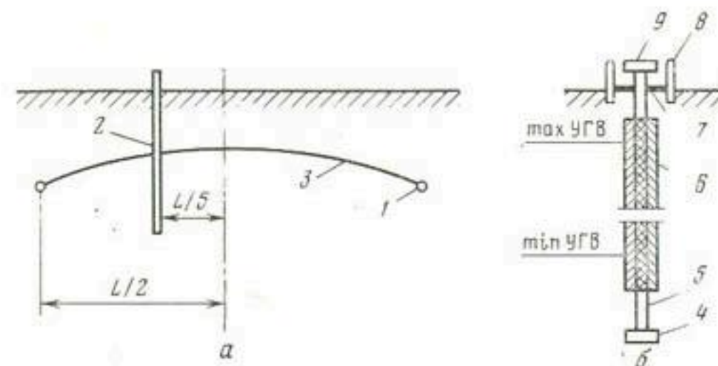
Рис. 36. Наблюдательная скважина при дренаже: а — схема размещения; б — конструкция скважины: 1 — дрена; 2 — скважина; 3 — депрессионная кривая; 4 — пробка; 5 — отстойник; 6 — фильтр; 7 — глиняный замок; 8 — колодец; 9 — оголовок.
