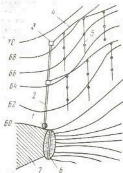
Рис. 44. Схема оросительной системы из пруда:
