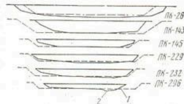
Рис. 24. Профили магистрального канала по контрольным поперечникам: 1 — после строительства; 2 — через 15 лет эксплуатации.
