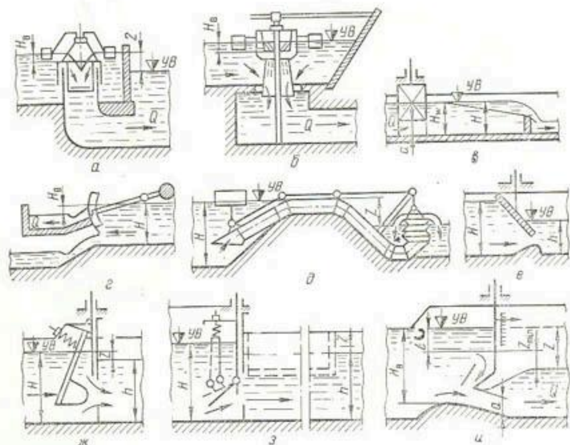
Рис. 61. Схемы некоторых гидроавтоматов постоянных расходов воды:
