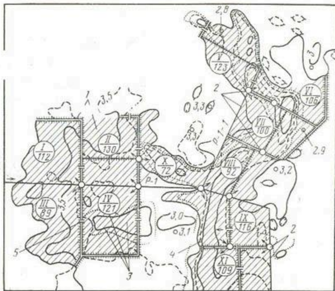
Рис. 39. Схема лиманов на обводнительно-оросительной системе: 1 — лиманы и палы; 2 — каналы и выпуски воды; 3 — номер секции и площадь (га); 4 — сбросной канал; 5 — выпуски воды из секции в секцию.
