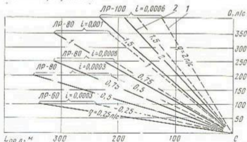
Рис. 27. График расход по длине лотка (справа налево) при подаче воды в борозды:
