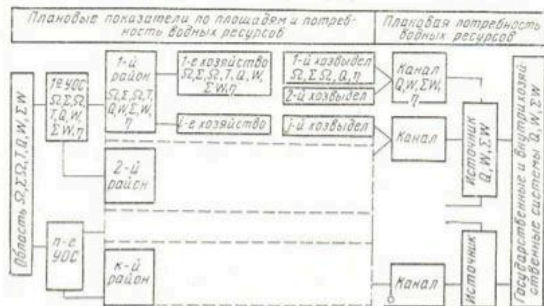
Рис. 65. Схема расчета на ЭВМ плана водораспределения для области: Q — площади; T — поливы-смены; η — КПД; Q — расход; W — сток.
