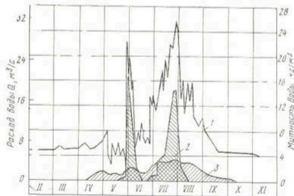
Рис. 22. Расходы реки и мутность воды: 1 — расходы воды; 2, 3 — расходы донных и взвешенных наносов.
