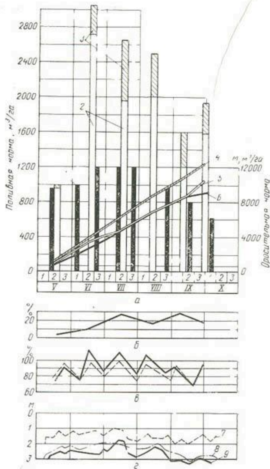
Рис. 17. Фактический режим поливов хлопчатника на участке:
