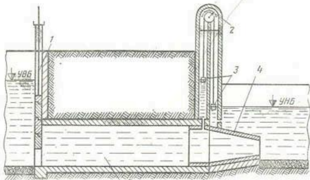
Рис. 13. Водомер-водоотпуск:
