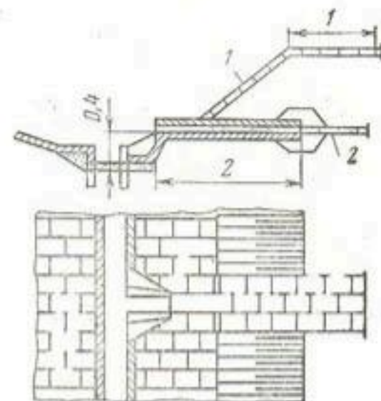
Рис. 53. Устье на канале: 1 — одерновки; 2 — дрена. (Размеры в м.)
