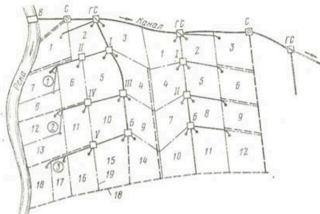
Рис. 3. Схема оросительных систем на крупном канале: В — водозабор из реки в канал; С — сбросы на канал; ГС — головные сооружения на канале; В — узлы командования; I...V — узлы распределения; 1...18 — точки выдела воды; 1, 2, 3 в кружках — пропорциональные вододелители; 18 — сбросные каналы; 19 — границы хозяйств.
