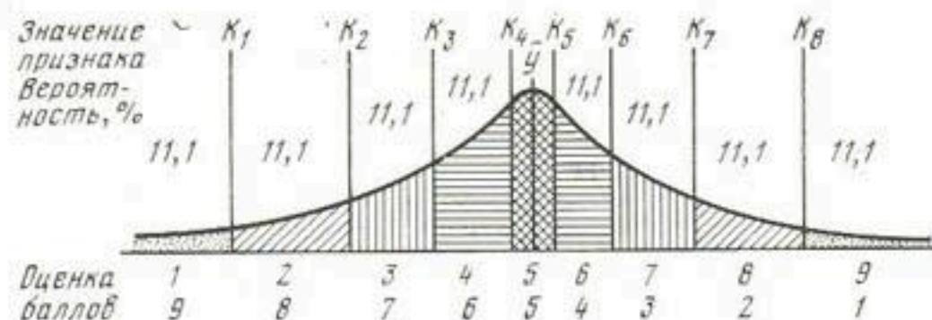
Рис. 25. Частота распределения случайных величин.
