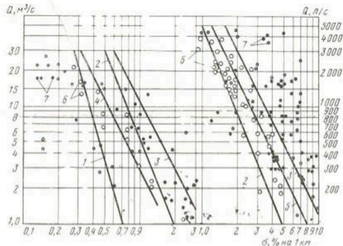
Рис. 21. Удельные расчетные (1 — для слабопроницаемых грунтов \sigma=0,7/Q^{0,3} ; 2 — для среднепроницаемых \sigma=1,9/Q^{0,4} ; 3 — для сильнопроницаемых грунтов \sigma=3,4/Q^{0,6} ; 4 — в магистральном канале \sigma=1,69/Q^{0,3} ; 5 — в распределительных каналах \sigma=2,52/Q^{0,6} ) и замеренные (6, 7 — на Атбашинской и на Вахшской системах) потери воды в межхозяйственных каналах.
