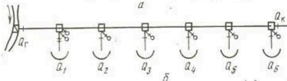
Рис. 16. График зависимости потерь воды в магистральном канале от расхода воды в голове канала (а) и схема расчета потерь воды по длине канала (б):
