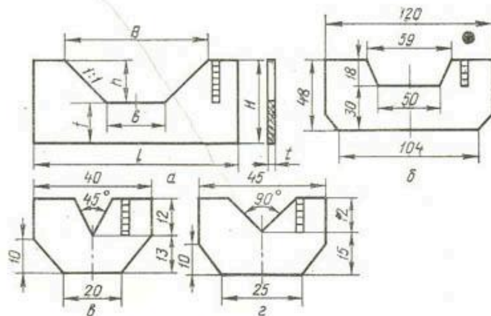
Рис. 15. Водосливы-водомеры:
