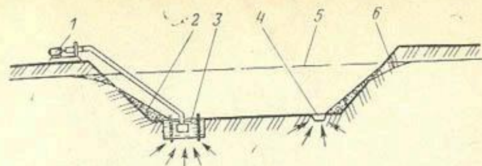
Рис. 22.2. Открытый водоотлив:
