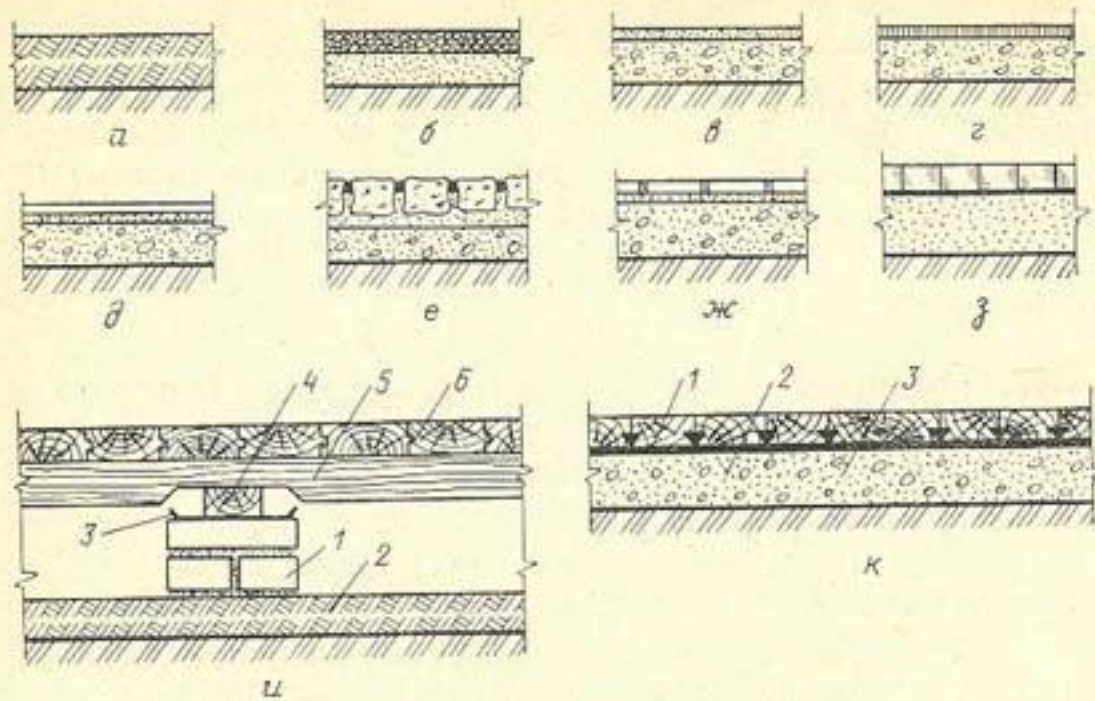
Рис. 18.22. Полы:
