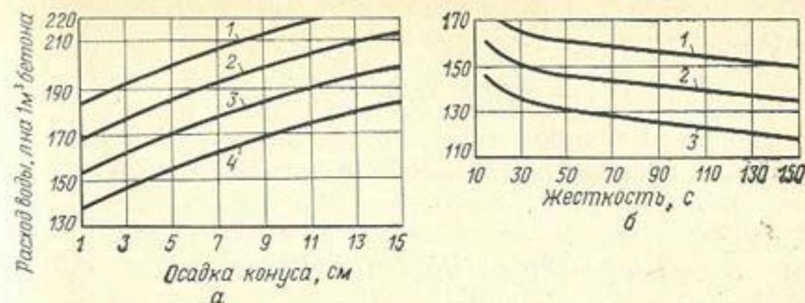
Рис. 5.4. Водопотребность пластичных (а) и жестких (б) бетонных смесей из портландцемента, песка средней крупности с водопоглощением 7% и гравия:
