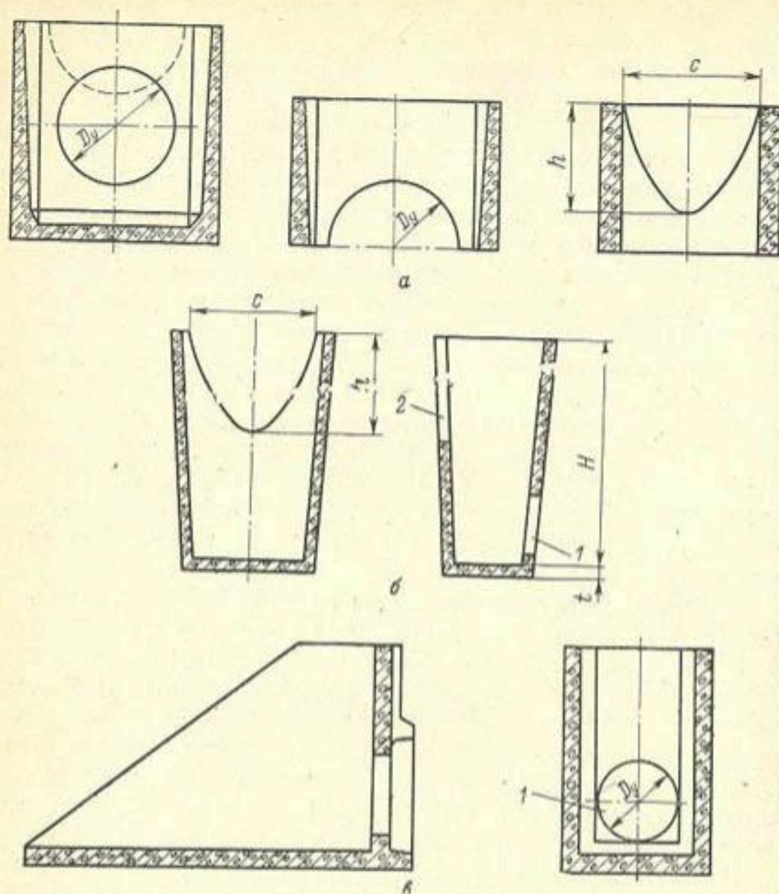
Рис. 7.4. Сборные железобетонные элементы водорегулирующих и водозаборных сооружений оросительных систем:
