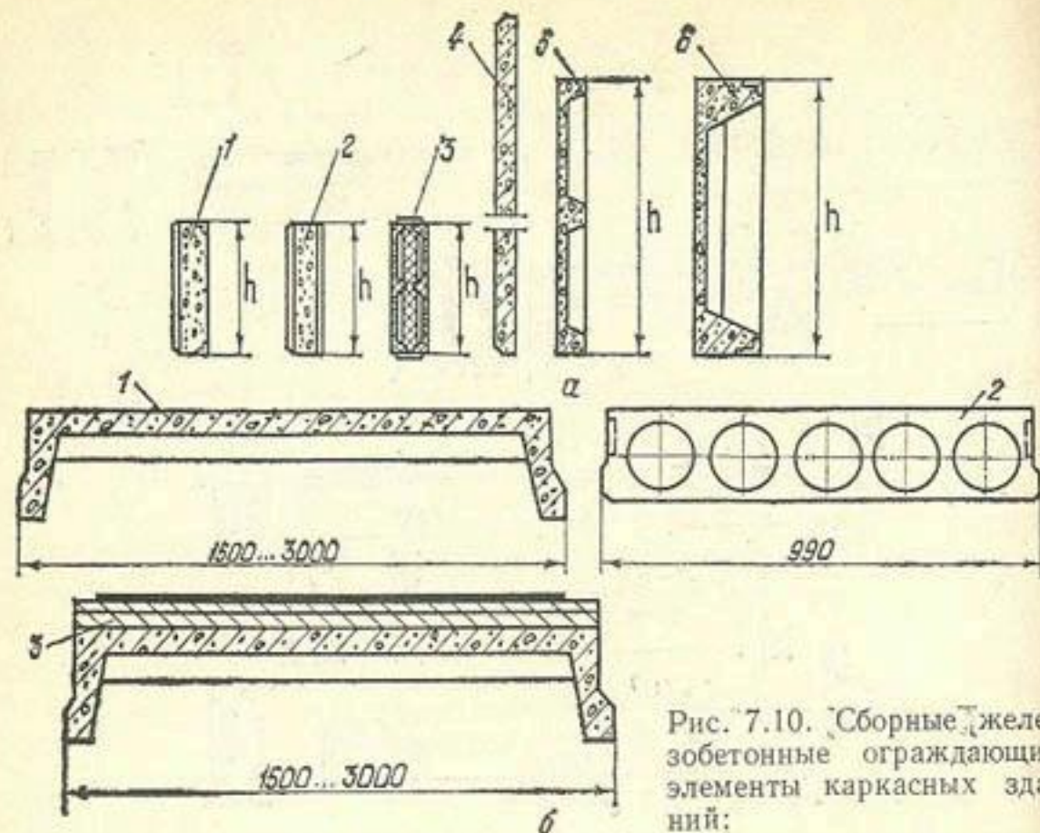
Рис. 7.10. Сборные железобетонные ограждающие элементы каркасных зданий: а — стеновые панели: 1 — однослойная легковесная с наружным фактурным слоем; 2 — однослойная из ячеистого бетона с наружным и внутренним фактурными слоями; 3 — многослойная из ребристых плит с прослойкой из полужесткой минераловатной плиты; 4 — однослойная из обычного бетона для неотапливаемых зданий; 5, 6 — однослойные ребристые из обычного бетона; б — панели перекрытий: 1 — ребристая; 2 — с круглыми пустотами; 3 — с теплоизоляционным слоем.
