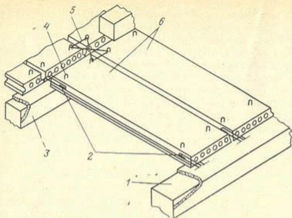
Рис. 18.15. Перекрытие из сборных железобетонных плит:
