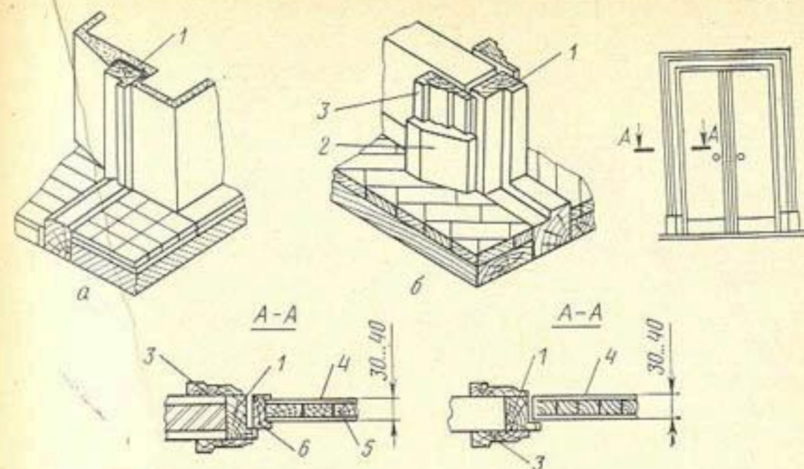
Рис. 18.27. Заполнение дверного проема:
