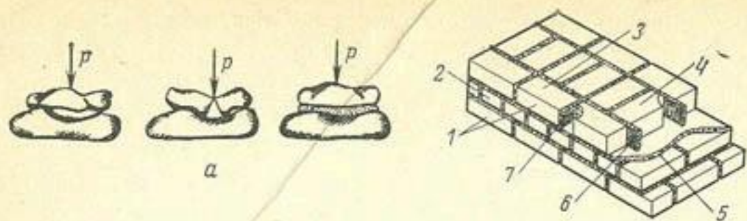
Рис. 24.1. Схемы к правилам разрезки каменной кладки:
