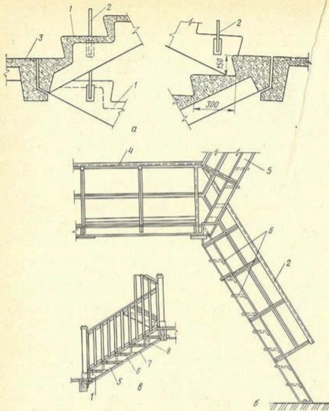
Рис. 18.25. Лестницы:
