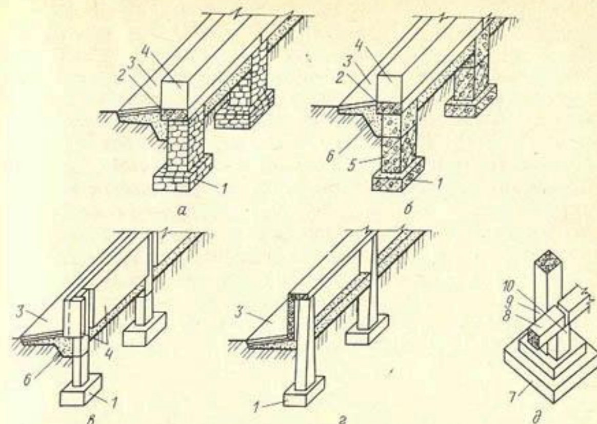
Рис. 18.4. Столбчатые фундаменты:
