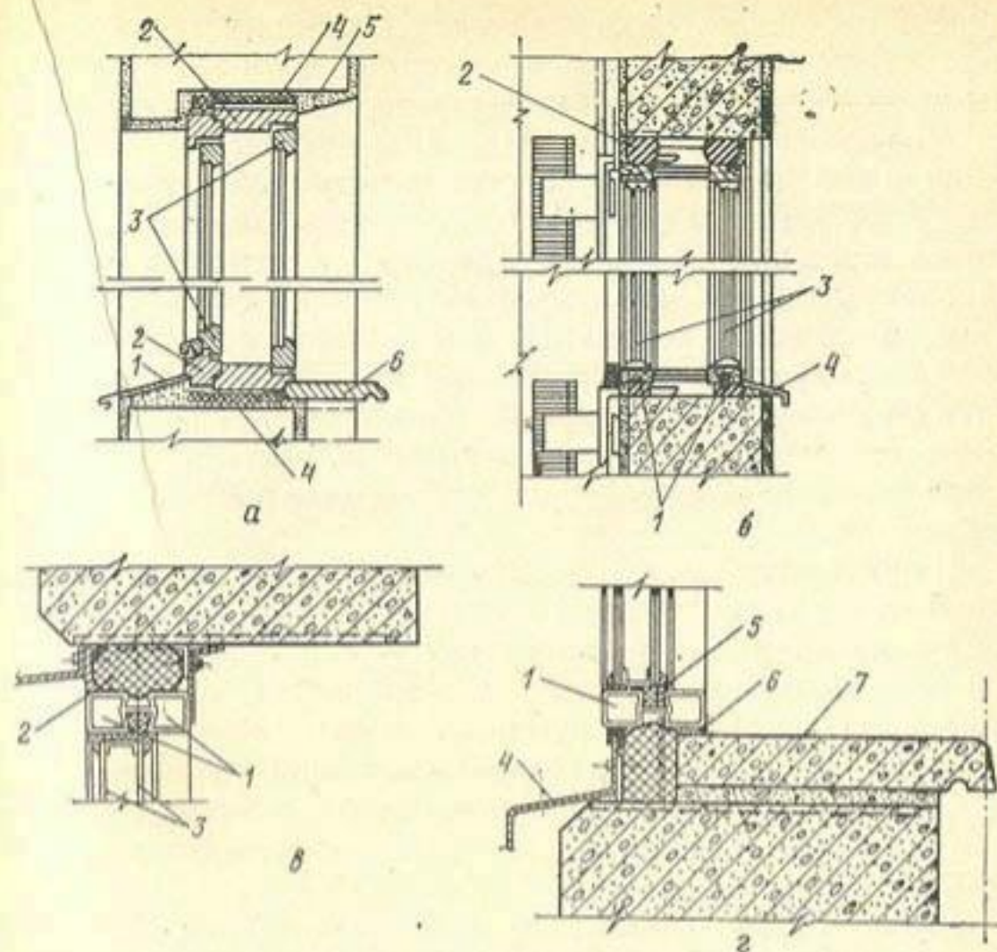
Рис. 18.26. Оконные проемы:
