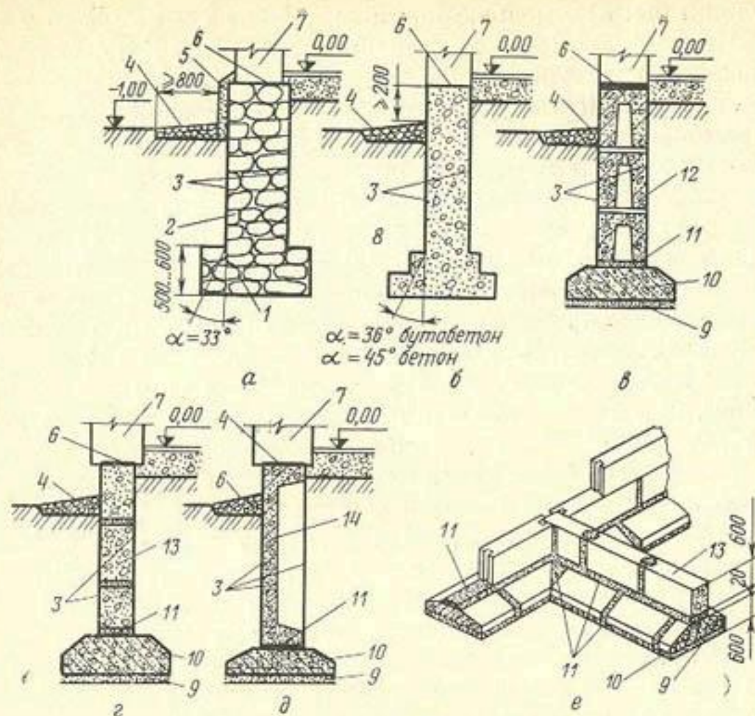
Рис. 18.3. Ленточные фундаменты:
