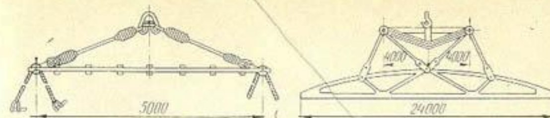
Рис. 23.7. Самоблокирующие траверсы.
