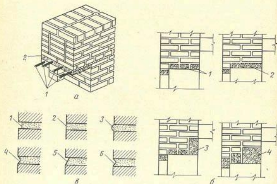
Рис. 18.13. Конструктивные элементы каменных стен: а — рядовая проемная перемычка кирпичных стен: 1 — стальная арматура; 2 — раствор повышенной марки; б — то же, из сборных железобетонных элементов: 1 — железобетонные несущие бруски; 2 — железобетонная плита; 3 — железобетонный несущий брусок; 4 — железобетонная несущая балка-брусок; в — расшивка швов кирпичных стен: 1 — прямоугольная заглубленная; 2 — прямоугольная вподрезку; 3 — выпуклая; 4 — вогнутая; 5 — односрезная; 6 — двухсрезная.
