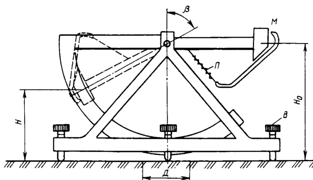
Рис. 6.13. Прибор для определения сцепления колес автомобиля с покрытием: М – груз; В – регулировочный винт; П – пружина; H_0 – начальная высота подъема груза; Д – диаметр следа колеса; \beta – угол отклонения маятника.
