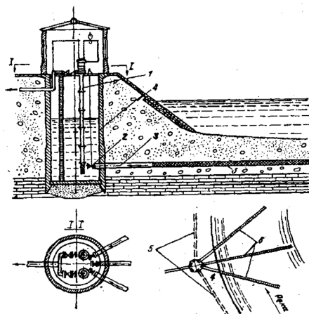
Рис. 7.1. Подрусловой лучевой дозатор: 1 – вертикальный насос; задвижка; 3 – фильтровая перфорированная труба; 4 – водосборная труба; 5 – береговые лучи; 6 – речные
