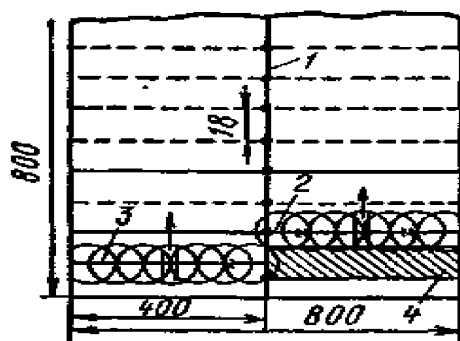
Рис. 5.3. Технологическая схема работы дождевальной машины “Волжанка”: 1 – за-крытый или разборный оросительный трубопровод; 2, 3 – первое и второе крылья; 4 – политая площадь (размеры в м).
