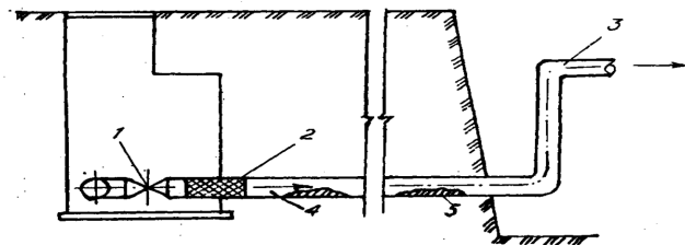
Рис. 7.8. Схема прочистки трубопровода поролоновым поршнем: 1 – задвижка, через которую вводится поршень; 2 – поролоновый поршень; 3 – выпуск; 4 – промываемый трубопровод; 5 – засорения.
