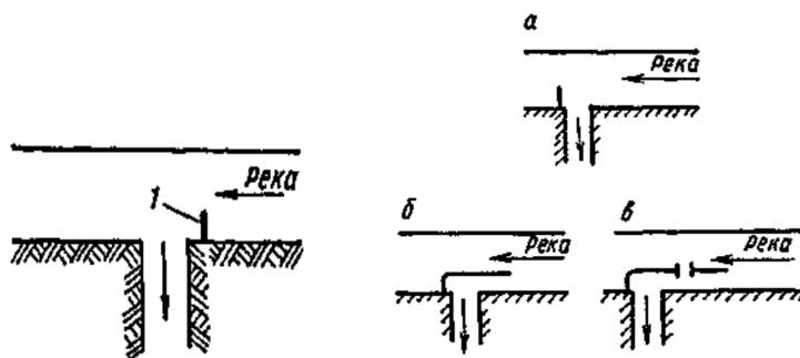
Рис. 5.12. Донный порог (1) перед головной частью магистрального канала.
