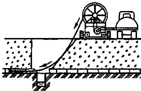
Рис. 4.18. Промывка дренажей и коллекторов от наносов дренажно-промывочной машиной (Д-910, ПДТ-125 и др.).
