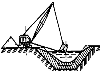
Рис. 4.14. Схема работы экскаватора при углублении и расширении русла водотока.
