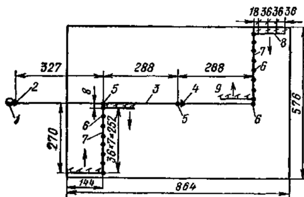
Рис. 5.9. Примерная схема при поливе установкой КИ-50 “Радуга”: 1 – насосная станция; 2, 4 – переходники 180×150; 3, 7 – магистральный и распределительный трубопроводы; 5, 6 – трубы-гидранты диаметром 150 и 125 мм; 8, 9 – дождевальные крыло и аппарат (размеры в м).
