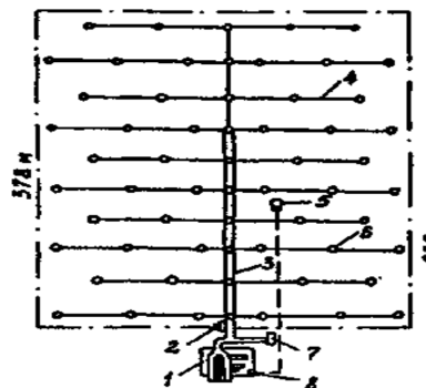
Рис. 5.11. Схема синхронного импульсного дождевания: 1 – насосная станция; 2 – гидроподкормщик; 3–4 – трубопроводная сеть; 5 – датчик; 6 – аппараты импульсного дождевания; 7 – генератор командных сигналов; 8 – пульт управления.
