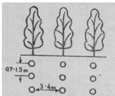
Рис. 11. Схема трёхрядной полезащитной полосы из одной главной породы:
